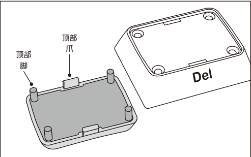
3. 抓住底部,用力压入专用拔键器,即可拆下顶部(字仁)。
