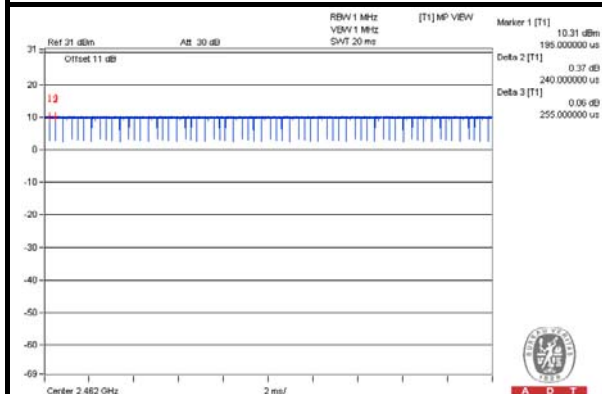
802.11n (20MHz)
