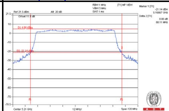
802.11ac (80MHz)
