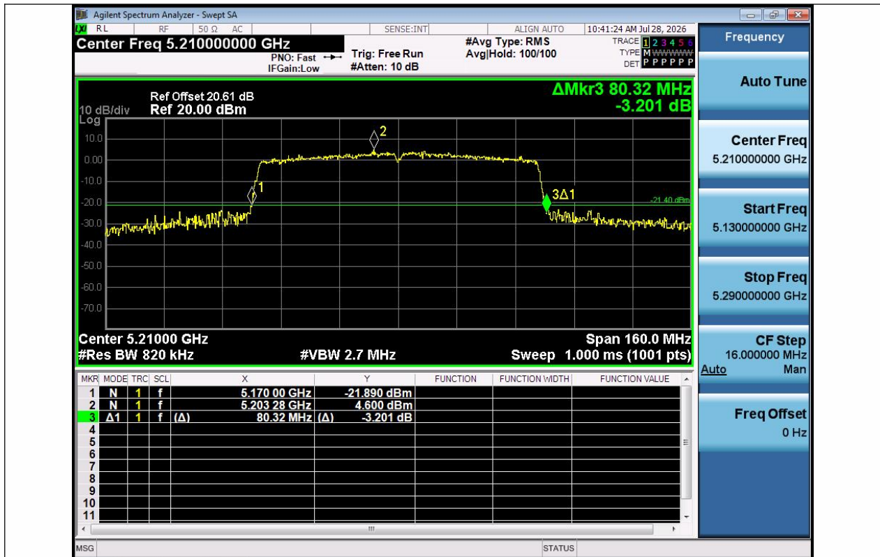
11AC80SISO-Ant1-5210
