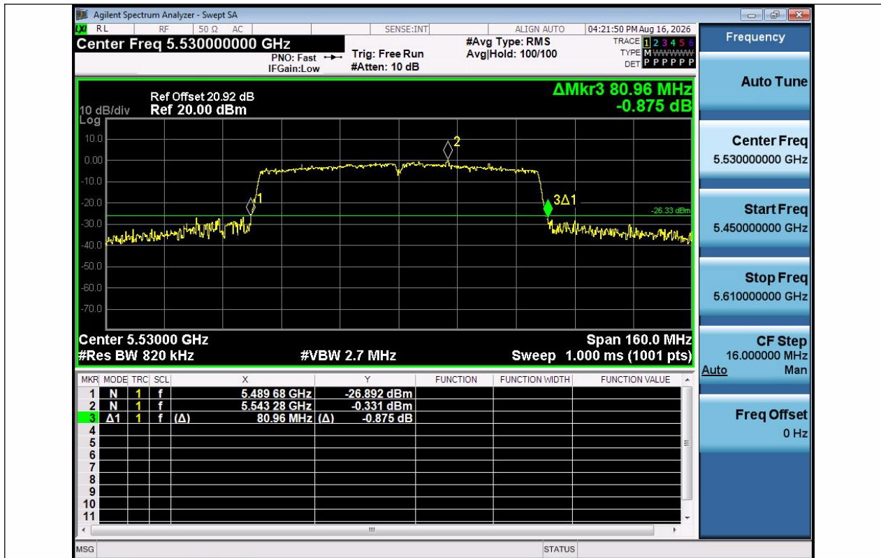
11AC80SISO-Ant1-5530
