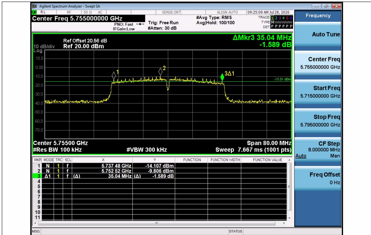
11N40SISO-Ant1-5755-PASS
