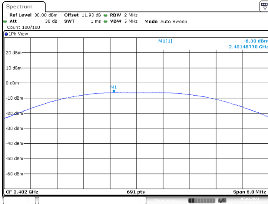
BLE_2M_Ant1_2402
