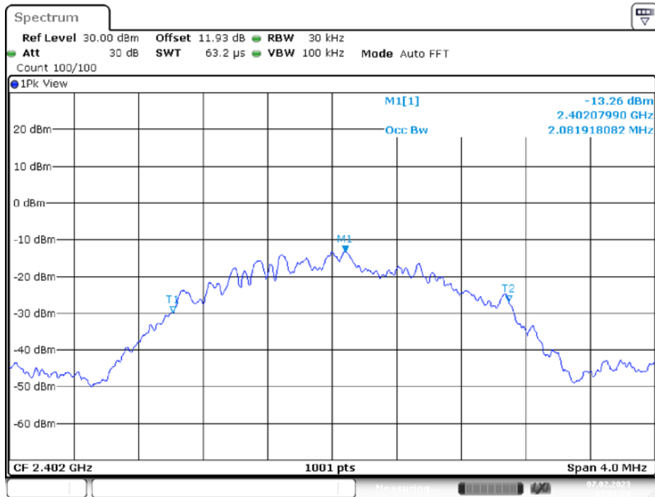
BLE_2M_Ant1_2402
