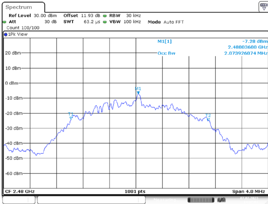
BLE_2M_Ant1_2480
