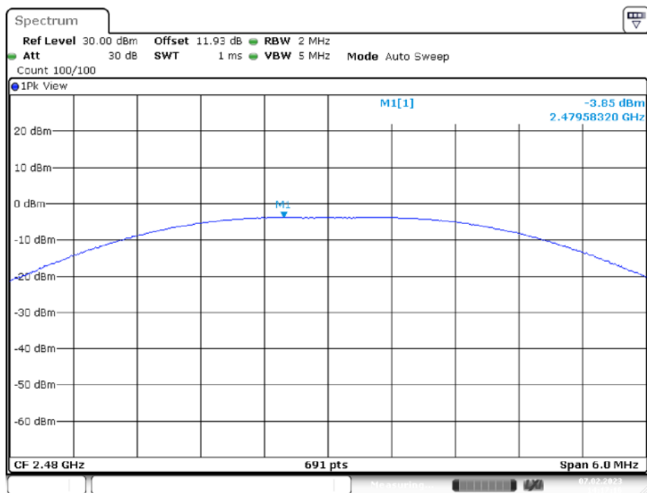
BLE_2M_Ant1_2480
