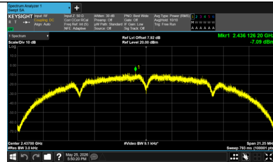
IEEE 802.11b_Channel 6_20MHz_Antenna 0
