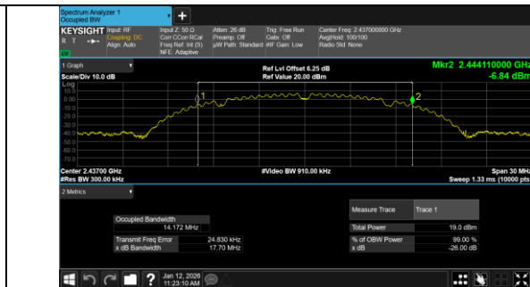
IEEE 802.11b_Channel 6_20MHz_Antenna 0
