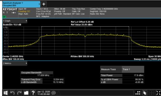
IEEE 802.11n_Channel 11_20MHz_Antenna 0
