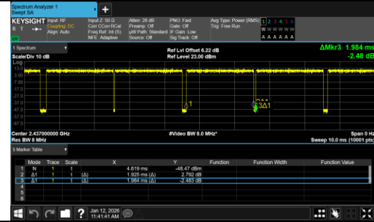
IEEE 802.11n_20MHz_Channel 6
