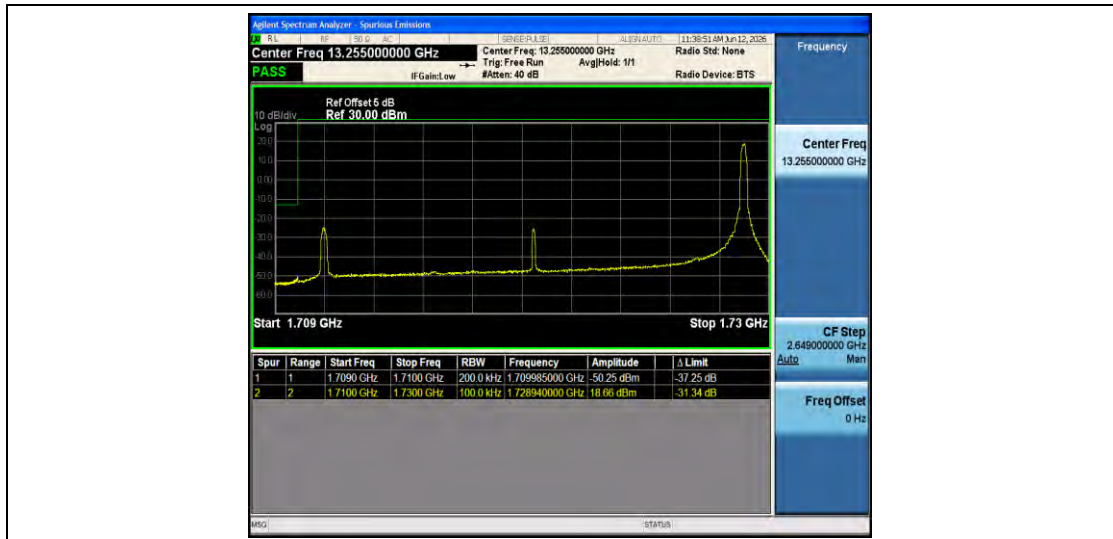
Band4-20MHz-16QAM-20050-1RB#99-PASS
