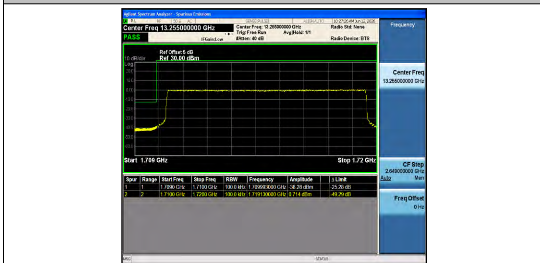
Band4-10MHz-QPSK-20000-50RB#0-PASS
