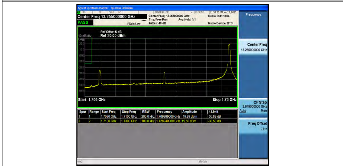
Band4-20MHz-QPSK-20050-1RB#99-PASS
