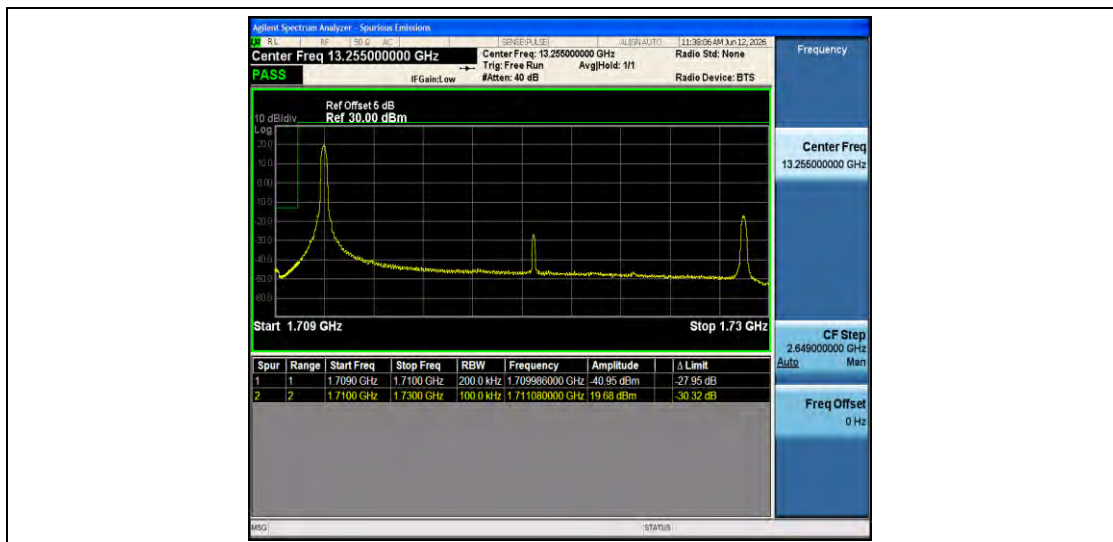
Band4-20MHz-QPSK-20050-1RB#0-PASS
