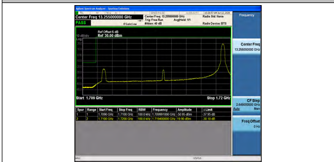
Band4-10MHz-QPSK-20000-1RB#49-PASS
