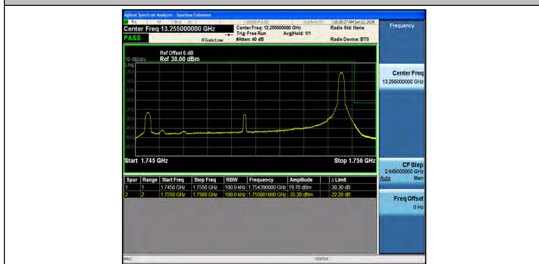
Band4-10MHz-QPSK-20350-1RB#49-PASS
