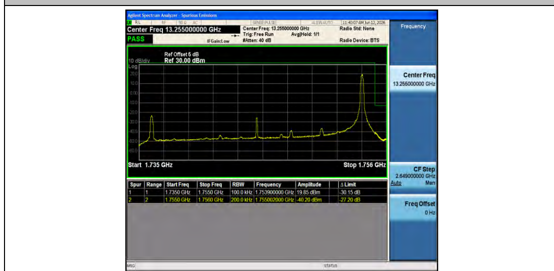
Band4-20MHz-QPSK-20300-1RB#99-PASS
