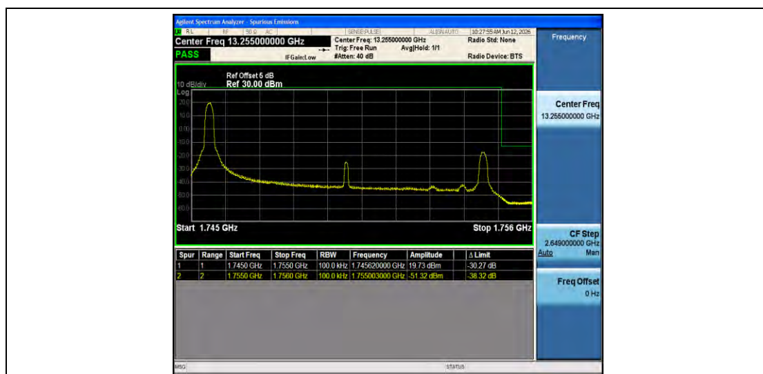
Band4-10MHz-QPSK-20350-1RB#0-PASS
