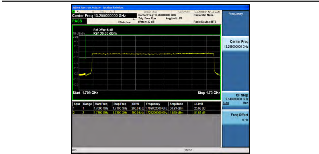
Band4-20MHz-QPSK-20050-100RB#0-PASS
