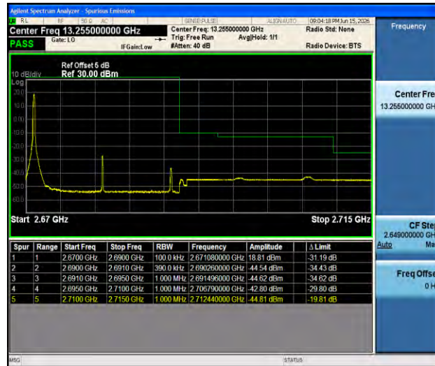
Band41-20MHz-QPSK-41490-1RB#0-PASS
