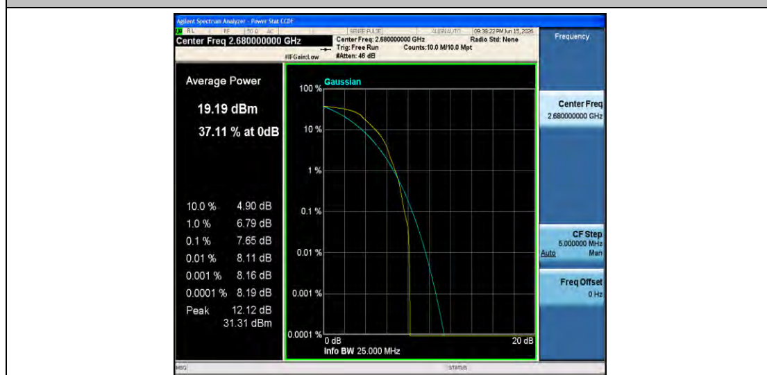
Band41-20MHz-QPSK-41490-1RB#0-PASS
