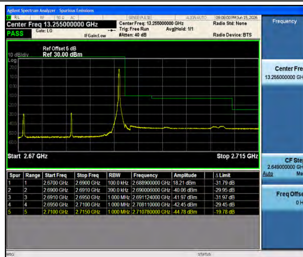
Band41-20MHz-QPSK-41490-1RB#99-PASS
