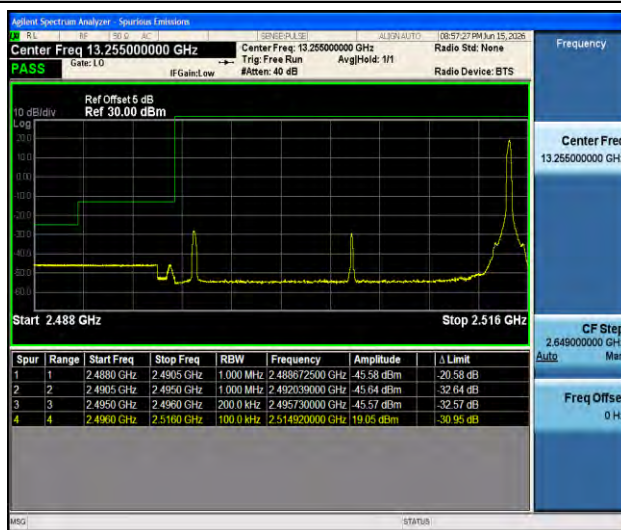
Band41-20MHz-QPSK-39750-1RB#99-PASS
