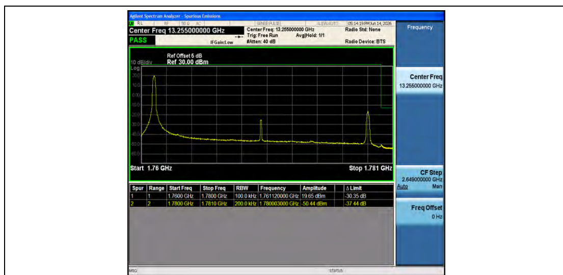
Band66-20MHz-QPSK-132572-1RB#0-PASS
