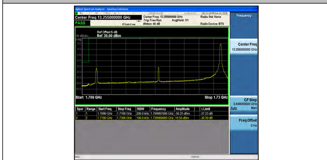
Band66-20MHz-QPSK-132072-1RB#99-PASS
