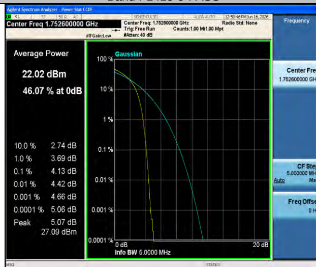
Band4-1513-5-PASS
