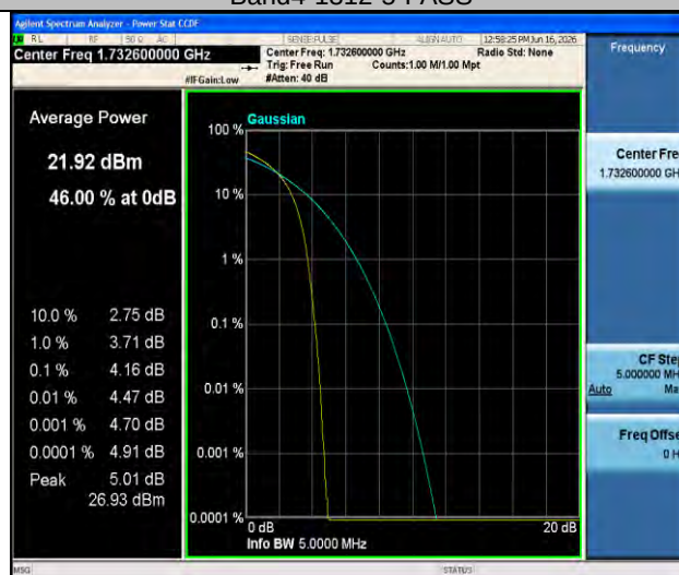
Band4-1413-5-PASS
