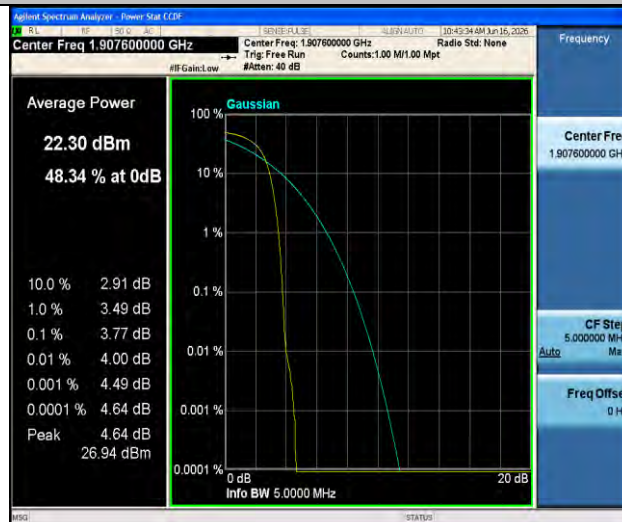
Band2-9538-3-PASS
