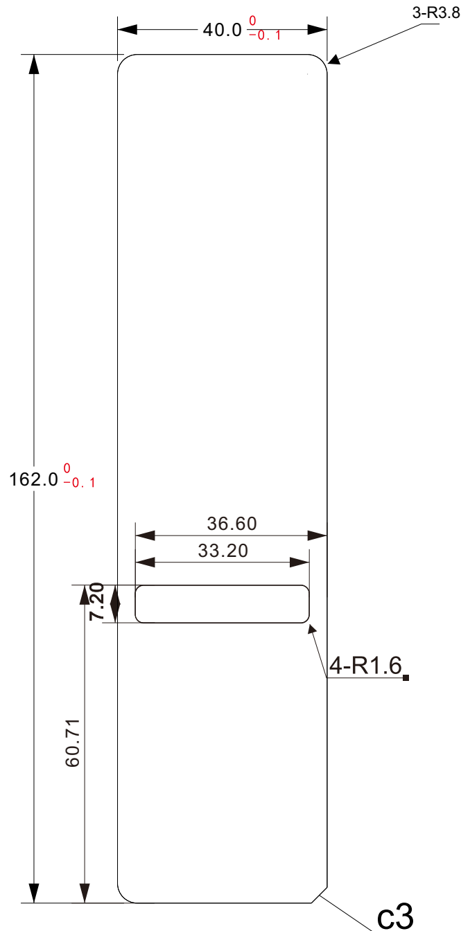
(尺寸图)
