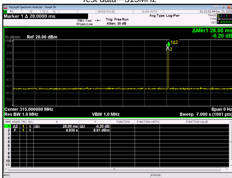
Test data—315MHz
