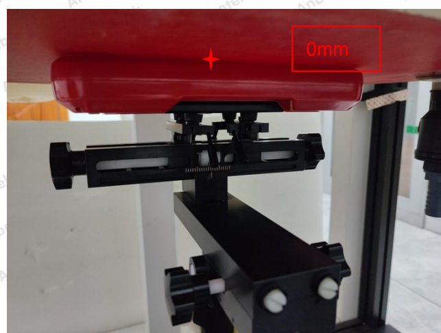
Front(0mm)
