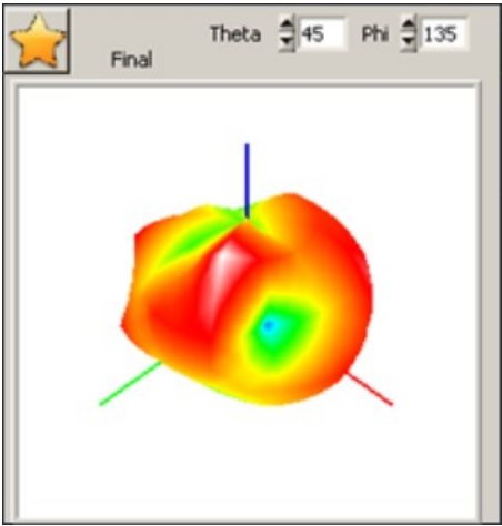
5500MHZ
