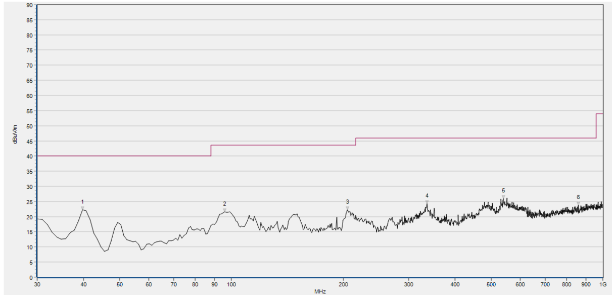
(Plot A: 30MHz – 1GHz, Test Antenna Vertical)
