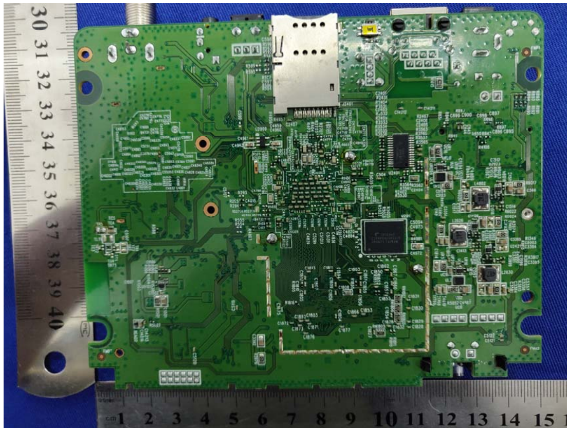
Wi-Fi Module
