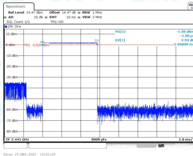
DH5_Hop
