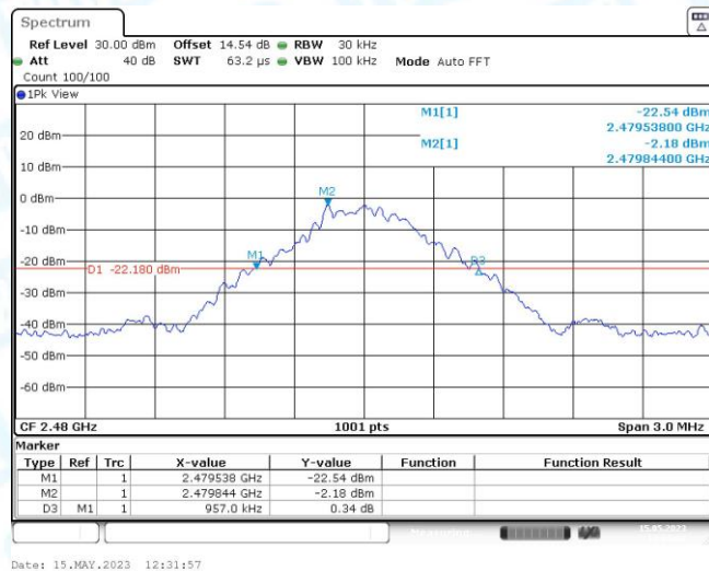
DH5_2480
