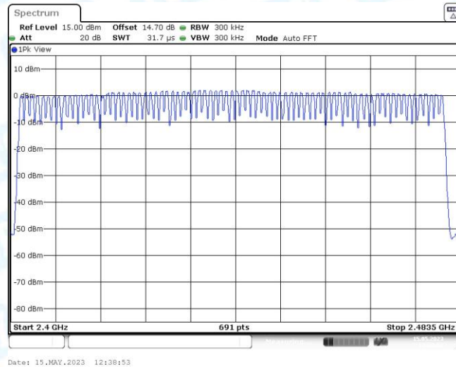
DH5_Hop
