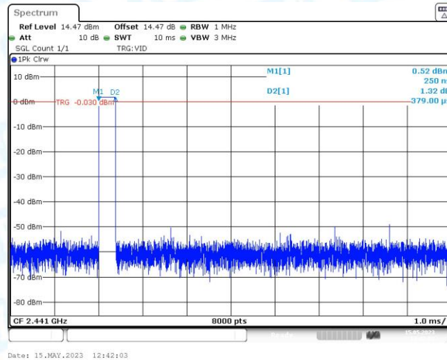
DH1_Hop
