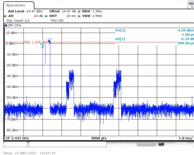
2DH1_Hop
