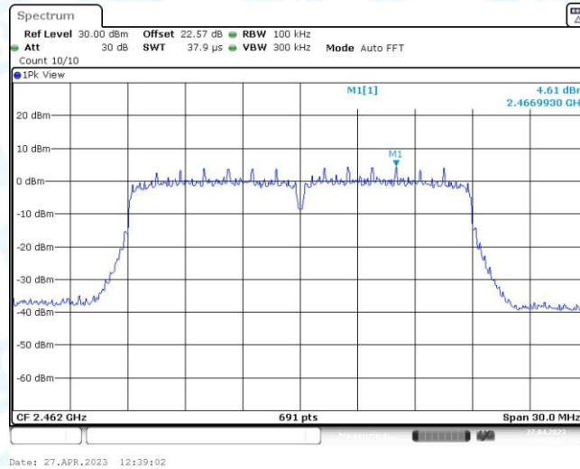
11N20MIMO_Ant2_2462_0~Reference
