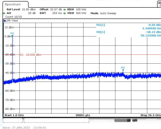
11N40MIMO_Ant2_2422_1000~26500
