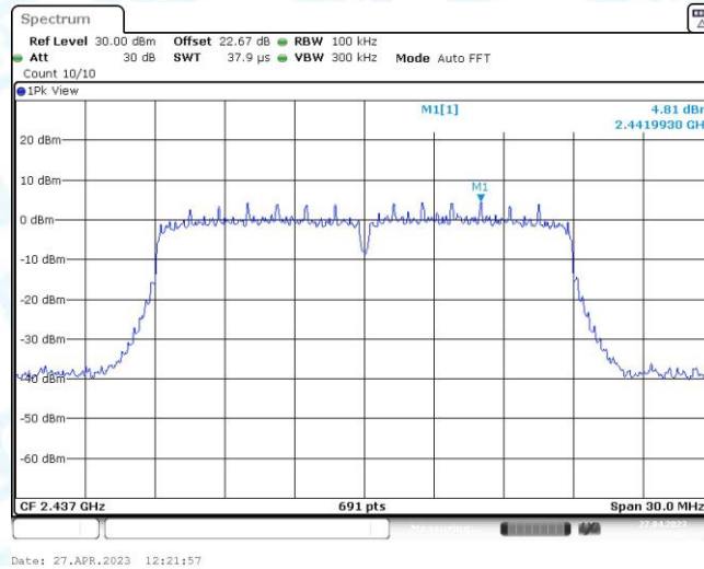
11N20MIMO_Ant2_2437_0~Reference
