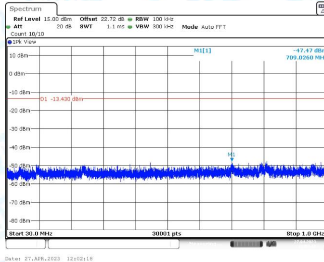
11G_Ant2_2412_30~1000
