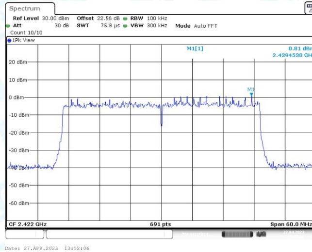
11AX40MIMO_Ant1_2422_0~Reference
