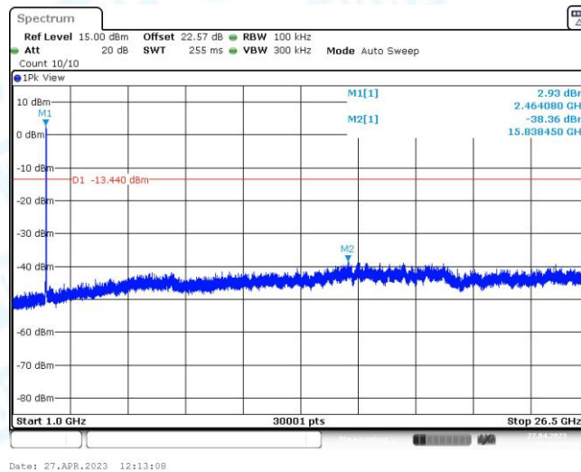
11G_Ant2_2462_1000~26500
