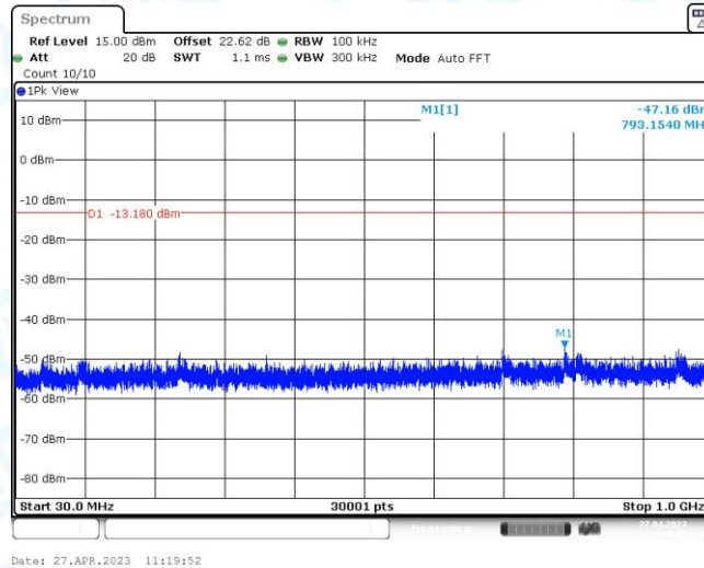
11G_Ant1_2412_30~1000
