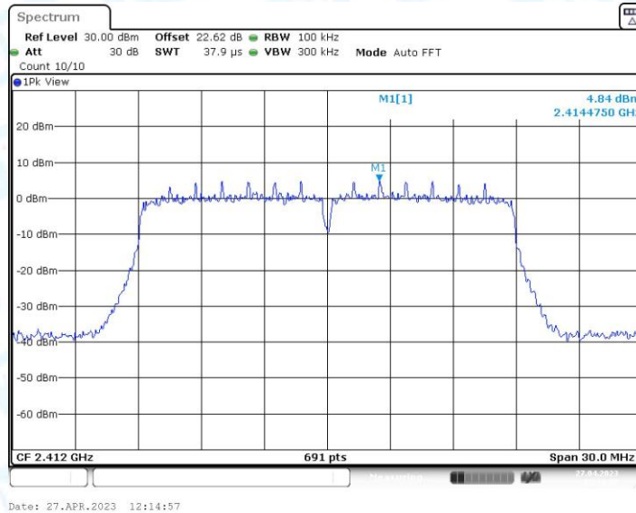
11N20MIMO_Ant1_2412_0~Reference
