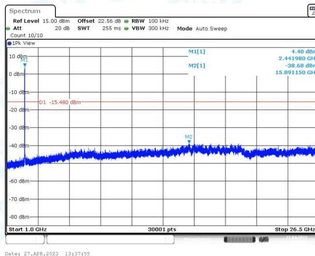
11AX20MIMO_Ant1_2437_1000~26500
