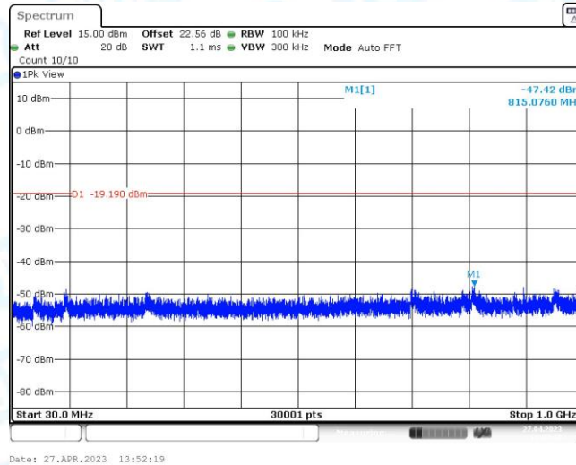
11AX40MIMO_Ant1_2422_30~1000
