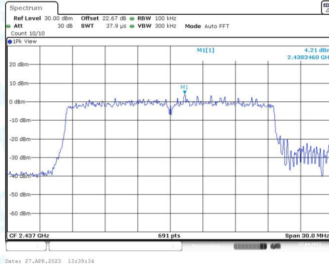
11AX20MIMO_Ant2_2437_0~Reference
