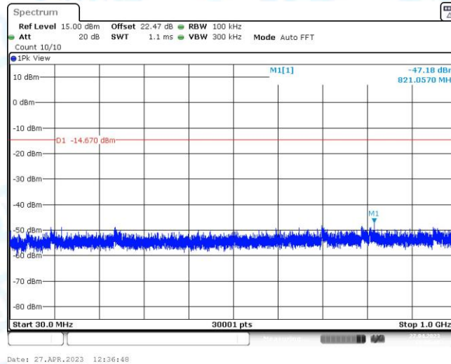
11N20MIMO_Ant1_2462_30~1000
