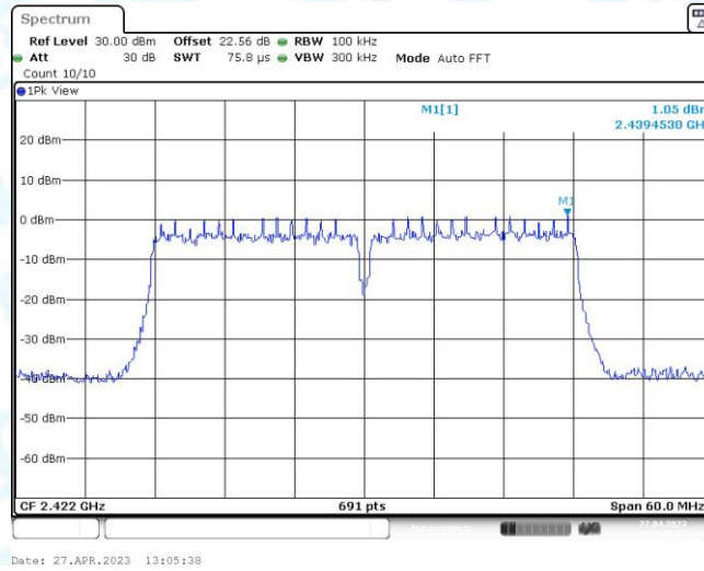
11N40MIMO_Ant1_2422_0~Reference
