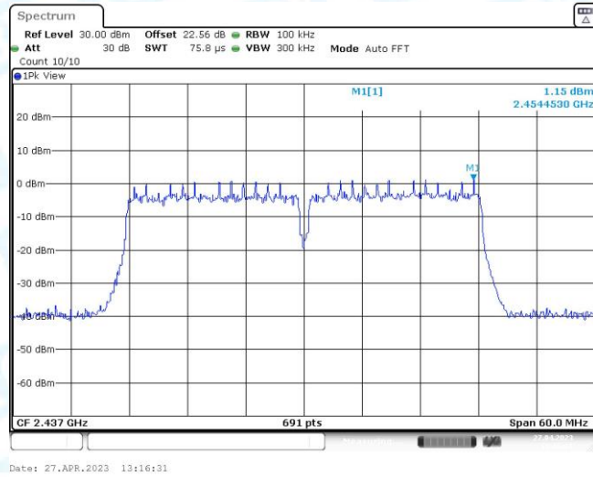
11N40MIMO_Ant1_2437_0~Reference
