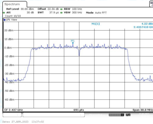
11AX20MIMO_Ant1_2437_0~Reference
