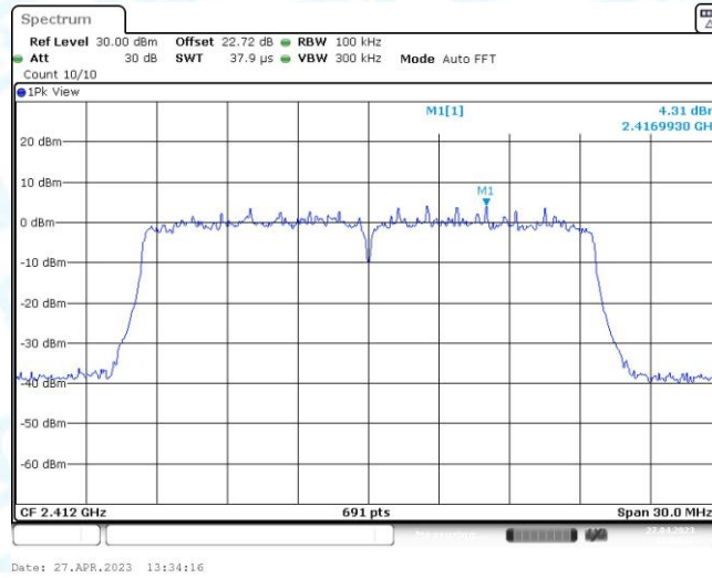
11AX20MIMO_Ant2_2412_0~Reference
