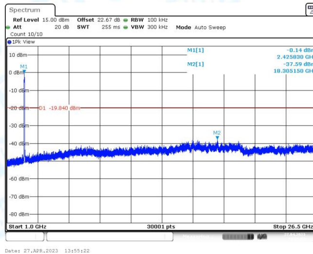
11AX40MIMO_Ant2_2422_1000~26500
