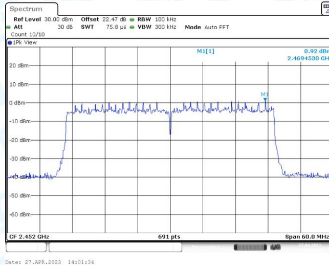
11AX40MIMO_Ant1_2452_0~Reference
