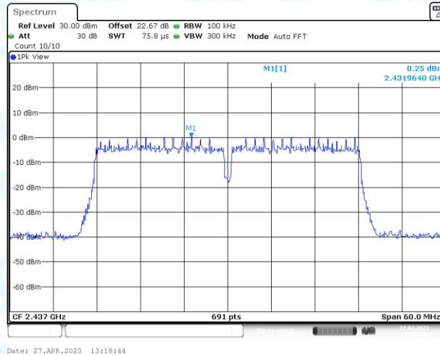
11N40MIMO_Ant2_2437_0~Reference
