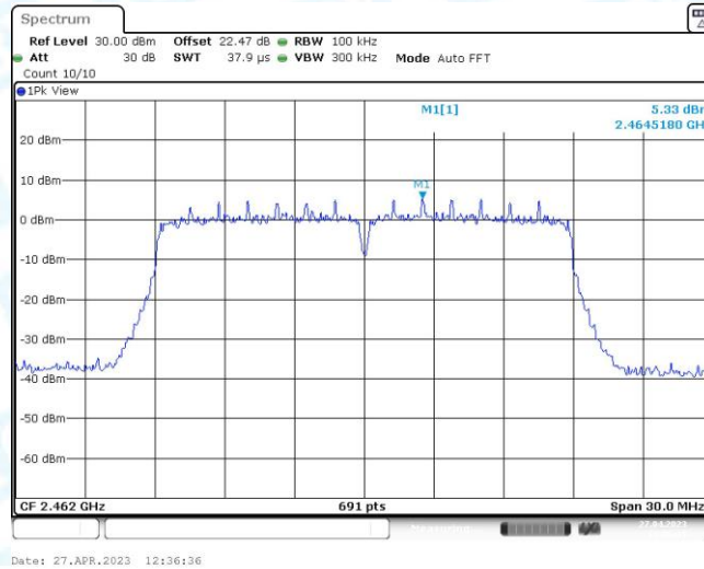
11N20MIMO_Ant1_2462_0~Reference
