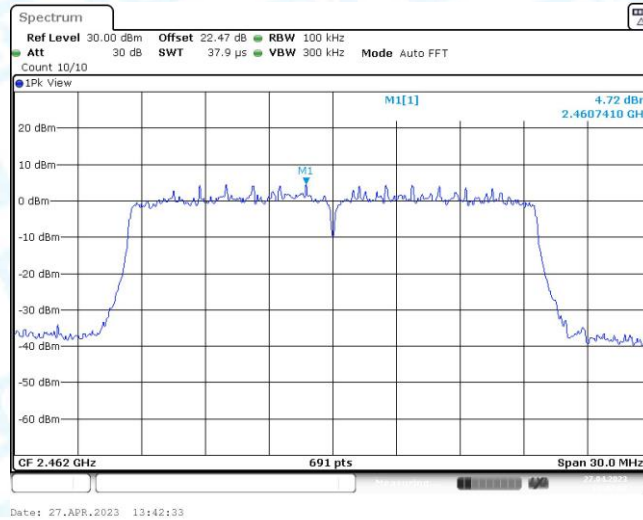
11AX20MIMO_Ant1_2462_0~Reference
