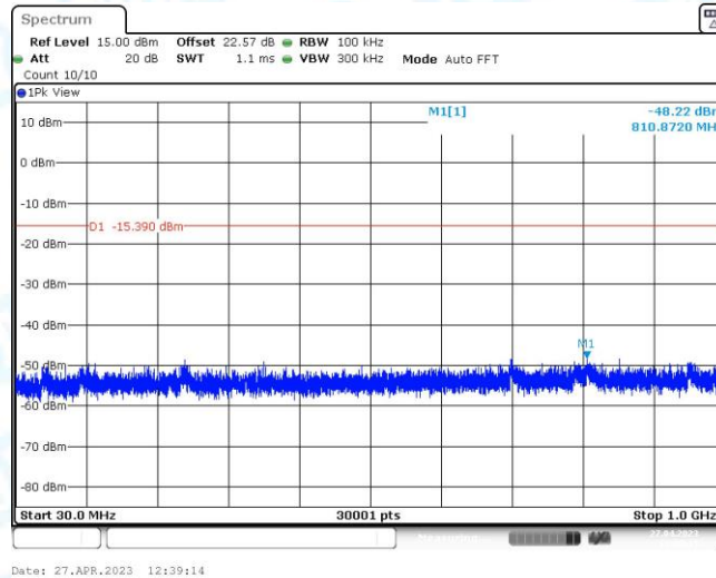
11N20MIMO_Ant2_2462_30~1000
