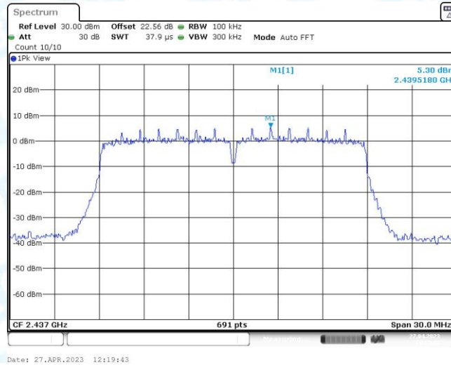
11N20MIMO_Ant1_2437_0~Reference
