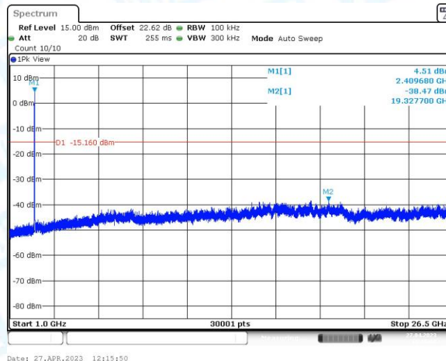
11N20MIMO_Ant1_2412_1000~26500
