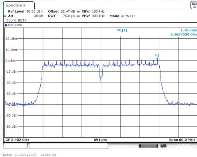
11N40MIMO_Ant1_2452_0~Reference
