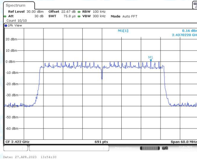
11AX40MIMO_Ant2_2422_0~Reference
