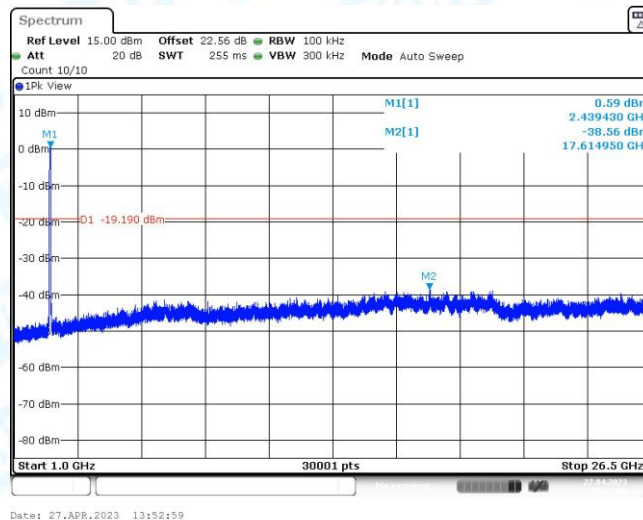
11AX40MIMO_Ant1_2422_1000~26500
