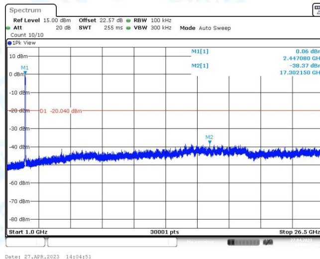
11AX40MIMO_Ant2_2452_1000~26500
