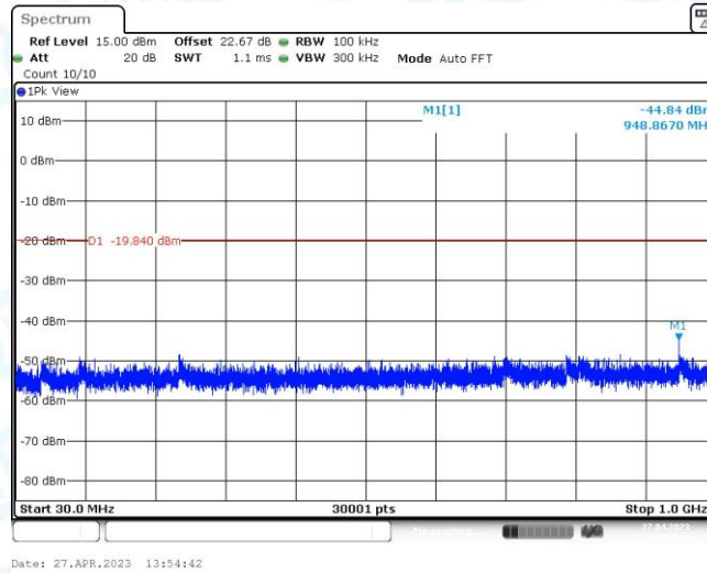
11AX40MIMO_Ant2_2422_30~1000
