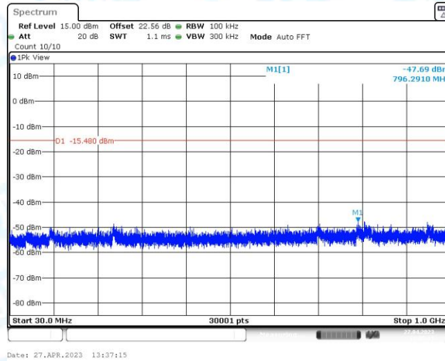
11AX20MIMO_Ant1_2437_30~1000
