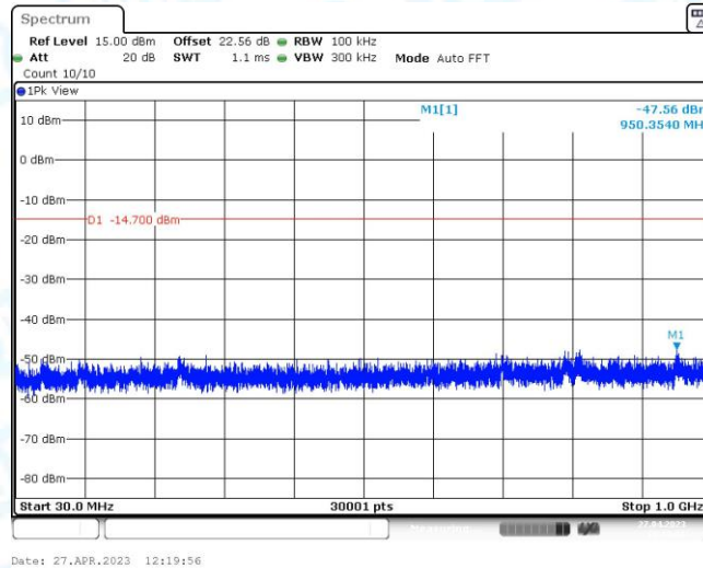
11N20MIMO_Ant1_2437_30~1000
