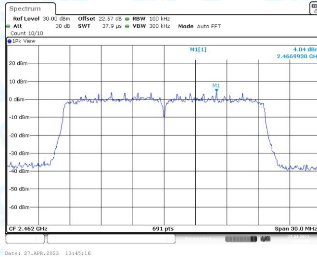
11AX20MIMO_Ant2_2462_0~Reference
