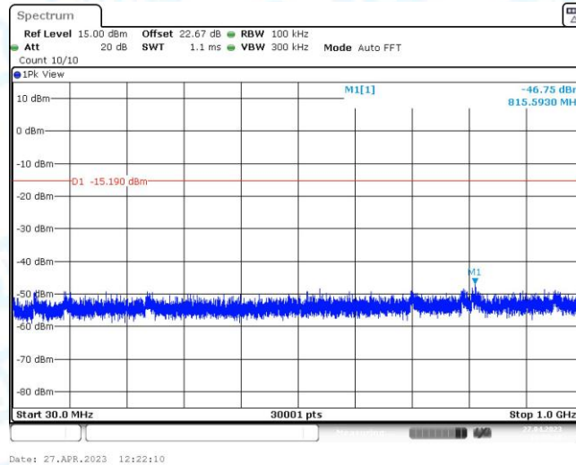
11N20MIMO_Ant2_2437_30~1000
