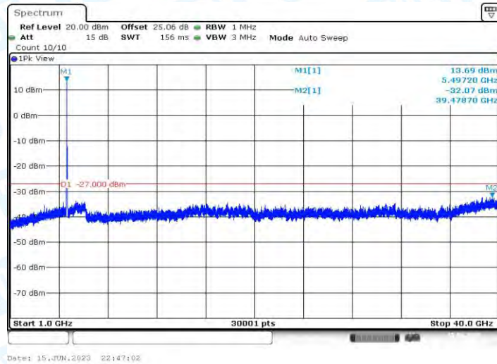
11AX20MIMO_Ant1_5500_1000~40000
