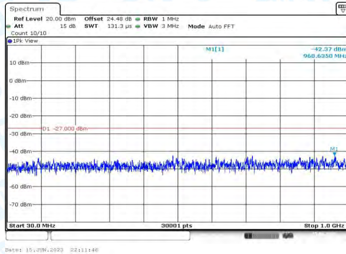
11AC40MIMO_Ant1_5190_30~1000
