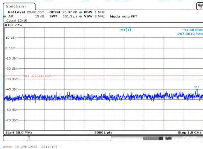
11AC20MIMO_Ant2_5825_30~1000
