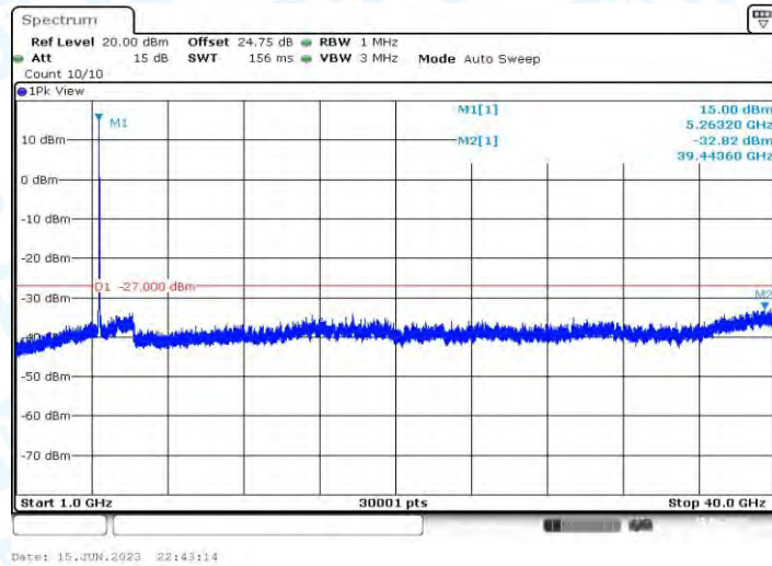
11AX20MIMO_Ant1_5260_1000~40000
