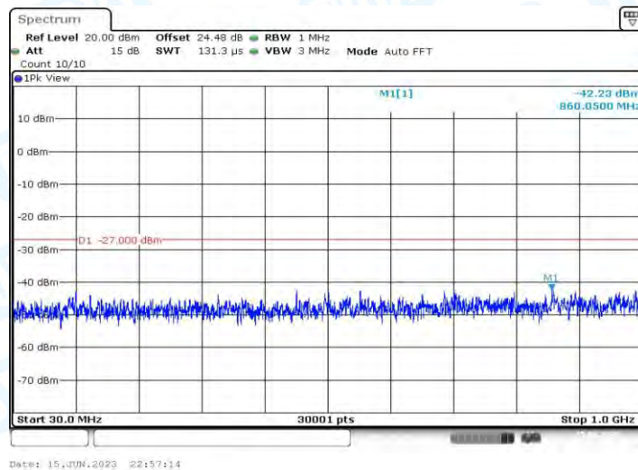
11AX40MIMO_Ant1_5190_30~1000
