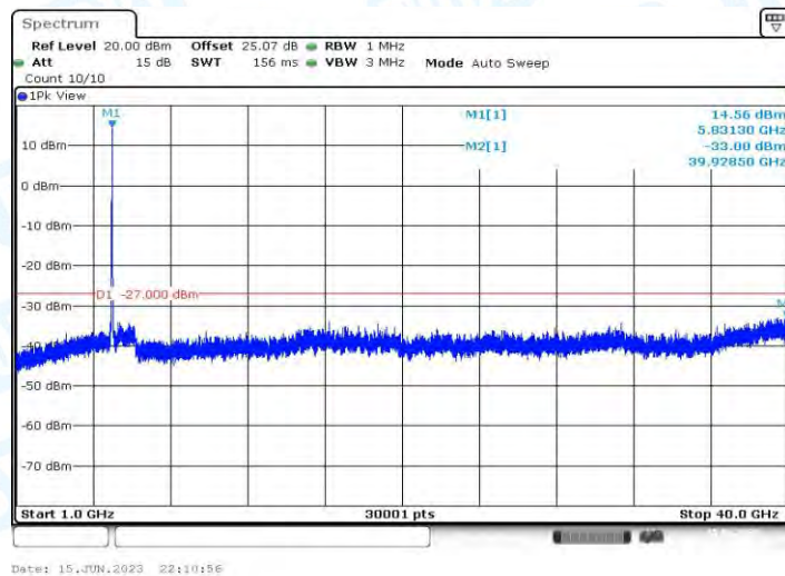
11AC20MIMO_Ant2_5825_1000~40000
