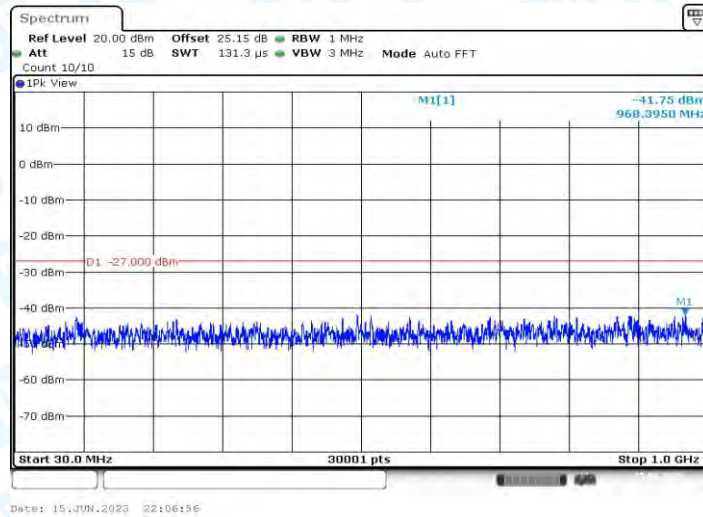
11AC20MIMO_Ant1_5745_30~1000
