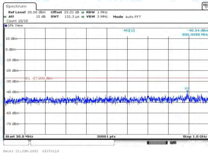
11AX20MIMO_Ant2_5785_30~1000
