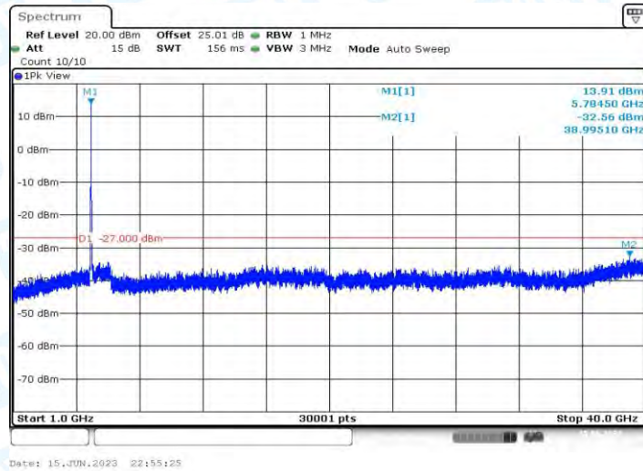
11AX20MIMO_Ant2_5785_1000~40000
