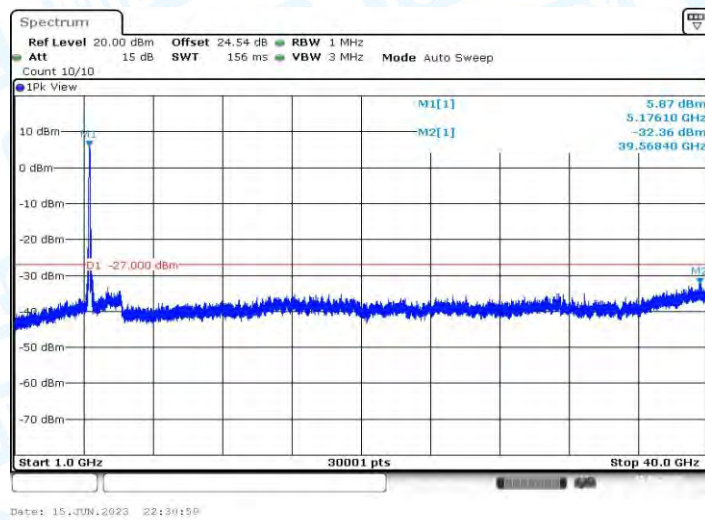
11AC80MIMO_Ant1_5210_1000~40000
