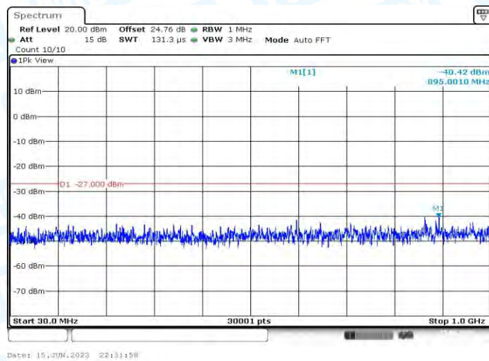
11AC80MIMO_Ant1_5290_30~1000
