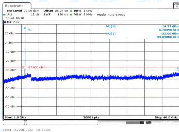
11AX20MIMO_Ant2_5700_1000~40000
