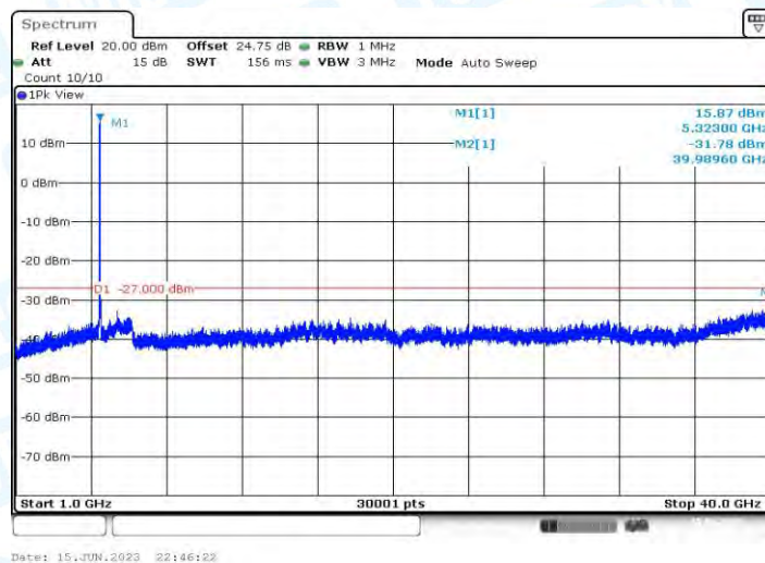
11AX20MIMO_Ant2_5320_1000~40000
