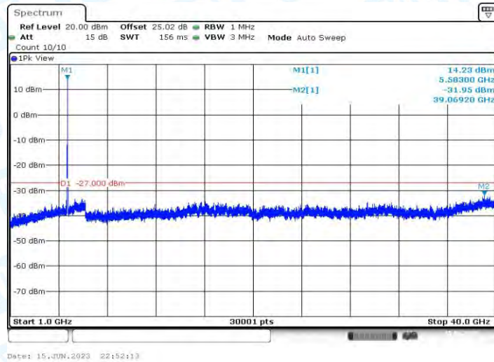
11AX20MIMO_Ant2_5580_1000~40000
