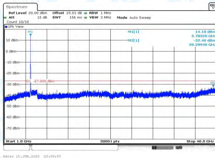
11AC20MIMO_Ant2_5785_1000~40000
