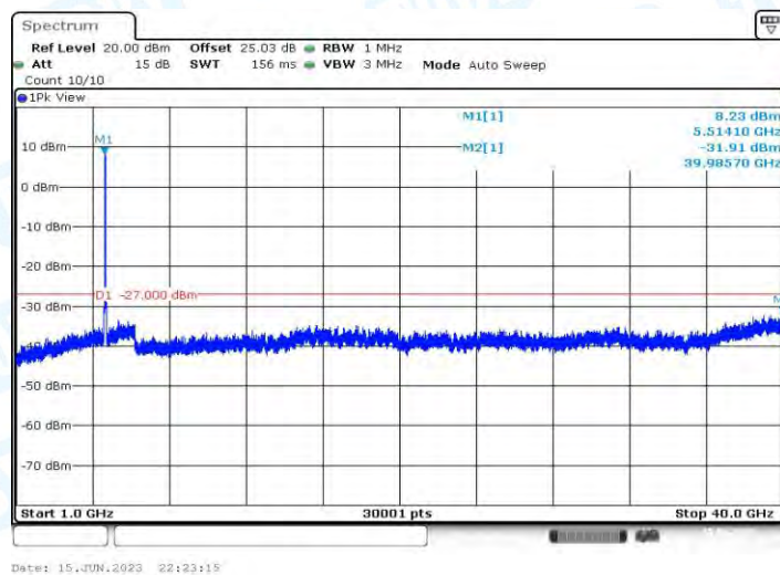
11AC40MIMO_Ant1_5510_1000~40000
