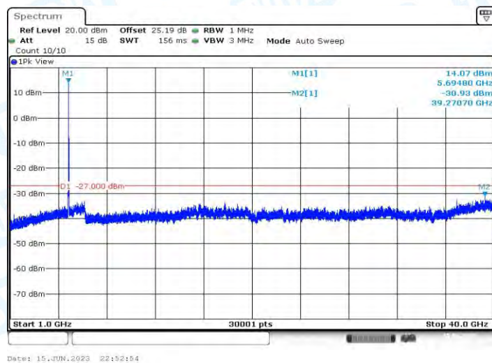
11AX20MIMO_Ant1_5700_1000~40000
