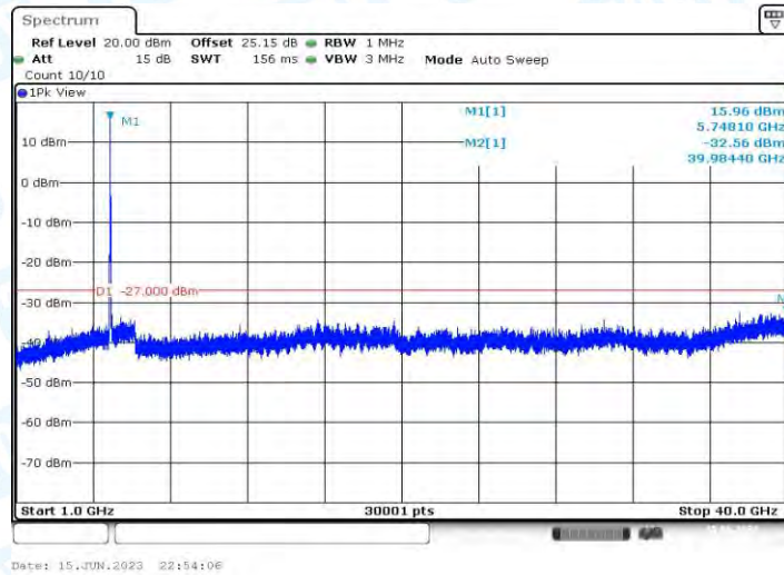
11AX20MIMO_Ant1_5745_1000~40000
