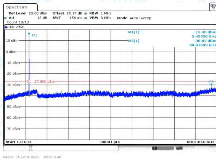
11AX20MIMO_Ant2_5500_1000~40000
