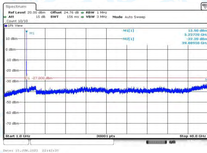
11AX20MIMO_Ant2_5240_1000~40000
