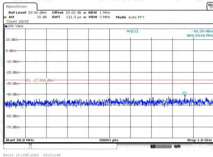
11AX20MIMO_Ant2_5580_30~1000
