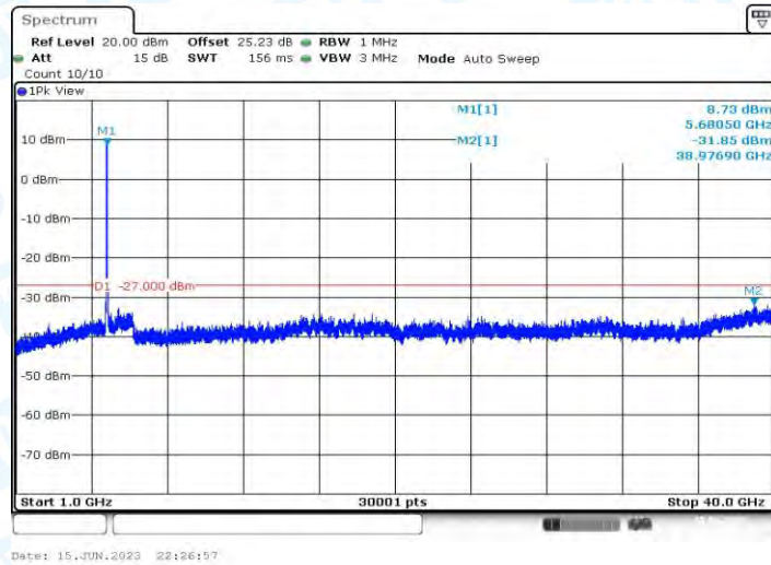
11AC40MIMO_Ant2_5670_1000~40000
