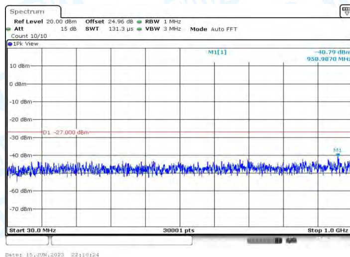
11AC20MIMO_Ant1_5825_30~1000
