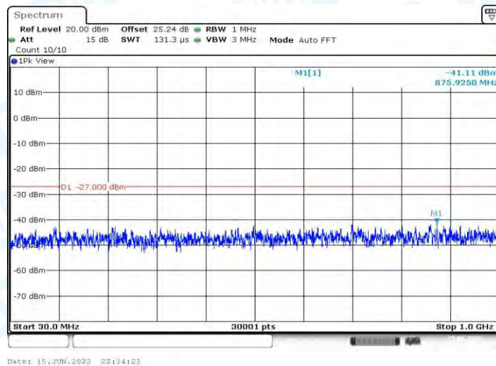
11AC80MIMO_Ant1_5530_30~1000
