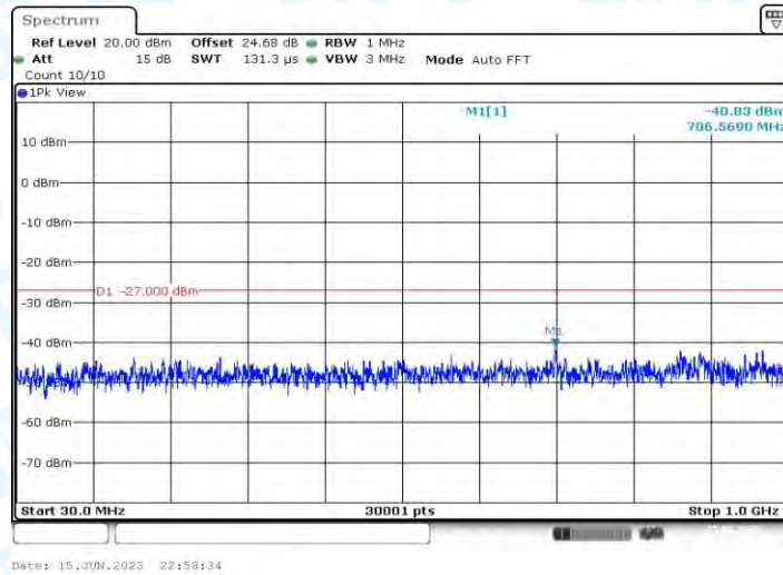
11AX40MIMO_Ant1_5230_30~1000
