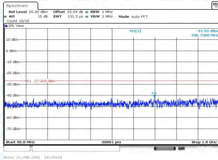
11AC80MIMO_Ant2_5775_30~1000
