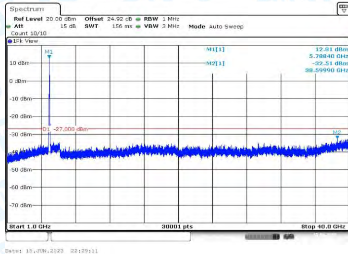
11AC40MIMO_Ant1_5795_1000~40000
