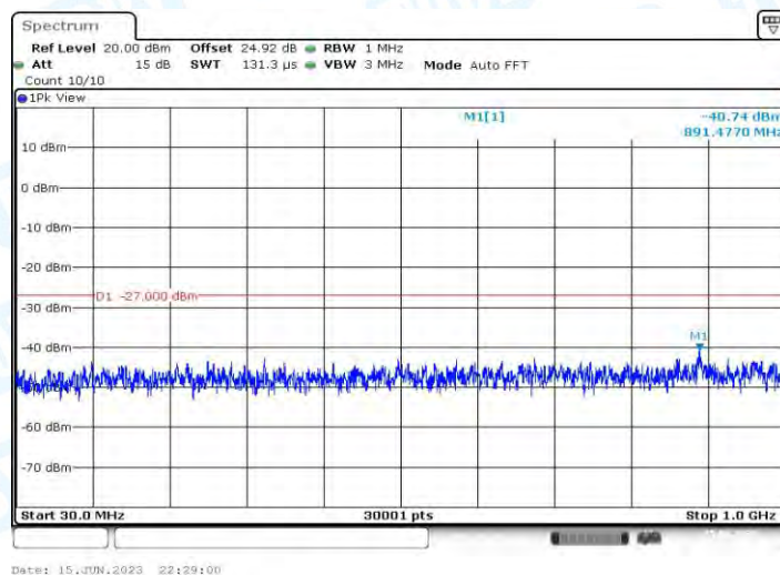
11AC40MIMO_Ant1_5795_30~1000
