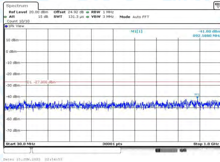
11AX20MIMO_Ant1_5785_30~1000
