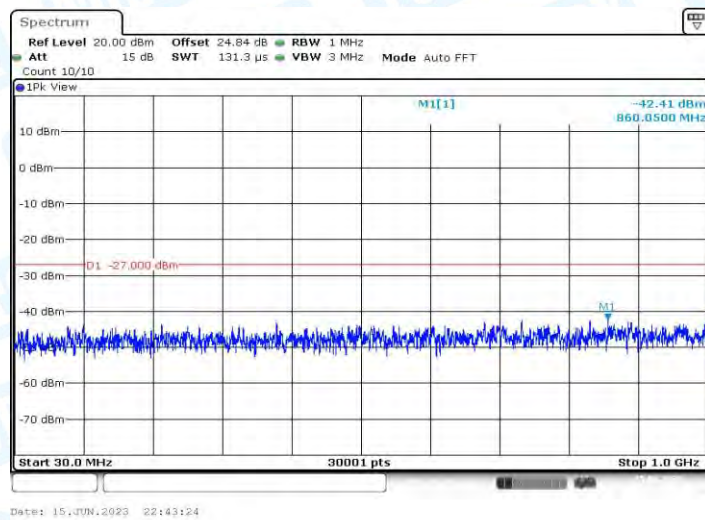
11AX20MIMO_Ant2_5260_30~1000
