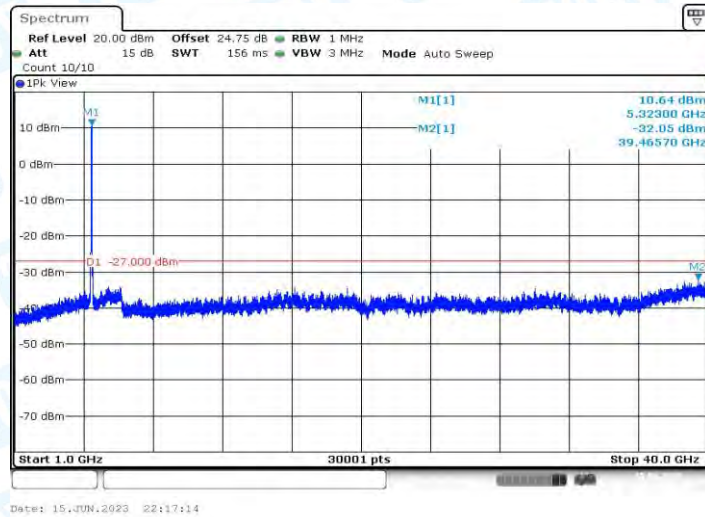
11AC40MIMO_Ant2_5310_1000~40000
