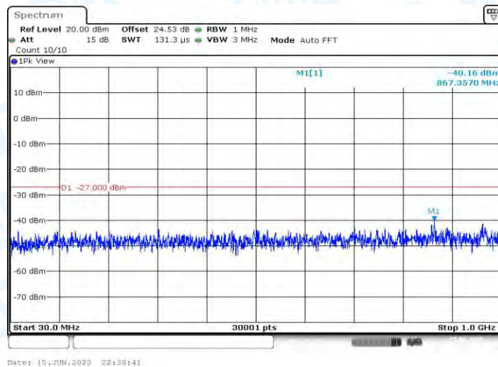
11AX20MIMO_Ant1_5180_30~1000
