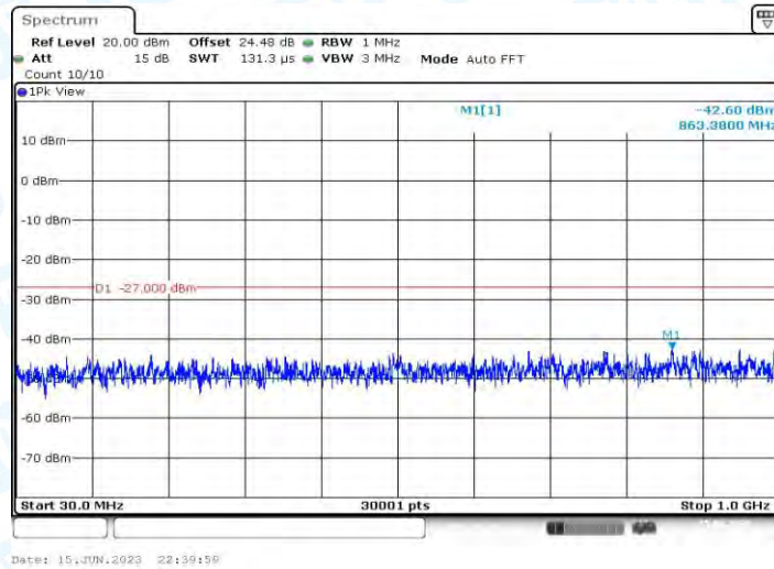
11AX20MIMO_Ant1_5200_30~1000
