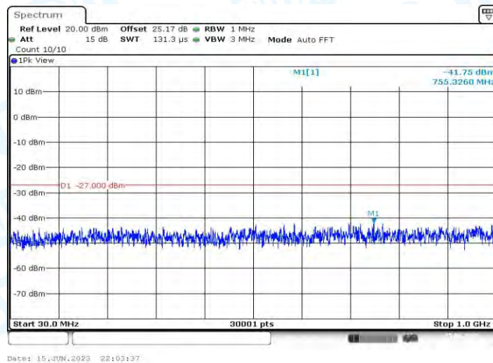
11AC20MIMO_Ant2_5500_30~1000
