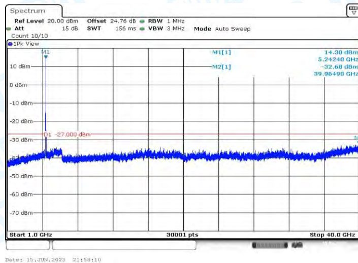
11AC20MIMO_Ant2_5240_1000~40000
