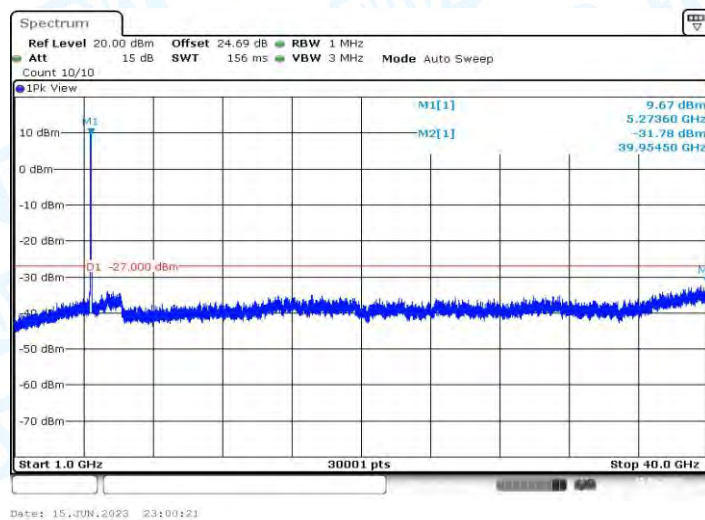
11AX40MIMO_Ant1_5270_1000~40000
