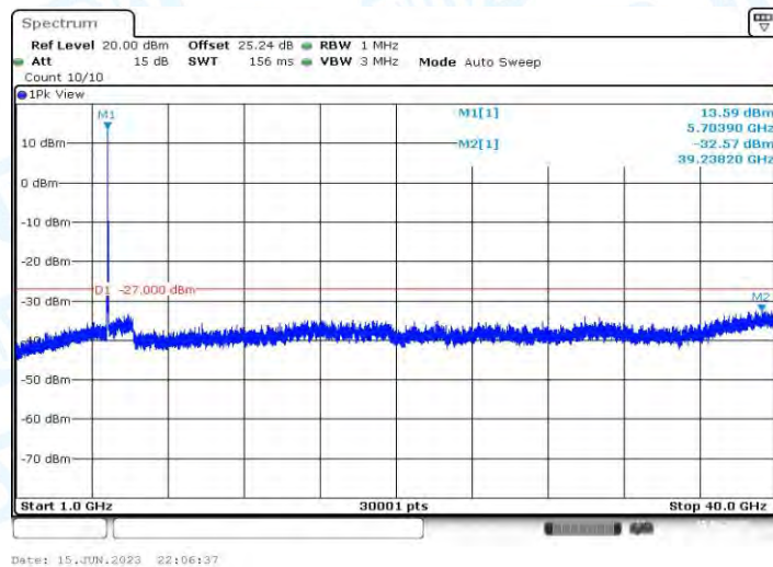
11AC20MIMO_Ant2_5700_1000~40000
