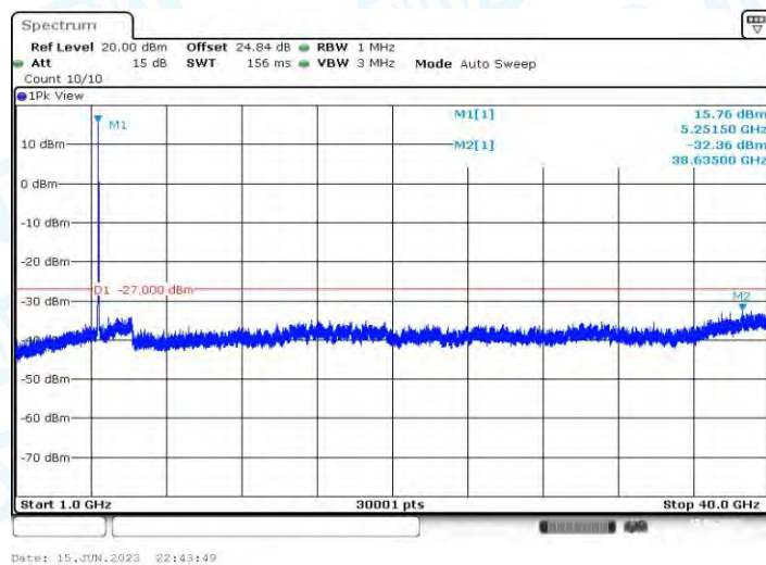
11AX20MIMO_Ant2_5260_1000~40000
