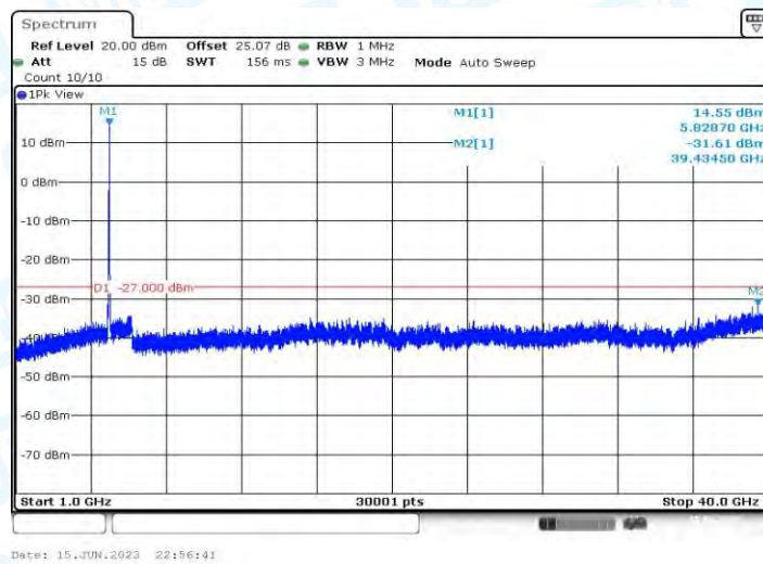
11AX20MIMO_Ant2_5825_1000~40000
