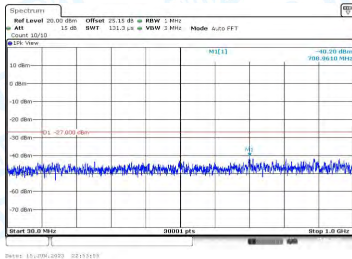
11AX20MIMO_Ant1_5745_30~1000
