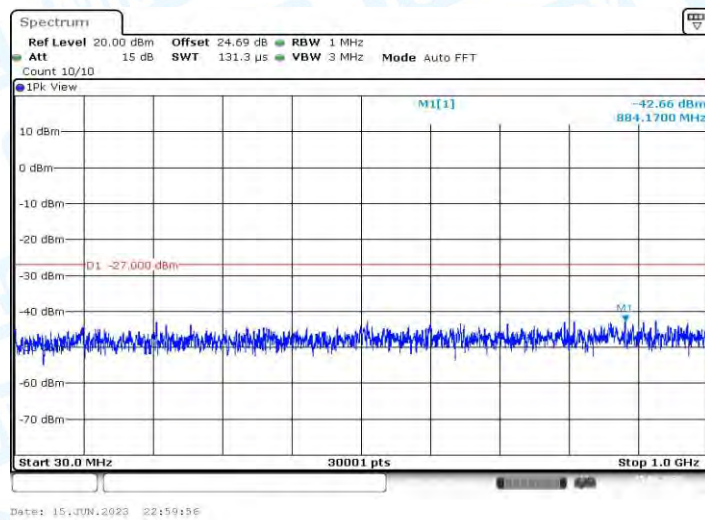
11AX40MIMO_Ant1_5270_30~1000
