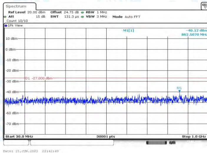
11AX20MIMO_Ant1_5260_30~1000
