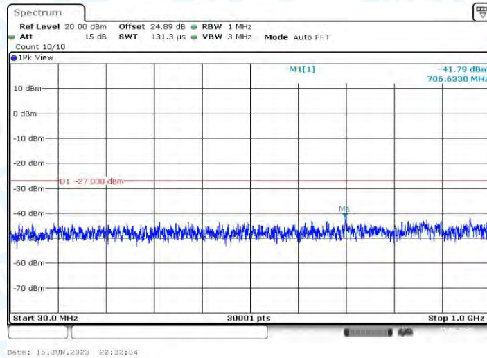
11AC80MIMO_Ant2_5290_30~1000
