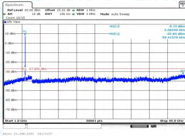
11AC40MIMO_Ant1_5550_1000~40000
