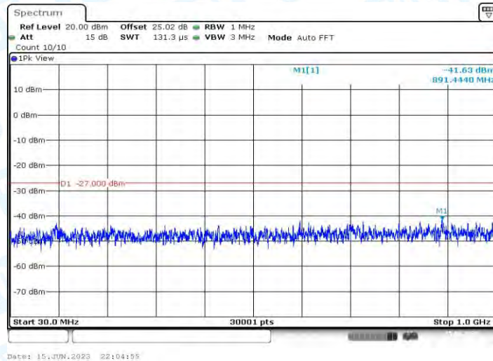
11AC20MIMO_Ant2_5580_30~1000
