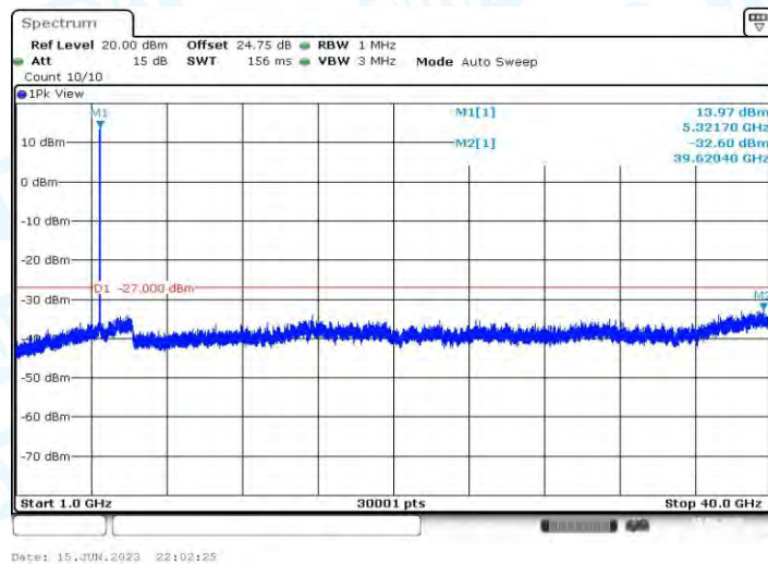
11AC20MIMO_Ant2_5320_1000~40000
