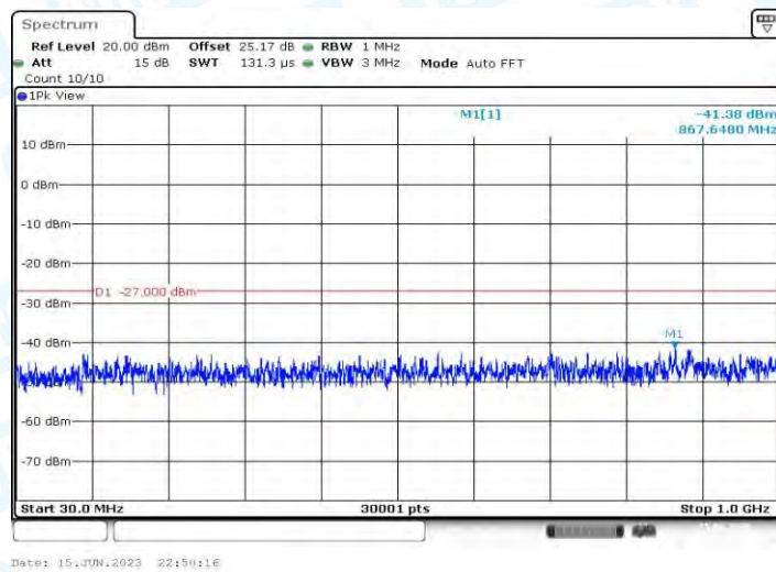
11AX20MIMO_Ant2_5500_30~1000
