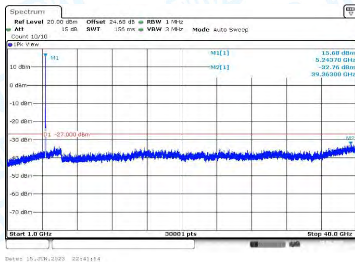
11AX20MIMO_Ant1_5240_1000~40000
