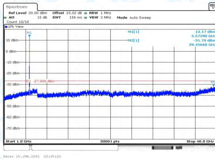
11AC20MIMO_Ant2_5580_1000~40000
