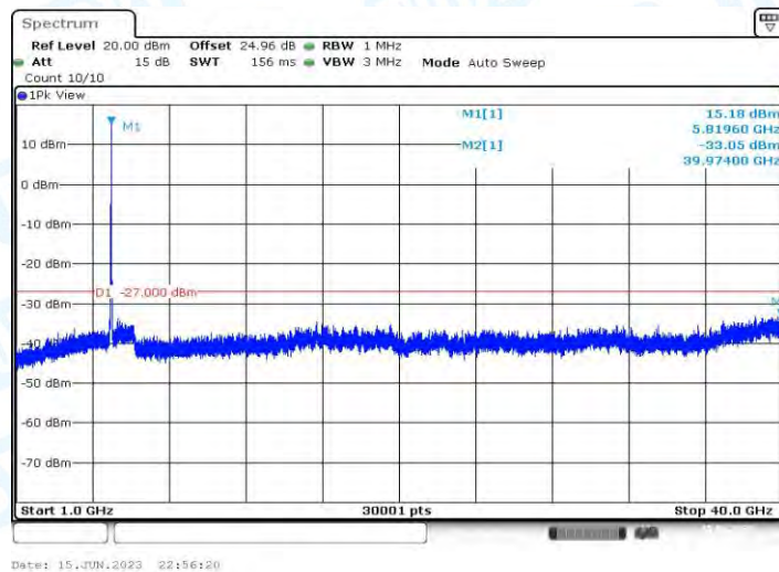
11AX20MIMO_Ant1_5825_1000~40000
