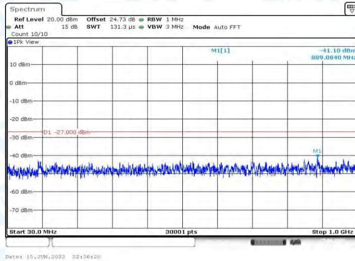
11AC80MIMO_Ant1_5610_30~1000
