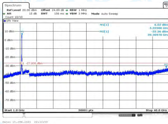
11AC80MIMO_Ant2_5290_1000~40000
