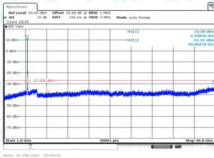
11AX40MIMO_Ant1_5230_1000~40000
