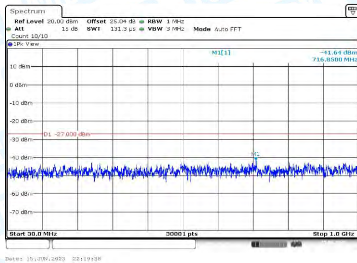
11AC40MIMO_Ant2_5550_30~1000
