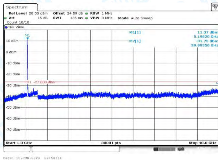
11AX40MIMO_Ant2_5190_1000~40000
