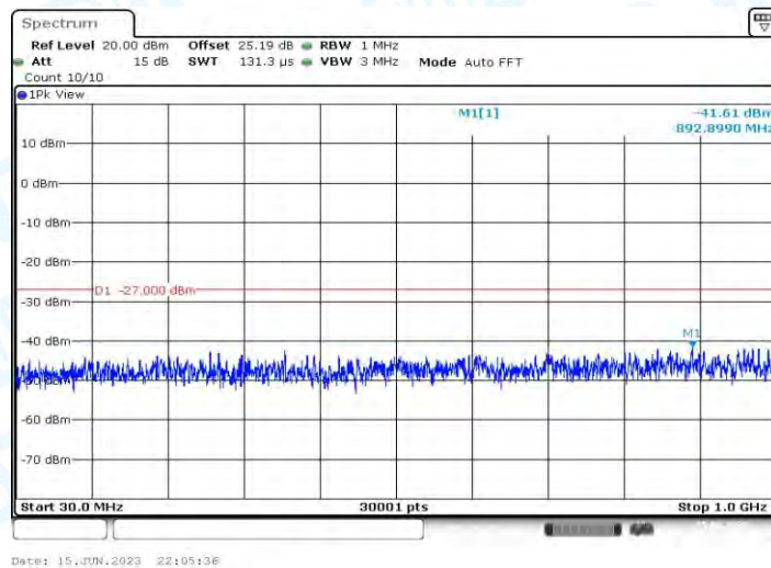
11AC20MIMO_Ant1_5700_30~1000
