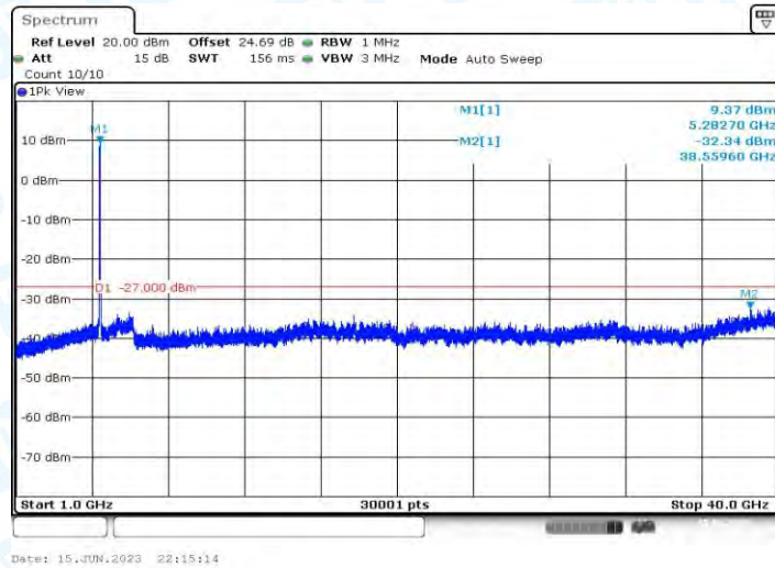
11AC40MIMO_Ant1_5270_1000~40000
