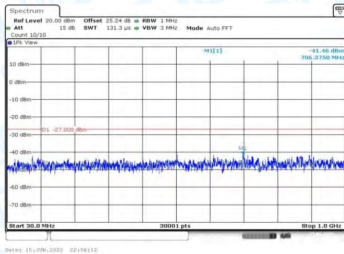
11AC20MIMO_Ant2_5700_30~1000
