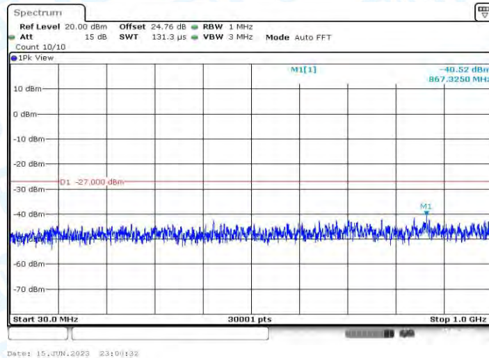
11AX40MIMO_Ant2_5270_30~1000
