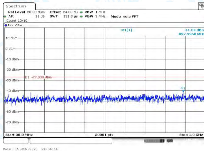
11AC80MIMO_Ant2_5610_30~1000
