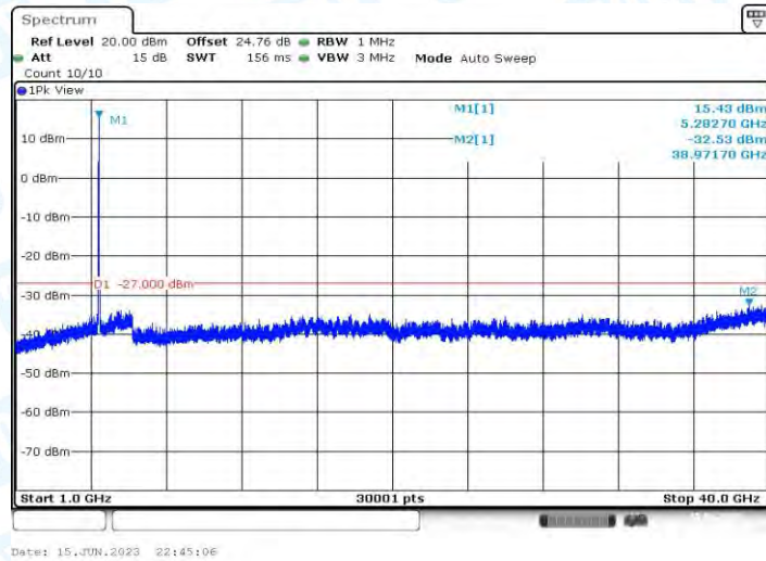
11AX20MIMO_Ant2_5280_1000~40000
