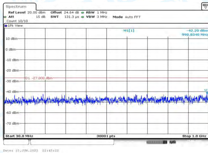
11AX20MIMO_Ant1_5320_30~1000
