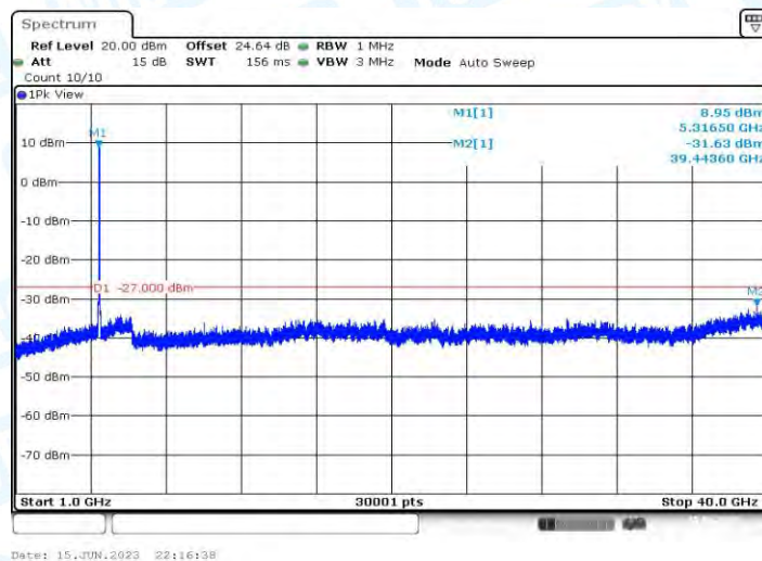
11AC40MIMO_Ant1_5310_1000~40000
