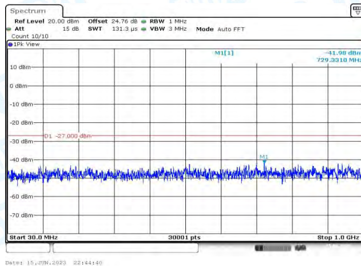
11AX20MIMO_Ant2_5280_30~1000
