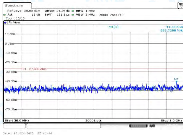
11AX20MIMO_Ant2_5200_30~1000
