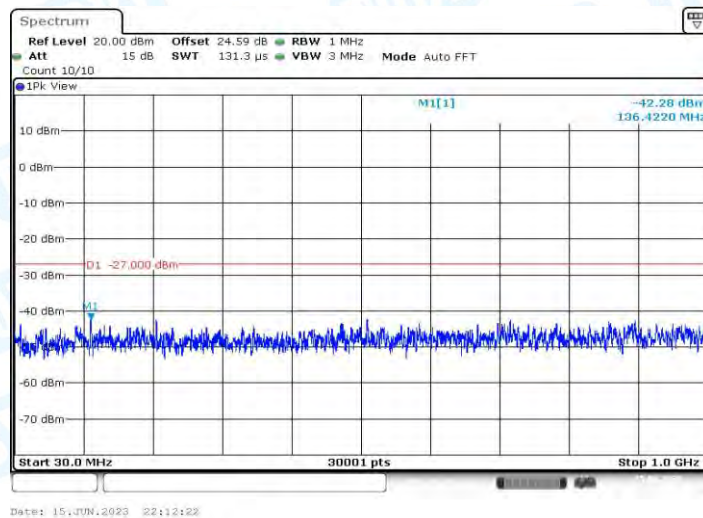
11AC40MIMO_Ant2_5190_30~1000
