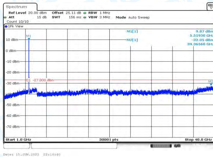
11AC40MIMO_Ant2_5510_1000~40000
