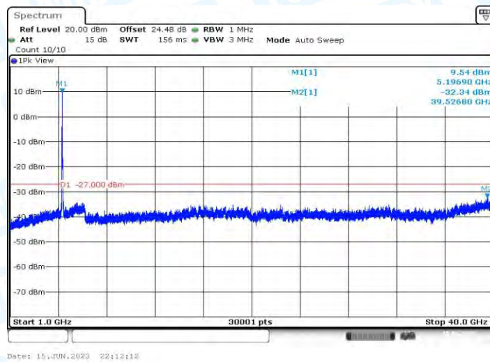
11AC40MIMO_Ant1_5190_1000~40000
