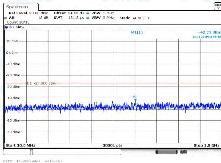
11AC80MIMO_Ant2_5210_30~1000
