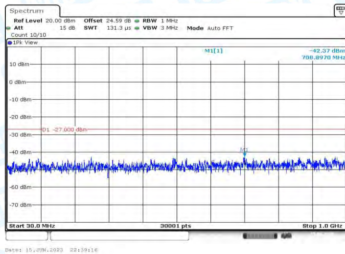
11AX20MIMO_Ant2_5180_30~1000
