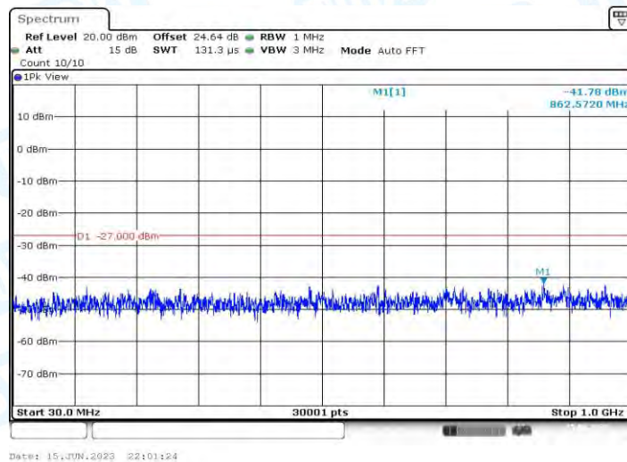
11AC20MIMO_Ant1_5320_30~1000
