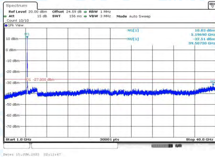
11AC40MIMO_Ant2_5190_1000~40000
