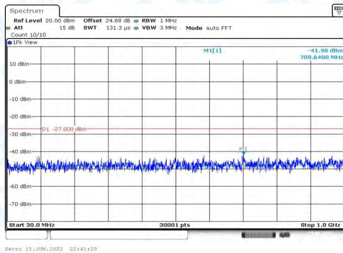
11AX20MIMO_Ant1_5240_30~1000
