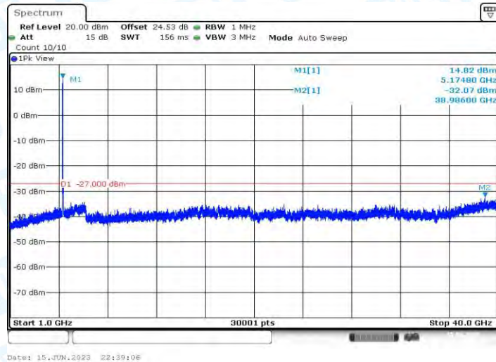
11AX20MIMO_Ant1_5180_1000~40000
