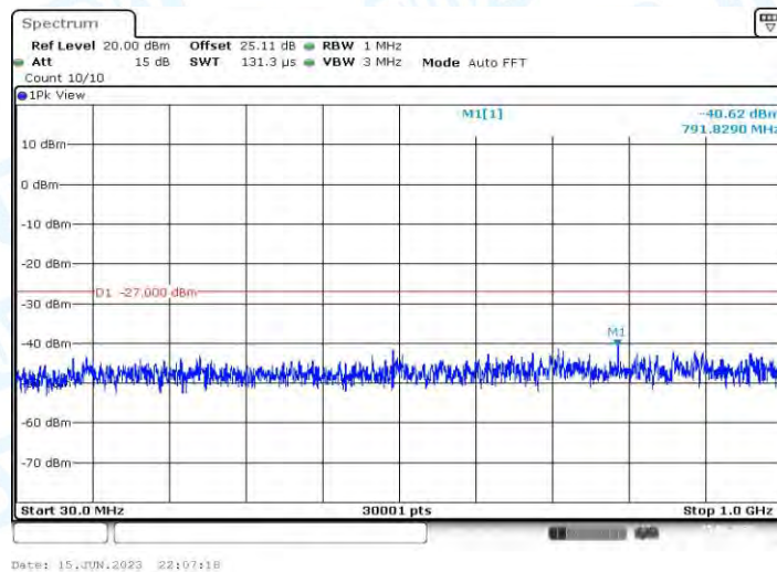
11AC20MIMO_Ant2_5745_30~1000
