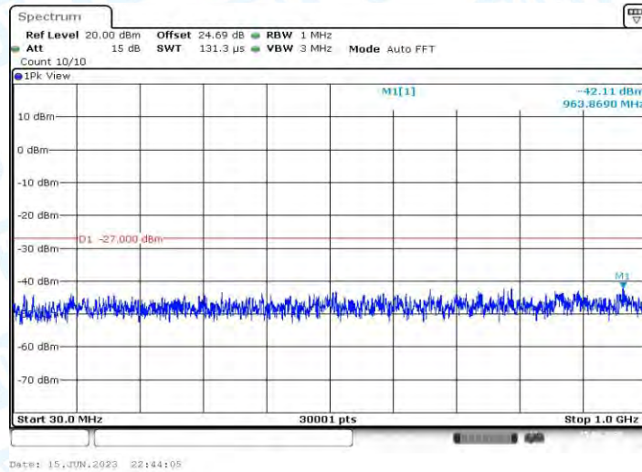
11AX20MIMO_Ant1_5280_30~1000
