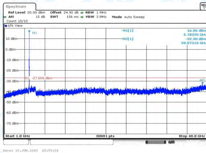
11AX20MIMO_Ant1_5785_1000~40000
