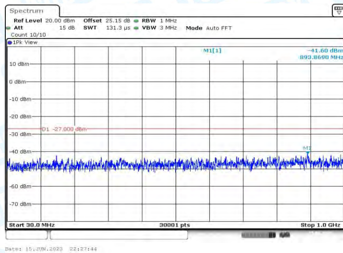
11AC40MIMO_Ant1_5755_30~1000
