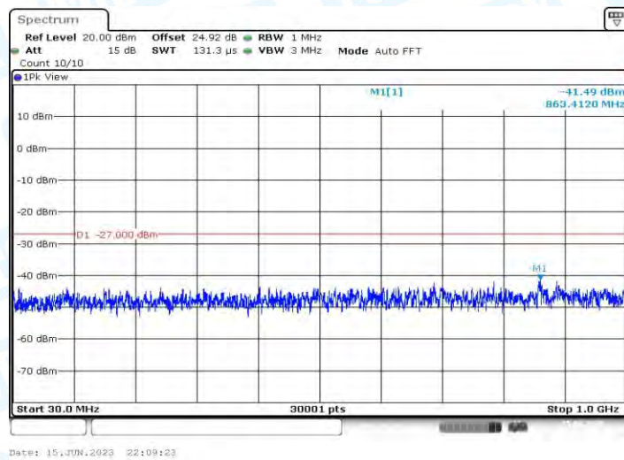
11AC20MIMO_Ant1_5785_30~1000
