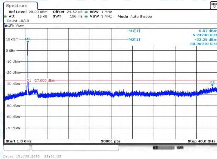
11AC80MIMO_Ant2_5210_1000~40000
