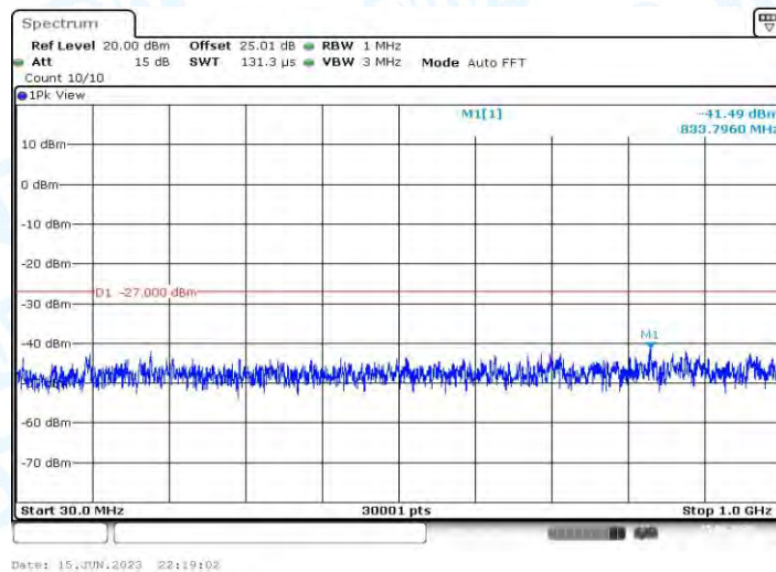
11AC40MIMO_Ant1_5550_30~1000
