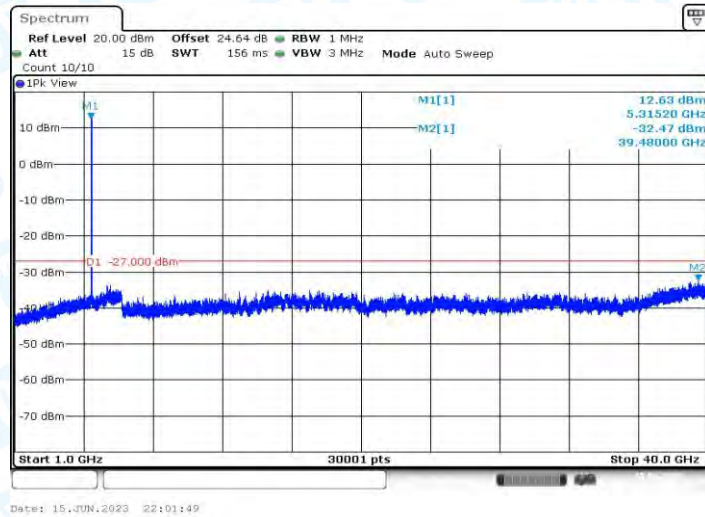
11AC20MIMO_Ant1_5320_1000~40000
