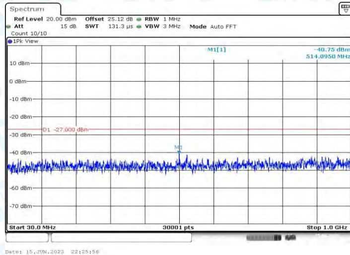
11AC40MIMO_Ant1_5670_30~1000
