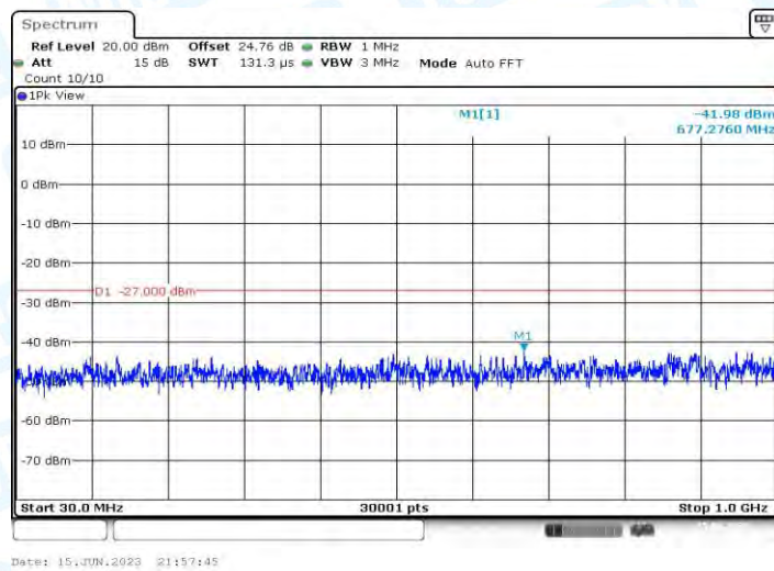
11AC20MIMO_Ant2_5240_30~1000
