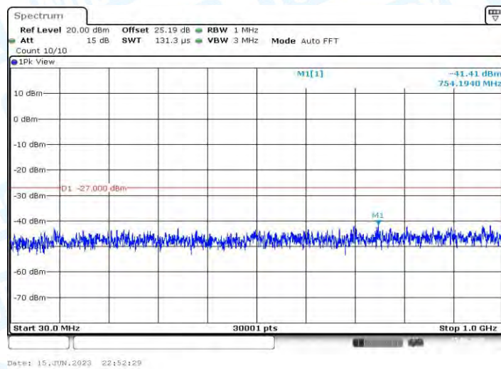
11AX20MIMO_Ant1_5700_30~1000
