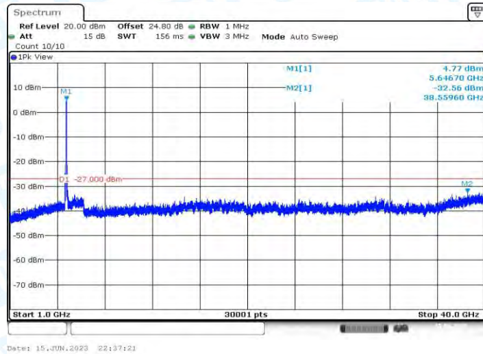
11AC80MIMO_Ant2_5610_1000~40000
