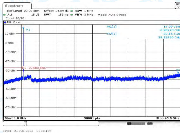
11AX20MIMO_Ant1_5280_1000~40000
