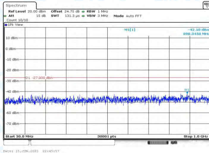
11AX20MIMO_Ant2_5320_30~1000
