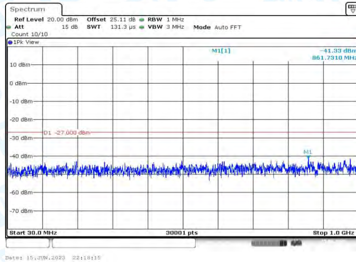
11AC40MIMO_Ant2_5510_30~1000
