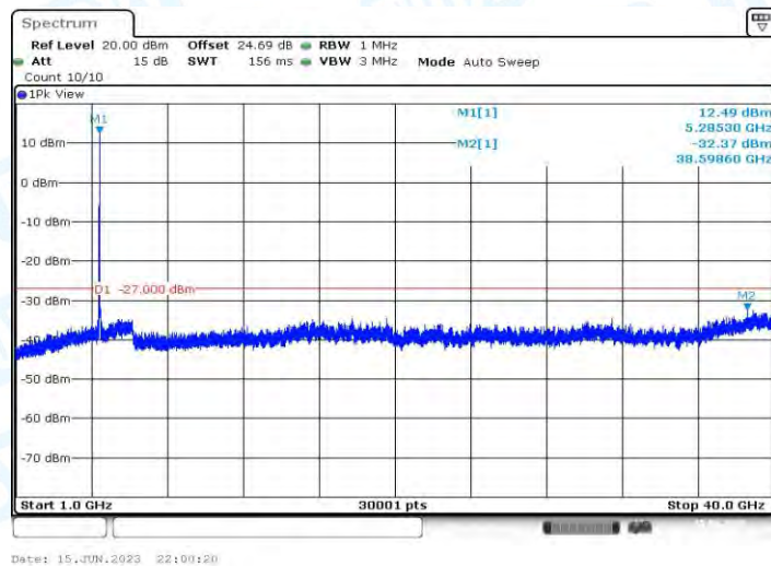
11AC20MIMO_Ant1_5280_1000~40000
