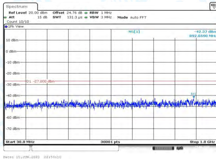
11AX40MIMO_Ant2_5230_30~1000
