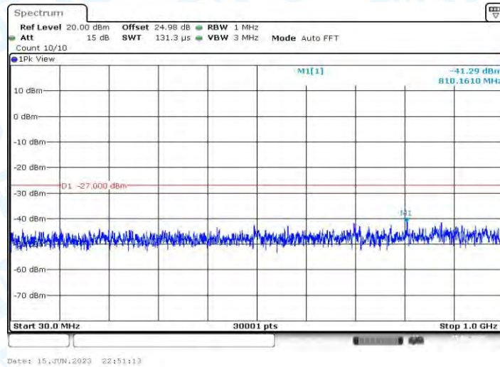
11AX20MIMO_Ant1_5580_30~1000
