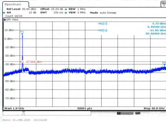
11AC80MIMO_Ant1_5530_1000~40000
