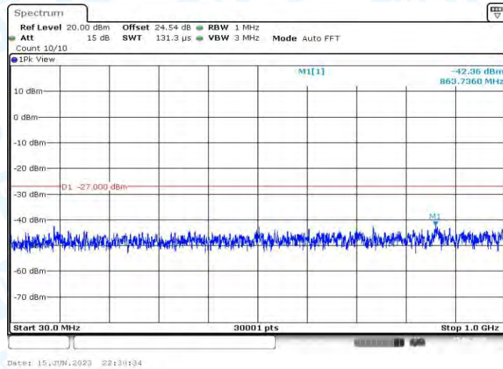
11AC80MIMO_Ant1_5210_30~1000
