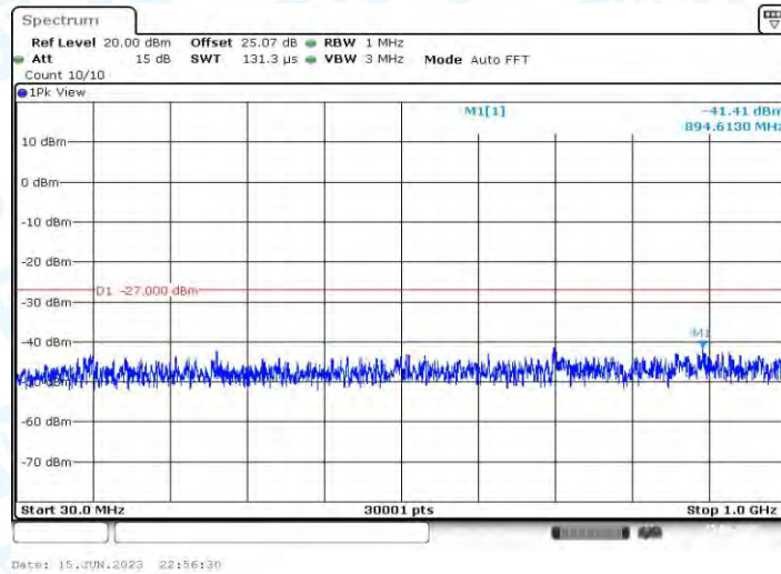
11AX20MIMO_Ant2_5825_30~1000
