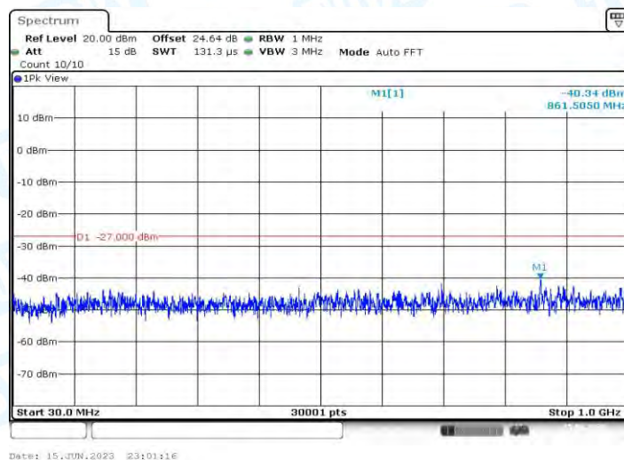
11AX40MIMO_Ant1_5310_30~1000
