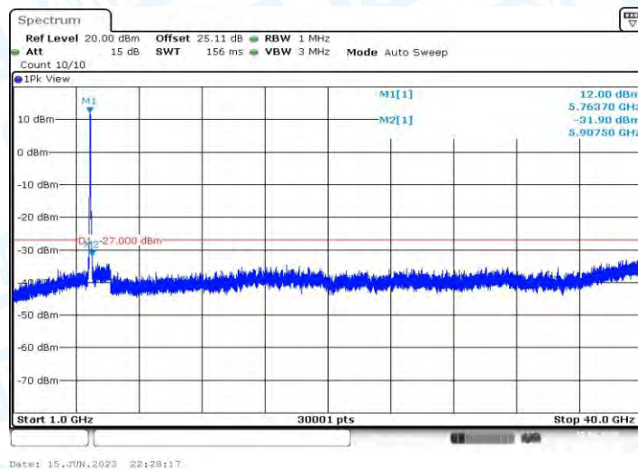
11AC40MIMO_Ant2_5755_1000~40000
