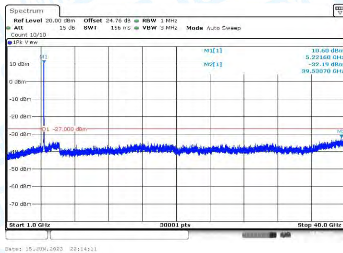
11AC40MIMO_Ant2_5230_1000~40000
