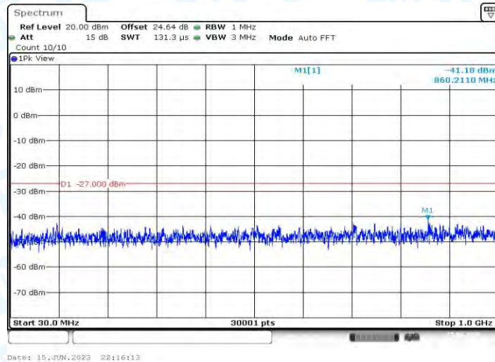
11AC40MIMO_Ant1_5310_30~1000
