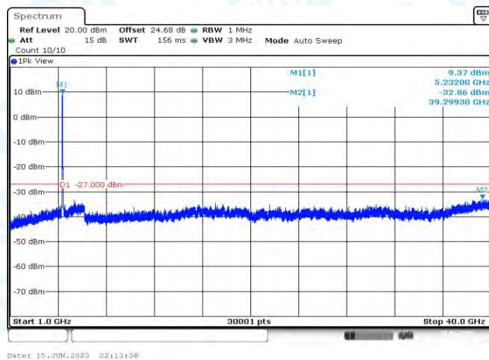
11AC40MIMO_Ant1_5230_1000~40000
