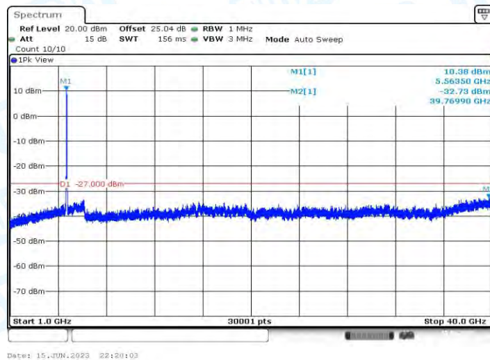
11AC40MIMO_Ant2_5550_1000~40000
