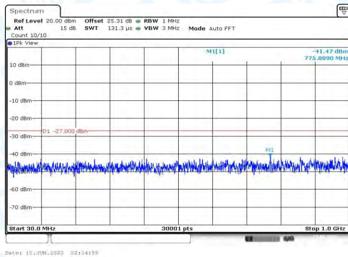
11AC80MIMO_Ant2_5530_30~1000
