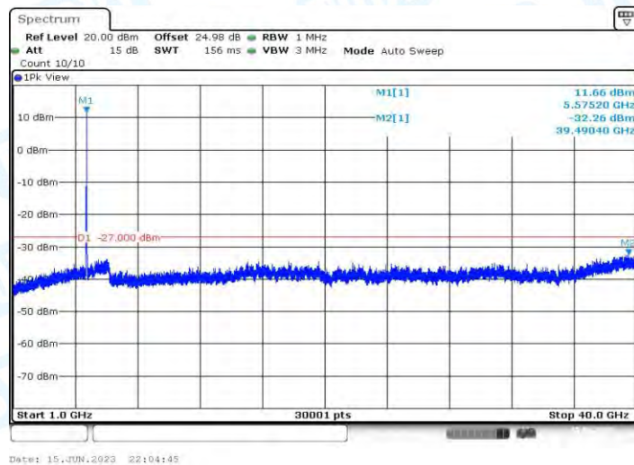
11AC20MIMO_Ant1_5580_1000~40000
