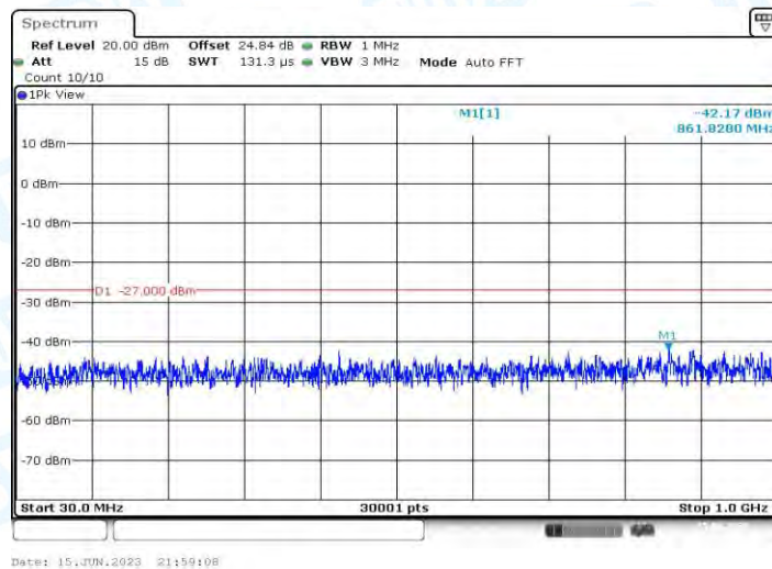
11AC20MIMO_Ant2_5260_30~1000
