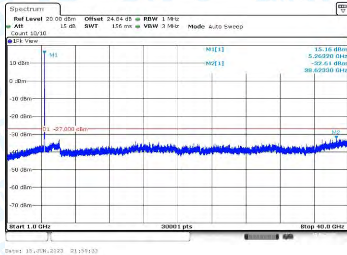
11AC20MIMO_Ant2_5260_1000~40000
