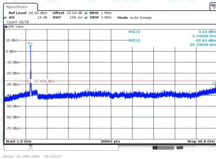
11AC80MIMO_Ant2_5775_1000~40000
