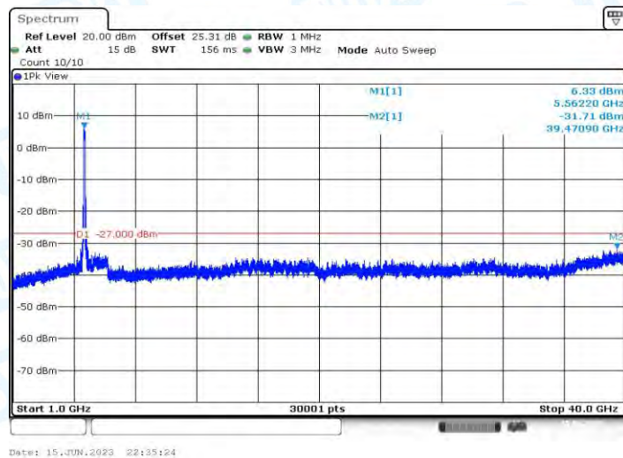
11AC80MIMO_Ant2_5530_1000~40000
