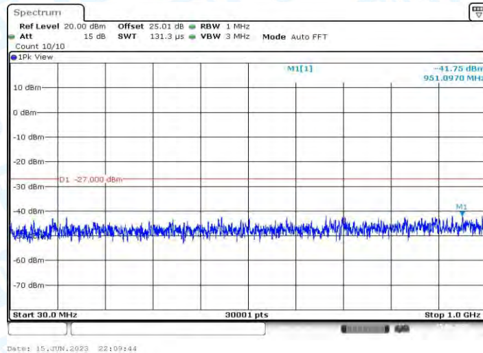
11AC20MIMO_Ant2_5785_30~1000
