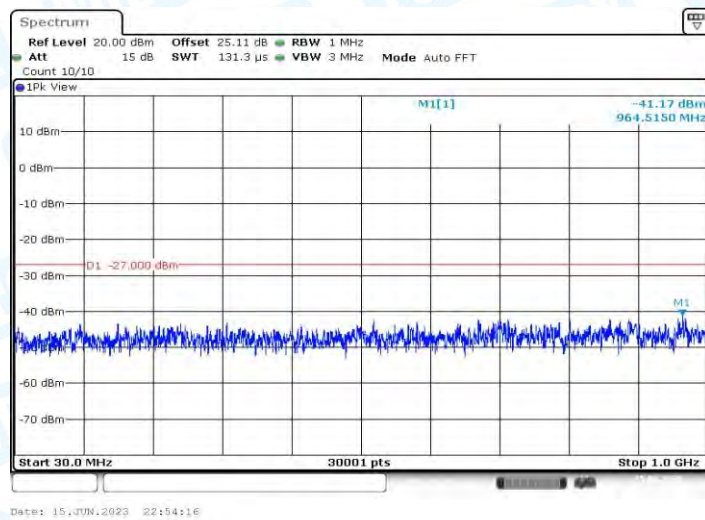
11AX20MIMO_Ant2_5745_30~1000
