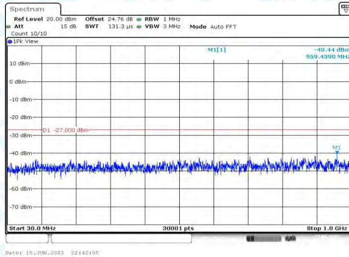
11AX20MIMO_Ant2_5240_30~1000
