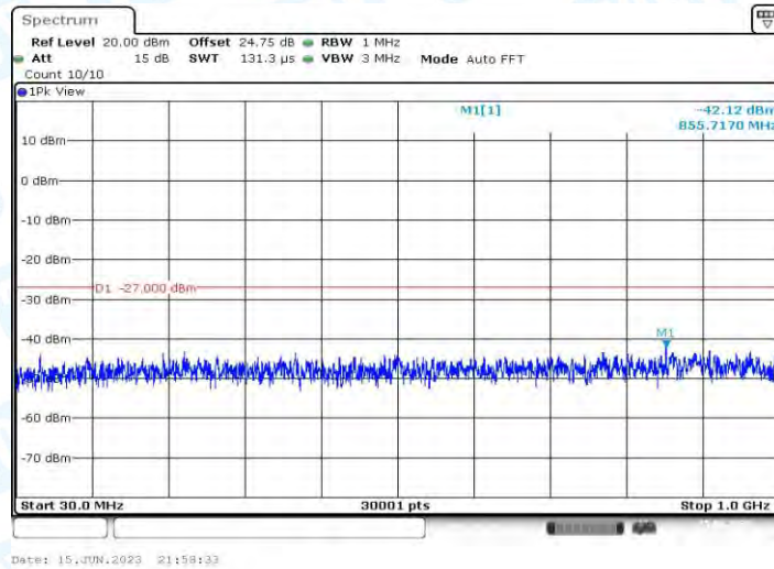
11AC20MIMO_Ant1_5260_30~1000
