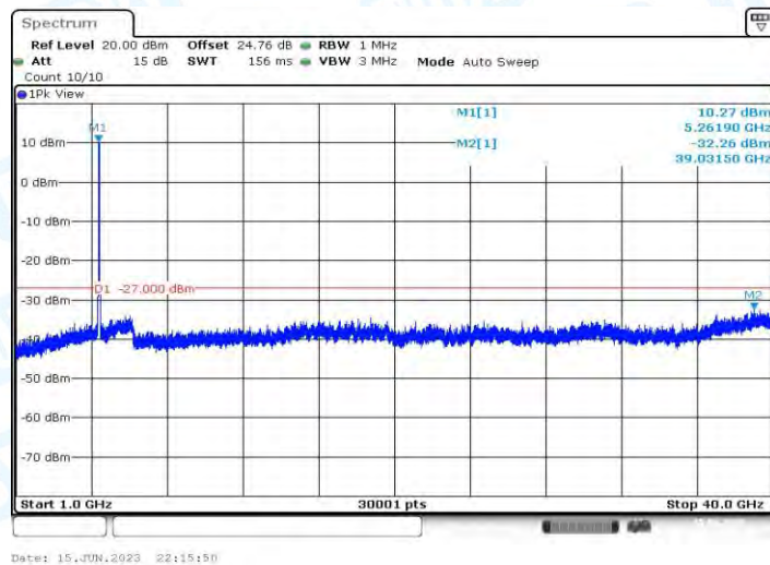
11AC40MIMO_Ant2_5270_1000~40000
