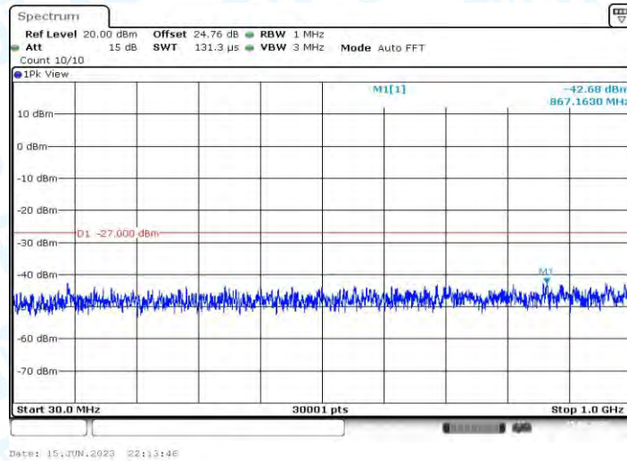
11AC40MIMO_Ant2_5230_30~1000
