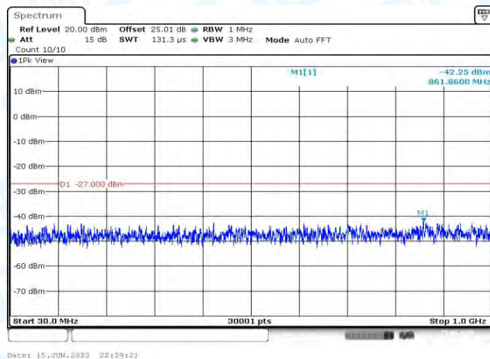
11AC40MIMO_Ant2_5795_30~1000
