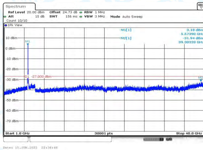
11AC80MIMO_Ant1_5610_1000~40000
