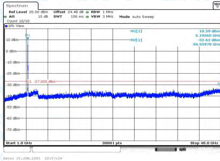
11AX40MIMO_Ant1_5190_1000~40000
