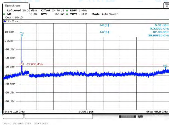
11AC80MIMO_Ant1_5290_1000~40000
