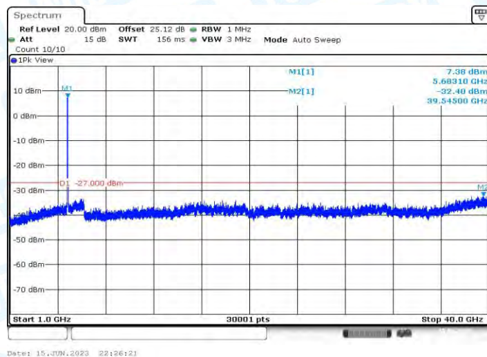
11AC40MIMO_Ant1_5670_1000~40000
