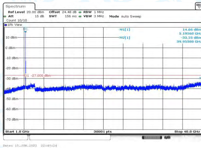
11AX20MIMO_Ant1_5200_1000~40000
