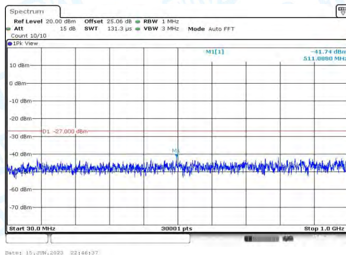
11AX20MIMO_Ant1_5500_30~1000
