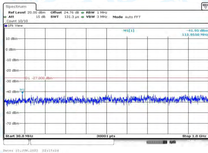
11AC40MIMO_Ant2_5270_30~1000
