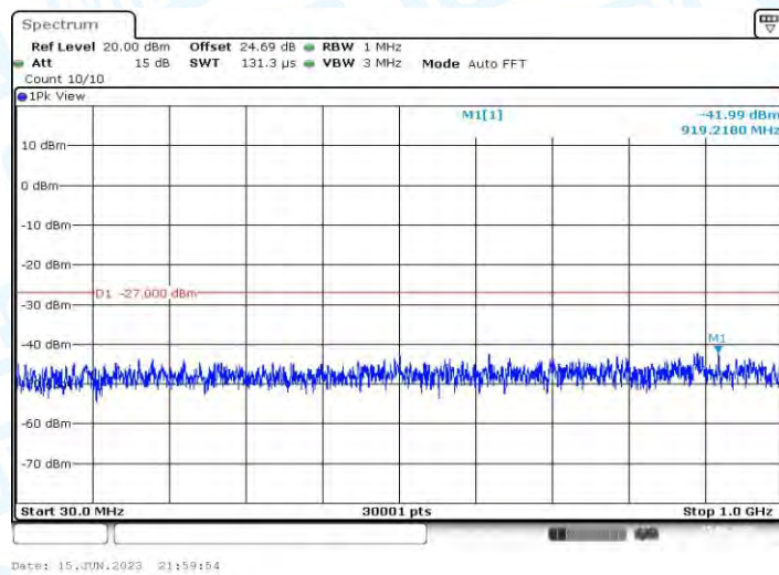
11AC20MIMO_Ant1_5280_30~1000
