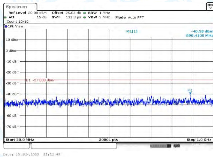
11AC40MIMO_Ant1_5510_30~1000
