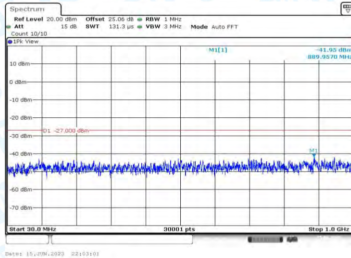
11AC20MIMO_Ant1_5500_30~1000
