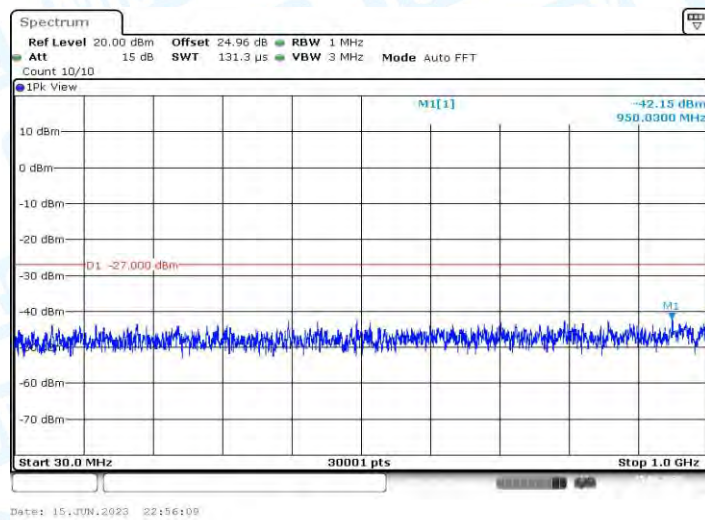
11AX20MIMO_Ant1_5825_30~1000
