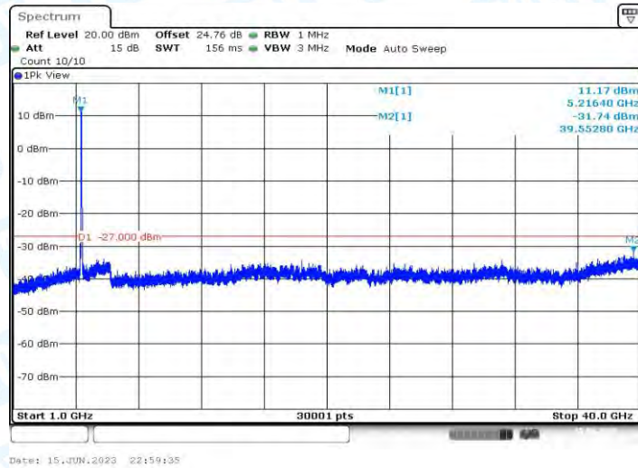
11AX40MIMO_Ant2_5230_1000~40000
