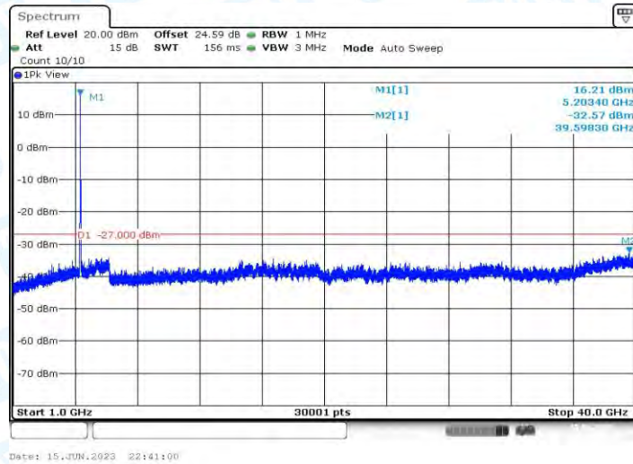
11AX20MIMO_Ant2_5200_1000~40000
