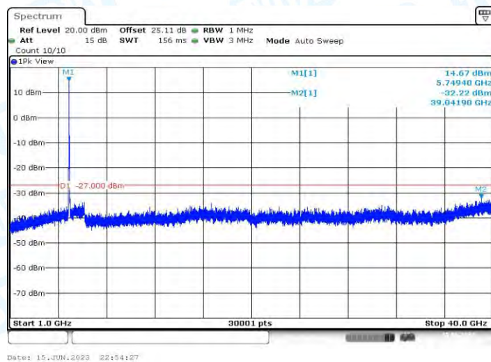
11AX20MIMO_Ant2_5745_1000~40000
