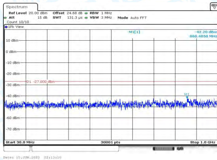
11AC40MIMO_Ant1_5230_30~1000
