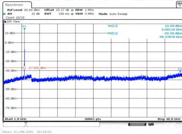
11AC20MIMO_Ant2_5500_1000~40000
