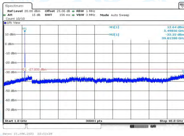
11AC20MIMO_Ant1_5500_1000~40000
