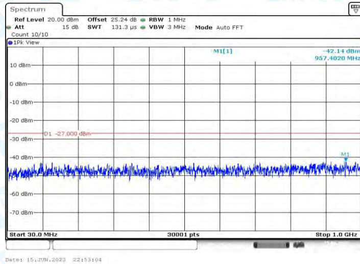
11AX20MIMO_Ant2_5700_30~1000
