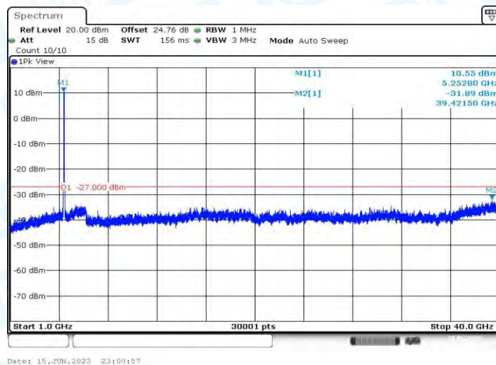
11AX40MIMO_Ant2_5270_1000~40000
