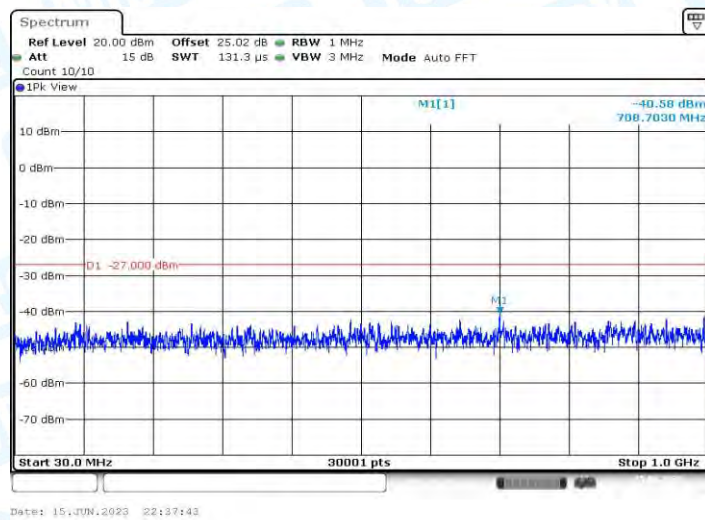
11AC80MIMO_Ant1_5775_30~1000
