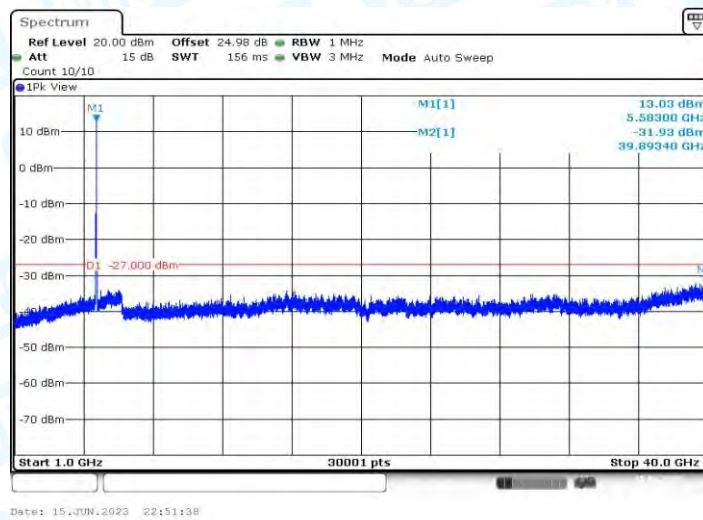
11AX20MIMO_Ant1_5580_1000~40000
