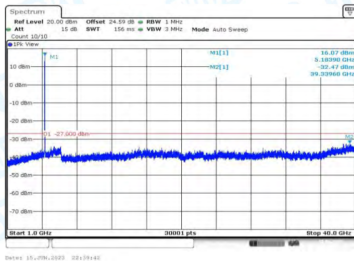
11AX20MIMO_Ant2_5180_1000~40000
