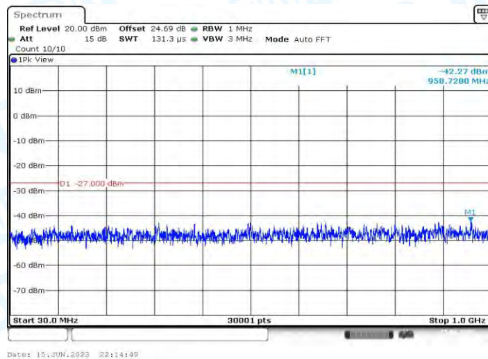
11AC40MIMO_Ant1_5270_30~1000
