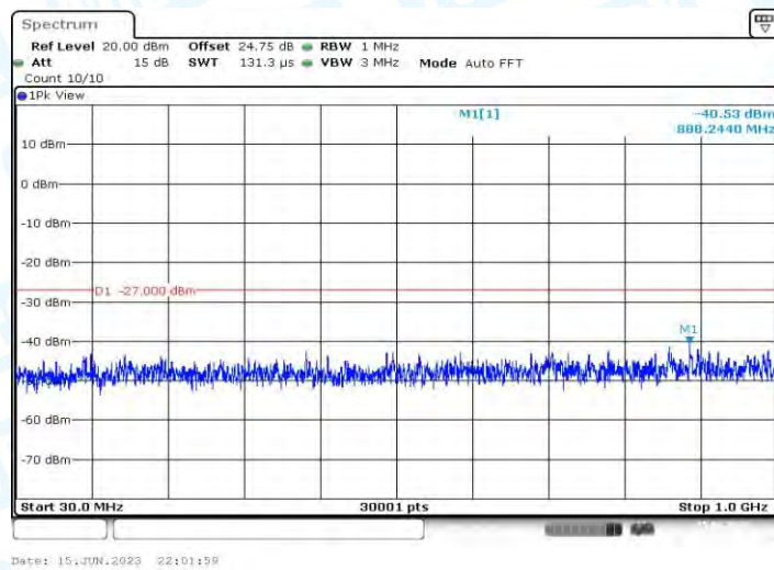
11AC20MIMO_Ant2_5320_30~1000
