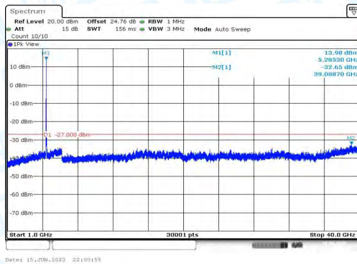
11AC20MIMO_Ant2_5280_1000~40000
