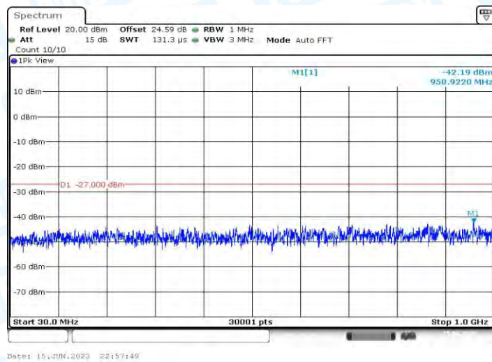
11AX40MIMO_Ant2_5190_30~1000
