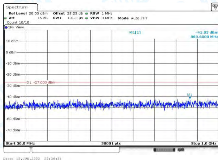
11AC40MIMO_Ant2_5670_30~1000
