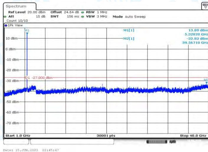
11AX20MIMO_Ant1_5320_1000~40000
