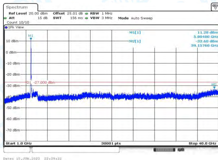
11AC40MIMO_Ant2_5795_1000~40000
