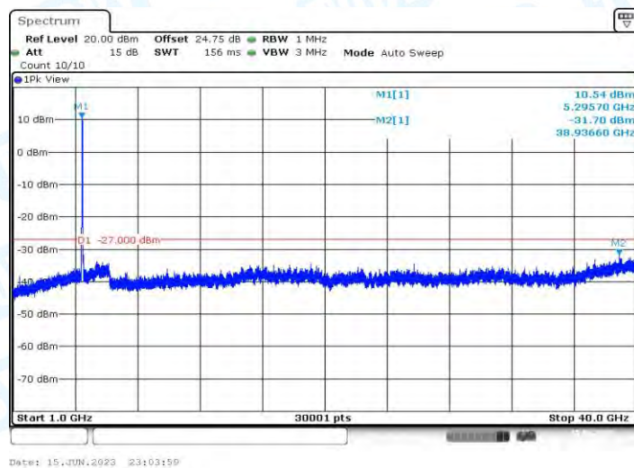
11AX40MIMO_Ant2_5310_1000~40000
