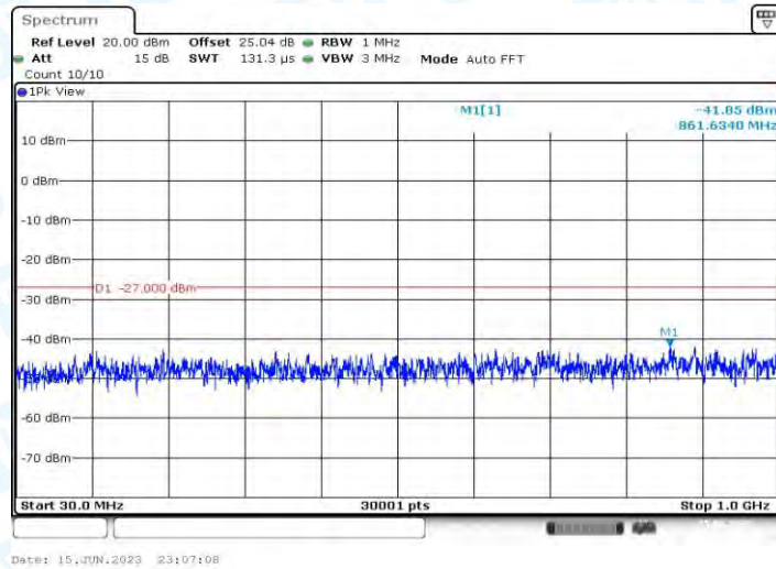
11AX40MIMO_Ant2_5550_30~1000
