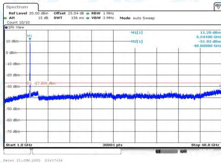
11AX40MIMO_Ant2_5550_1000~40000
