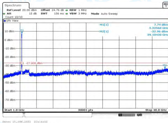
11AX80MIMO_Ant1_5290_1000~40000
