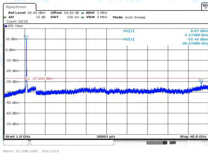
11AX80MIMO_Ant2_5210_1000~40000
