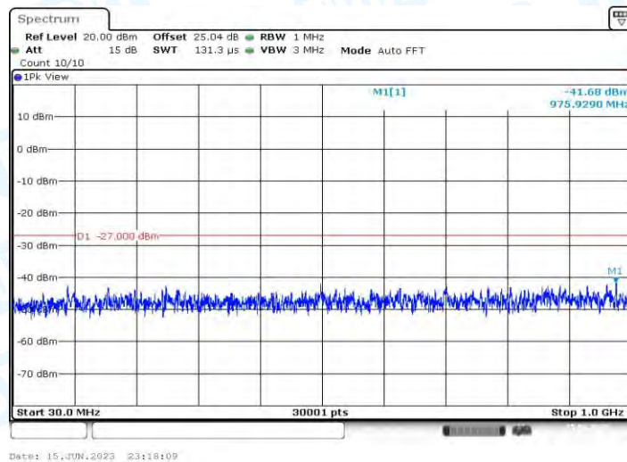
11AX80MIMO_Ant2_5775_30~1000
