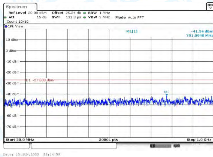
11AX80MIMO_Ant1_5530_30~1000
