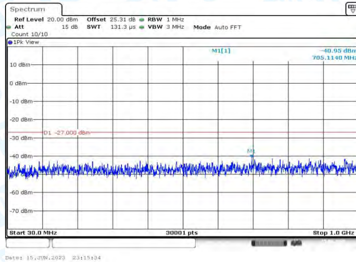
11AX80MIMO_Ant2_5530_30~1000
