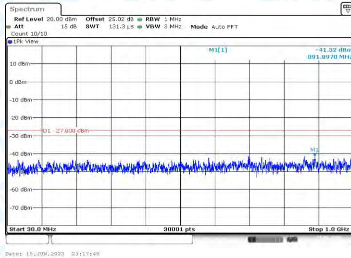
11AX80MIMO_Ant1_5775_30~1000
