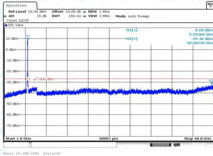
11AX80MIMO_Ant2_5290_1000~40000
