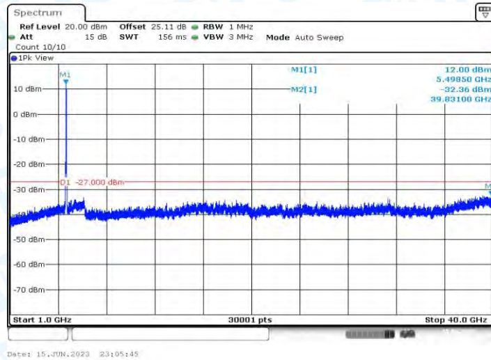
11AX40MIMO_Ant2_5510_1000~40000
