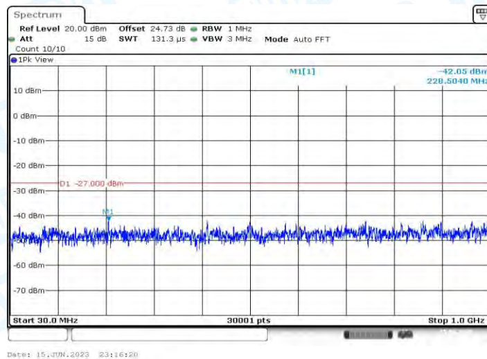
11AX80MIMO_Ant1_5610_30~1000
