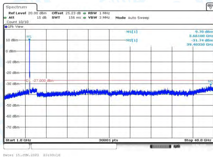
11AX40MIMO_Ant2_5670_1000~40000
