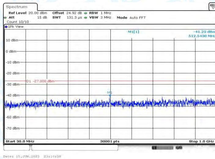
11AX40MIMO_Ant1_5795_30~1000
