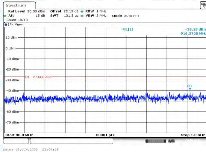
11AX40MIMO_Ant1_5755_30~1000
