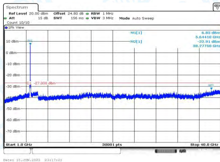
11AX80MIMO_Ant2_5610_1000~40000
