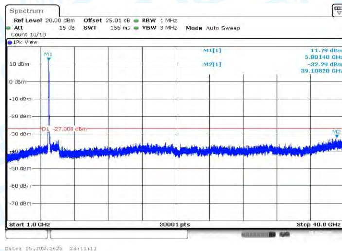
11AX40MIMO_Ant2_5795_1000~40000
