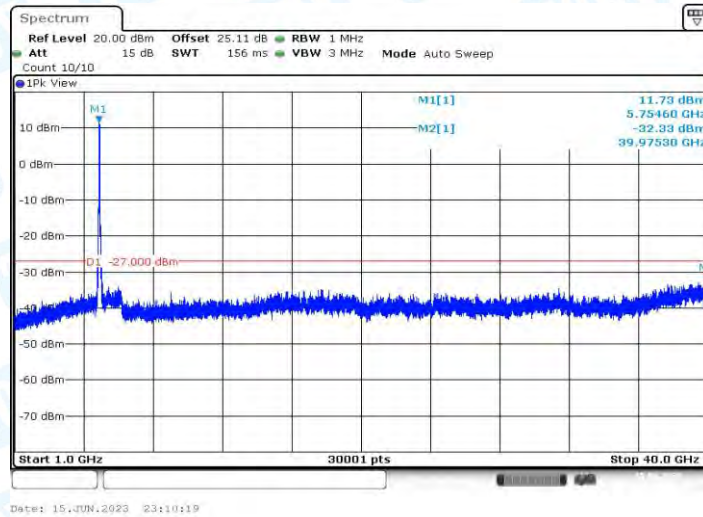
11AX40MIMO_Ant2_5755_1000~40000
