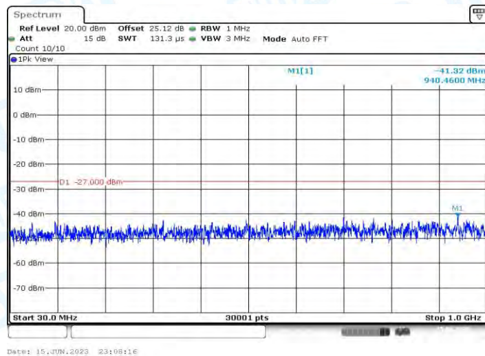
11AX40MIMO_Ant1_5670_30~1000
