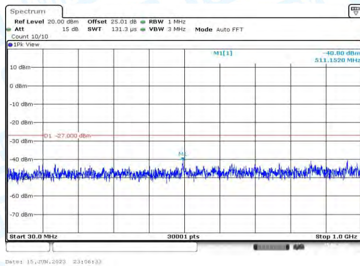
11AX40MIMO_Ant1_5550_30~1000
