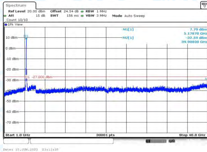
11AX80MIMO_Ant1_5210_1000~40000
