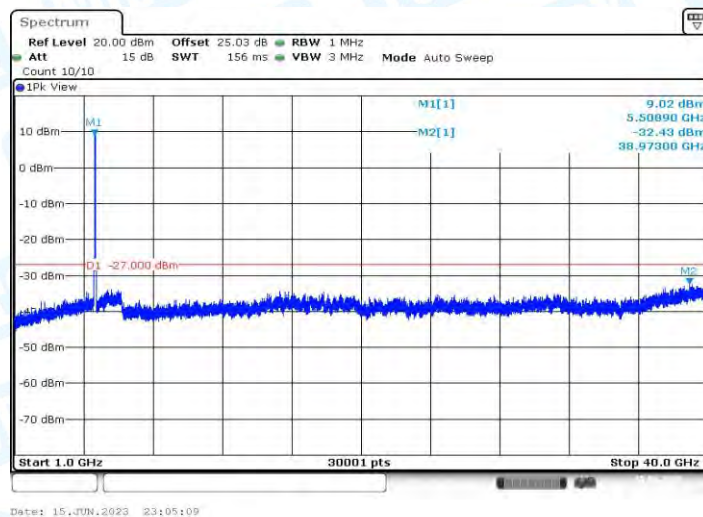
11AX40MIMO_Ant1_5510_1000~40000
