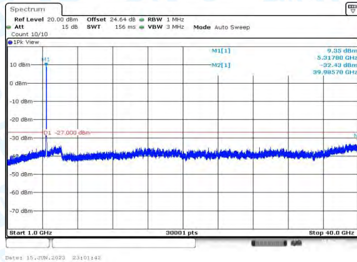
11AX40MIMO_Ant1_5310_1000~40000
