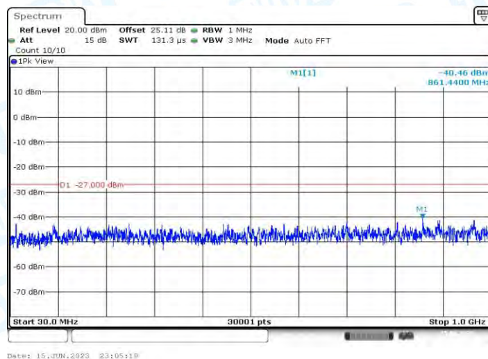
11AX40MIMO_Ant2_5510_30~1000
