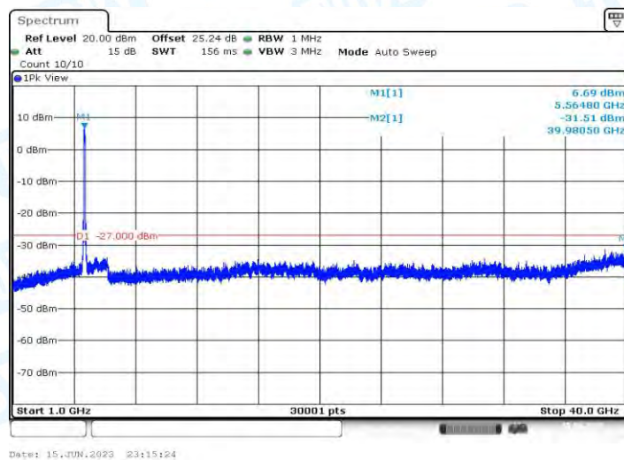
11AX80MIMO_Ant1_5530_1000~40000
