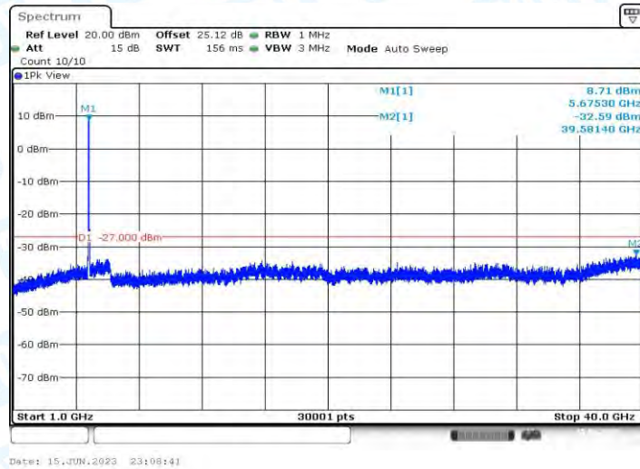
11AX40MIMO_Ant1_5670_1000~40000
