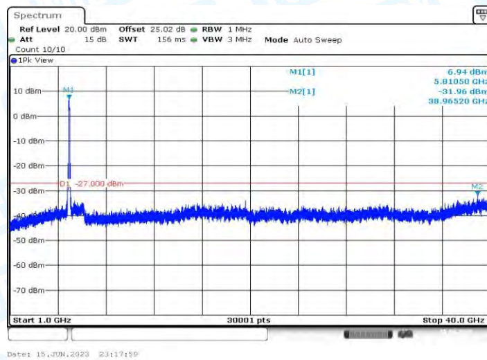
11AX80MIMO_Ant1_5775_1000~40000
