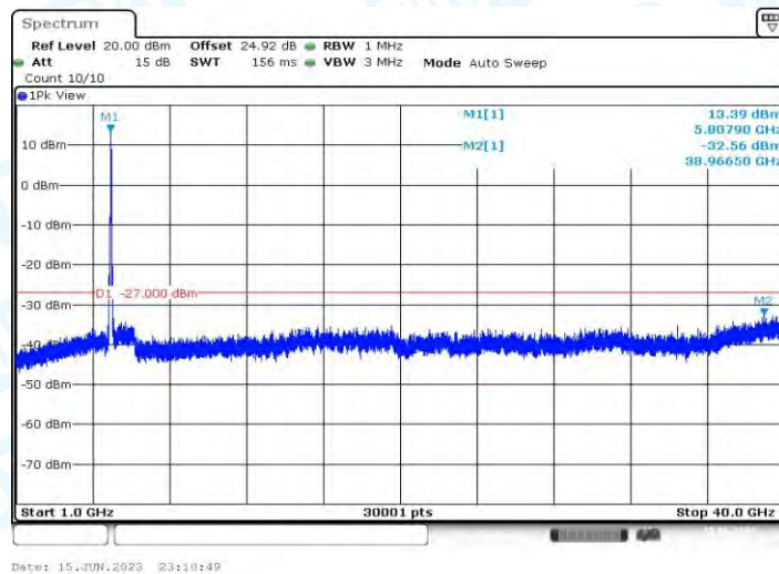
11AX40MIMO_Ant1_5795_1000~40000
