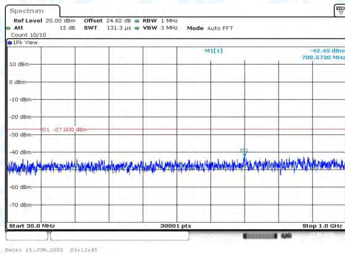
11AX80MIMO_Ant2_5210_30~1000
