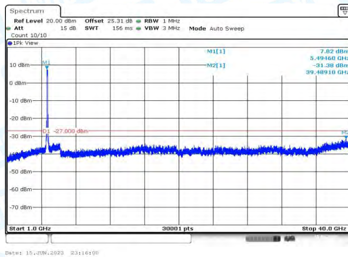
11AX80MIMO_Ant2_5530_1000~40000
