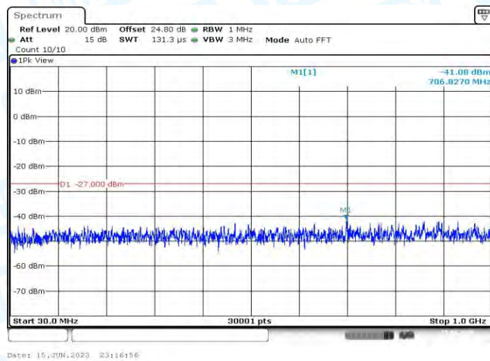
11AX80MIMO_Ant2_5610_30~1000
