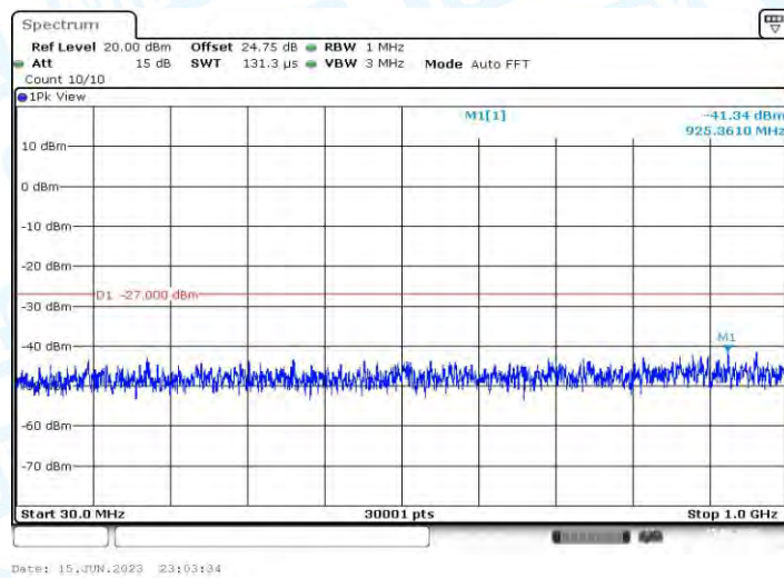
11AX40MIMO_Ant2_5310_30~1000
