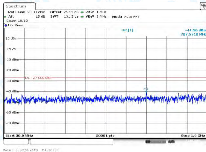
11AX40MIMO_Ant2_5755_30~1000
