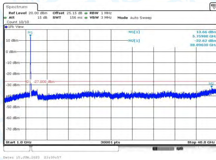
11AX40MIMO_Ant1_5755_1000~40000
