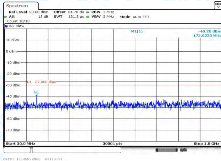
11AX80MIMO_Ant1_5290_30~1000
