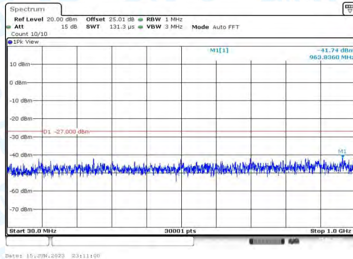
11AX40MIMO_Ant2_5795_30~1000
