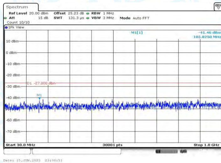
11AX40MIMO_Ant2_5670_30~1000
