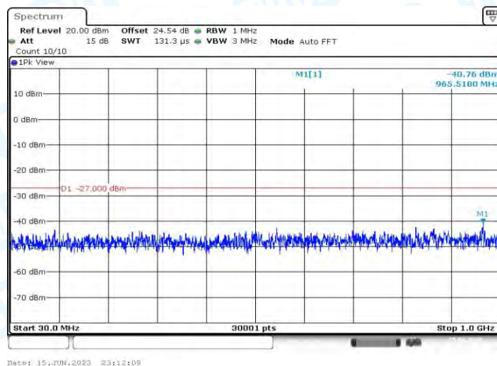
11AX80MIMO_Ant1_5210_30~1000
