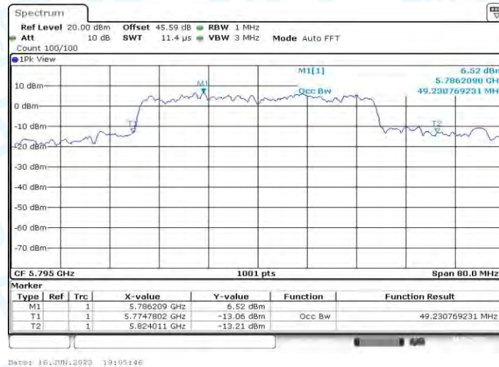
11AX40MIMO_Ant1_5795
