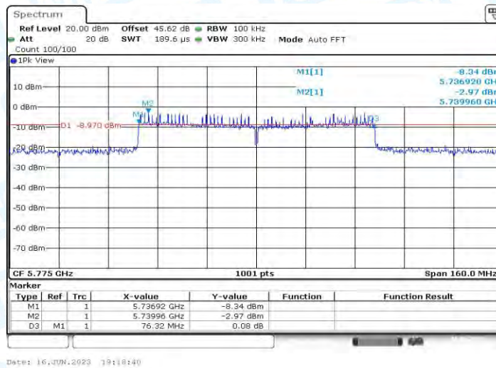
11AC80MIMO_Ant1&Ant.2_5775
