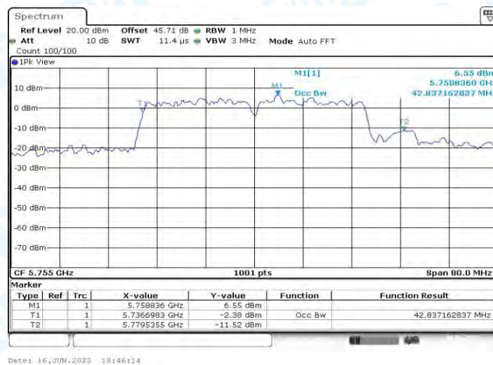
11N40MIMO_Ant1_5755
