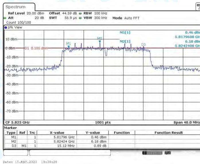
11N20MIMO_Ant1&Ant.2_5825
