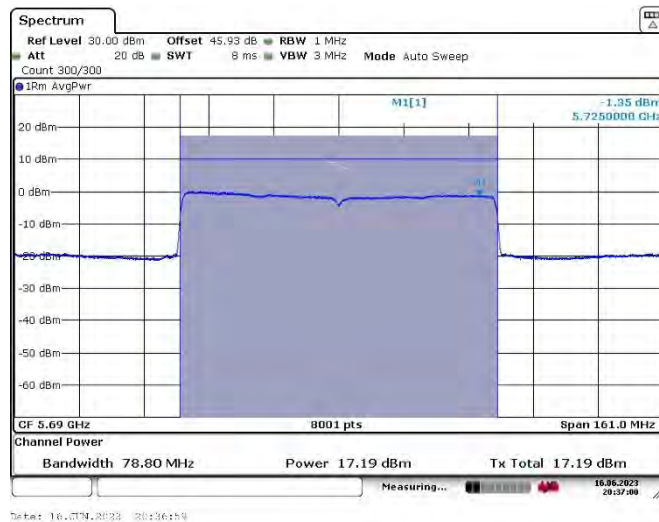
11AX80_Ant1&Ant2
