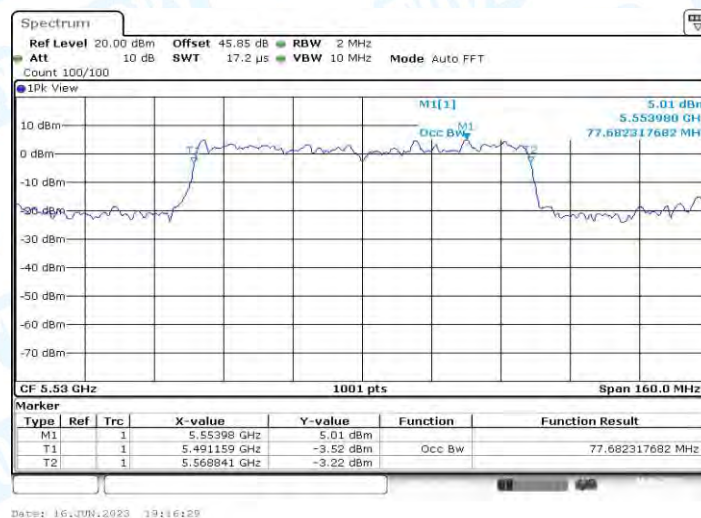
11AC80MIMO_Ant1_5530
