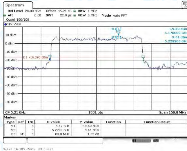
11AX80MIMO_Ant1&Ant.2_5210
