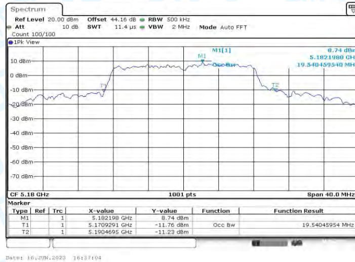
11A_Ant1_5180
