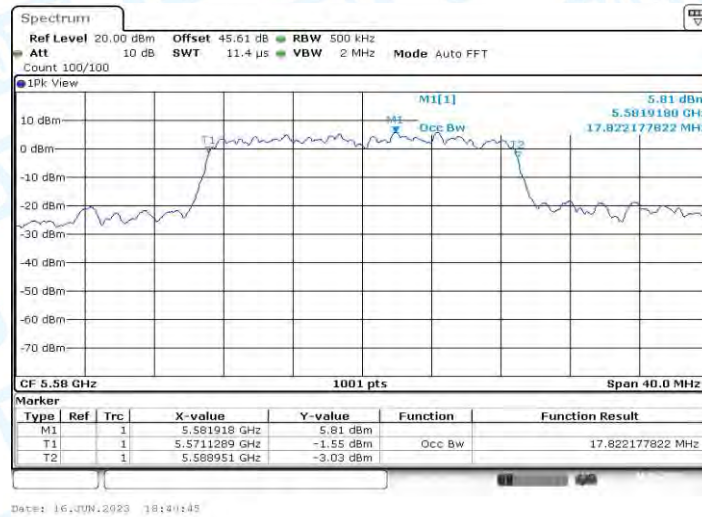
11N20MIMO_Ant1_5580
