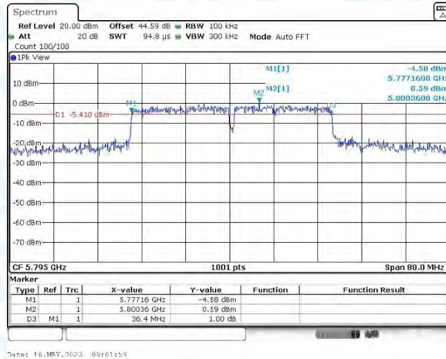
11AC40MIMO_Ant1&Ant.2_5795
