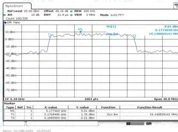
11AX20MIMO_Ant1_5180
