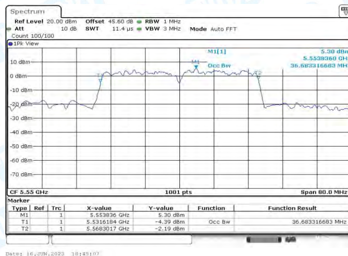
11N40MIMO_Ant1_5550
