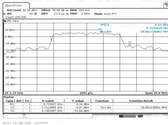
11A_Ant2_5720
