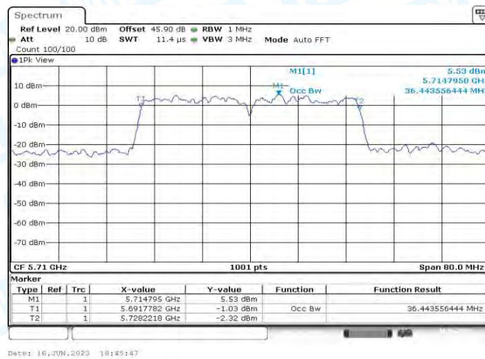
11N40MIMO_Ant1_5710
