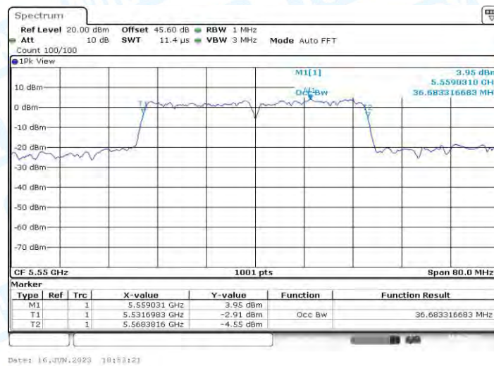
11AC40MIMO_Ant1_5550
