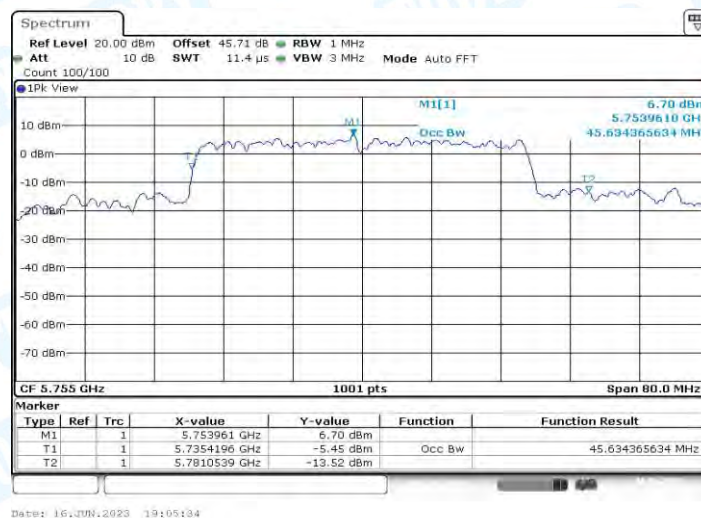
11AX40MIMO_Ant1_5755
