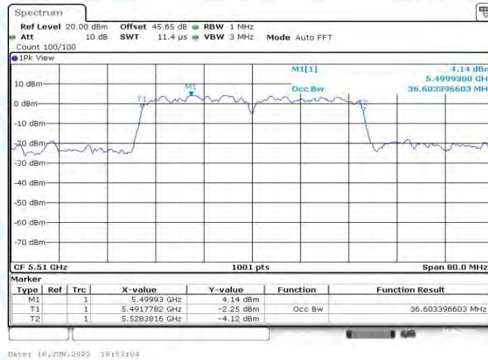
11AC40MIMO_Ant1_5510
