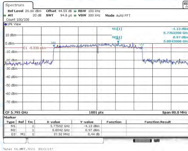
11AX40MIMO_Ant1&Ant.2_5795
