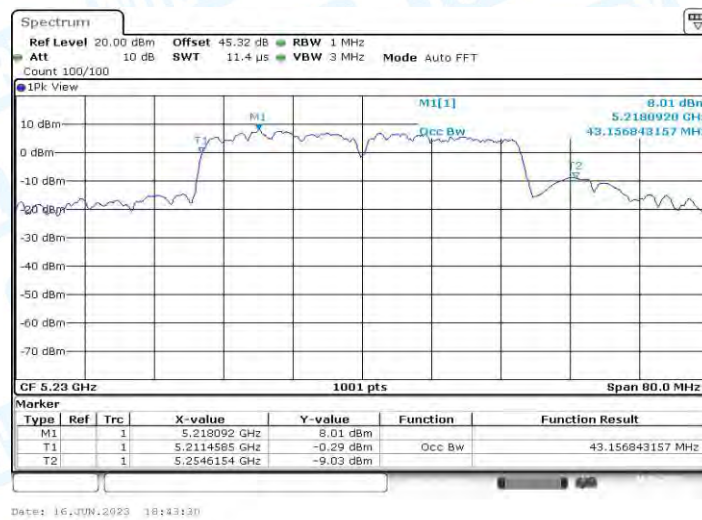
11N40MIMO_Ant1_5230
