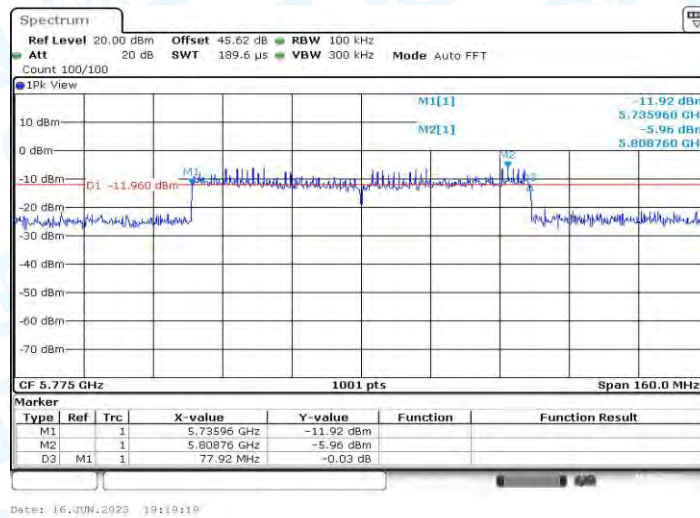
11AX80MIMO_Ant1&Ant.2_5775
