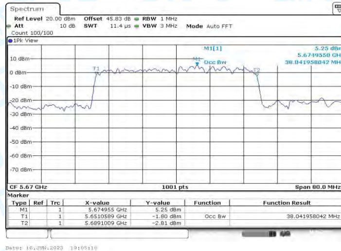
11AX40MIMO_Ant1_5670
