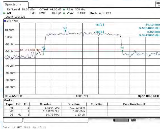
11AX40MIMO_Ant1&Ant.2_5550
