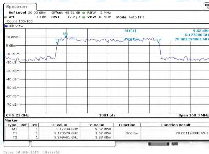
11AX80MIMO_Ant1_5210
