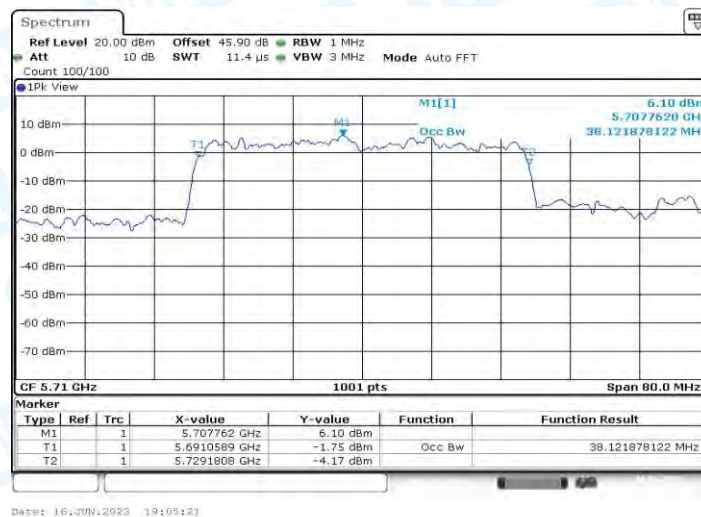
11AX40MIMO_Ant1_5710
