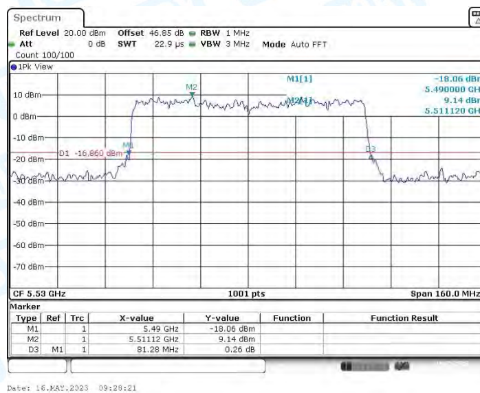
11AX80MIMO_Ant1&Ant.2_5530
