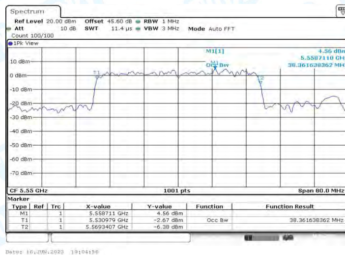
11AX40MIMO_Ant1_5550
