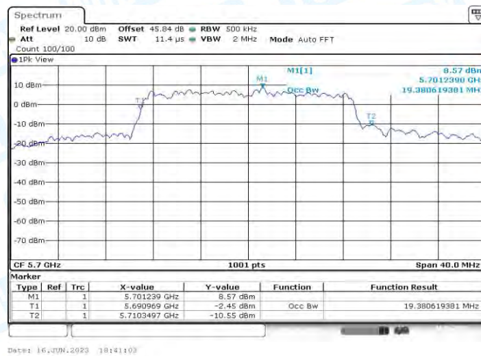
11N20MIMO_Ant1_5700
