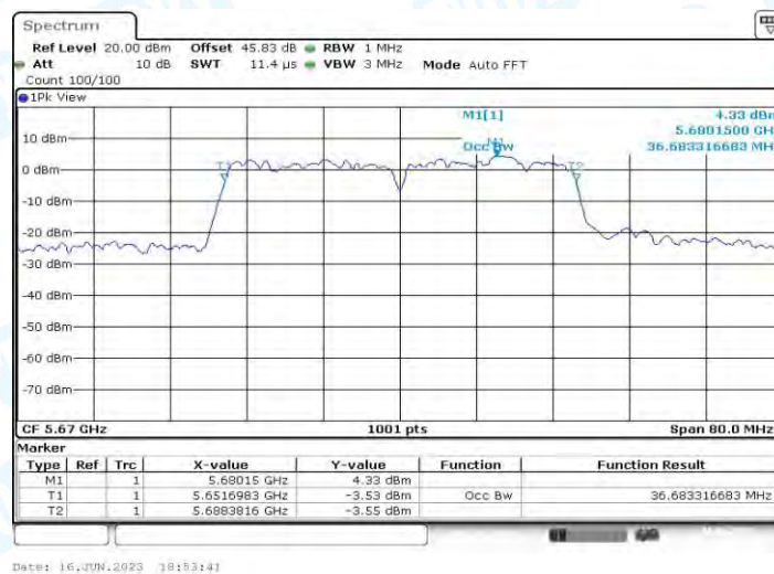
11AC40MIMO_Ant1_5670
