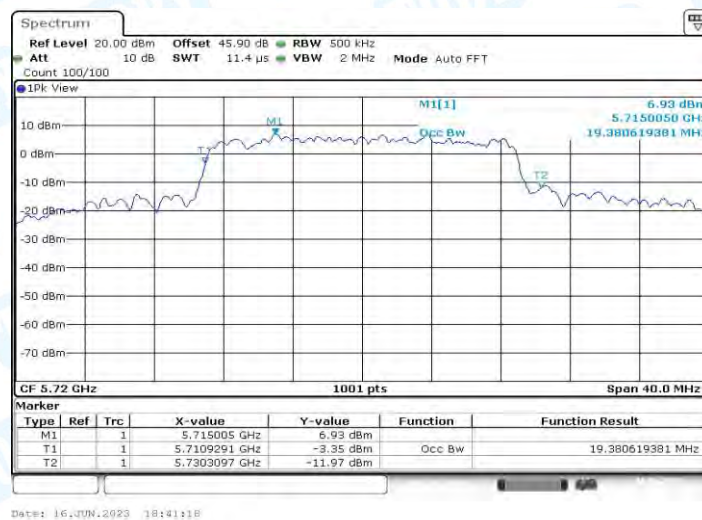
11N20MIMO_Ant1_5720
