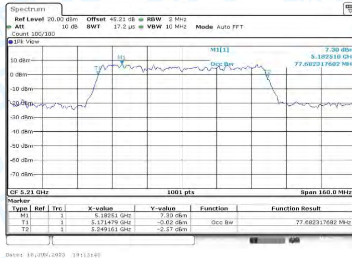
11AC80MIMO_Ant1_5210
