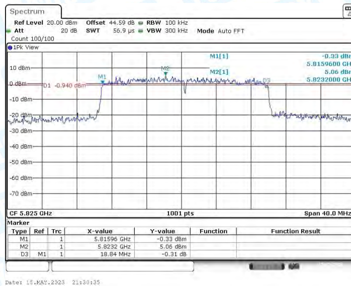
11AX20MIMO_Ant1&Ant.2_5825
