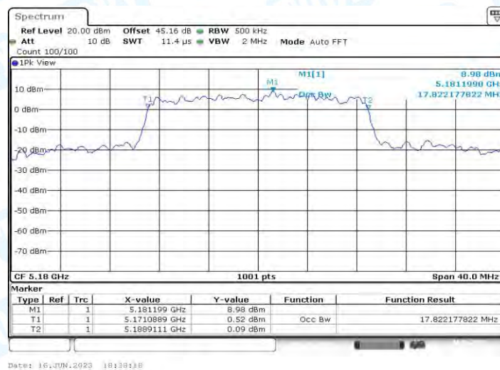
11N20MIMO_Ant1_5180
