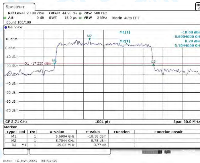
11AX40MIMO_Ant1&Ant.2_5710
