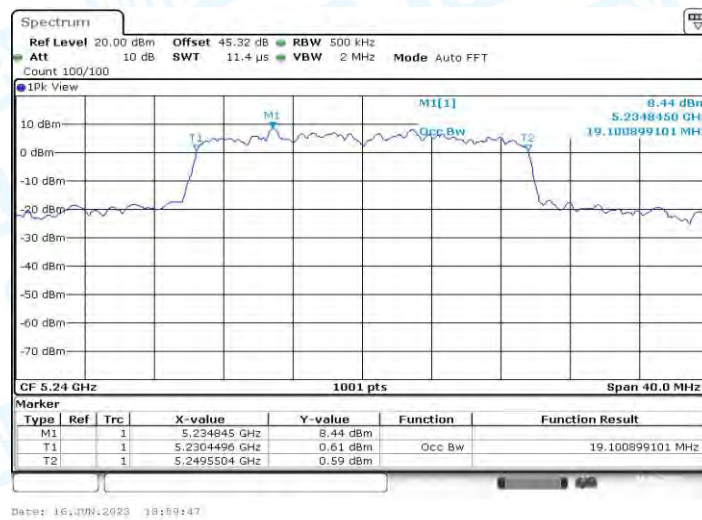
11AX20MIMO_Ant1_5240
