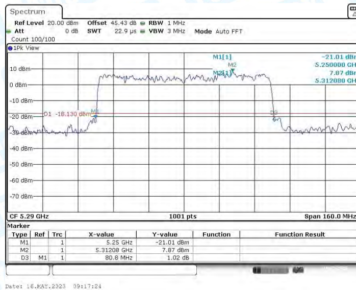
11AX80MIMO_Ant1&Ant.2_5290
