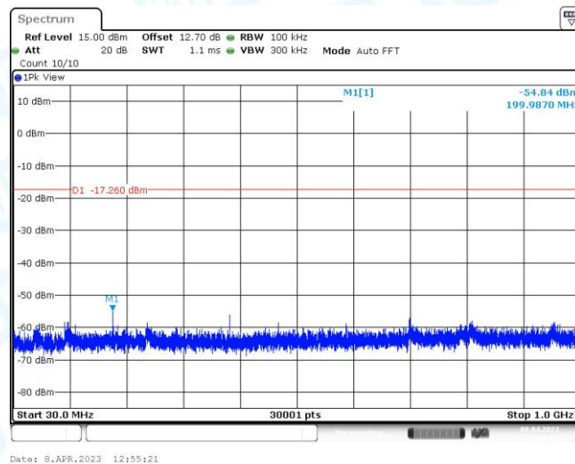
BLE_1M_2402_30~1000
