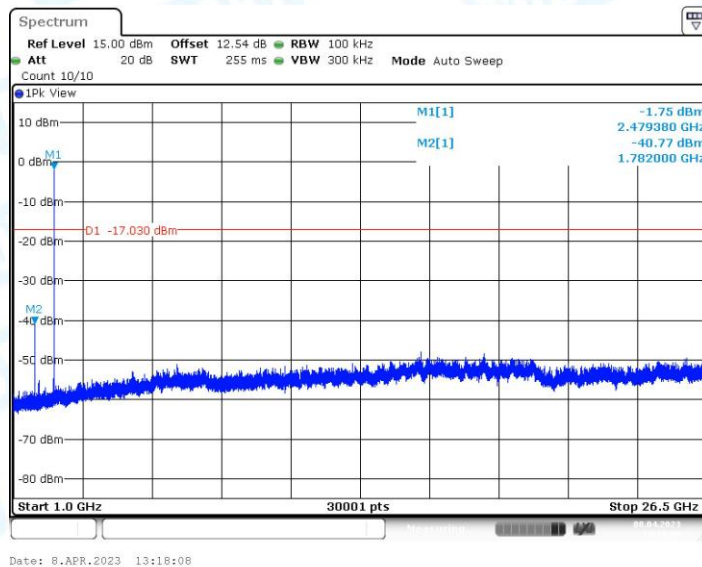
BLE_2M_2480_1000~26500
