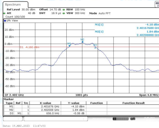
DTS-BLE_1M_2402
