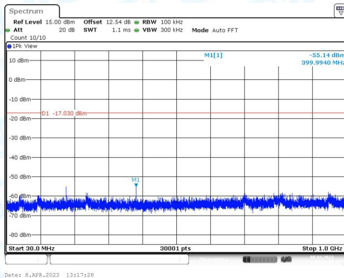
BLE_2M_2480_30~1000
