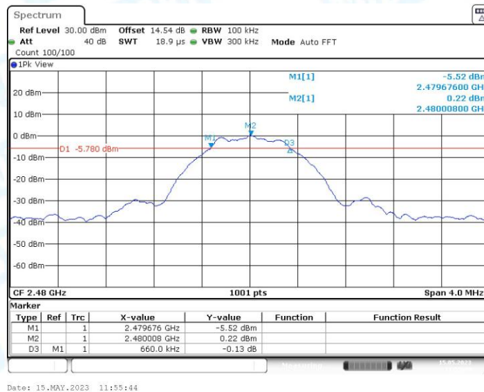
DTS-BLE_1M_2480
