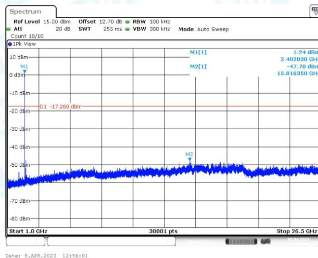
BLE_1M_2402_1000~26500
