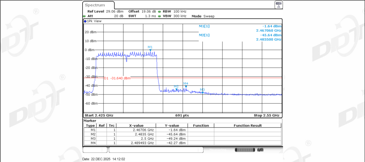
11AX40MIMO_Ant2_High_2452
