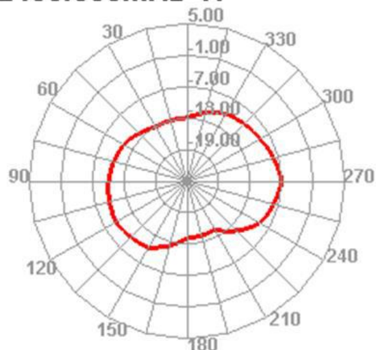
2450.000MHz H
