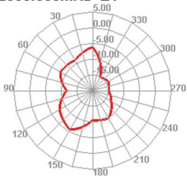
2500.000MHz E1
