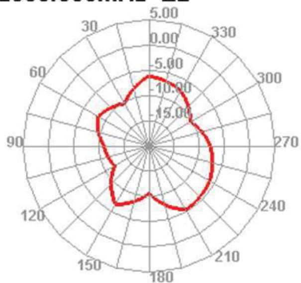
2500.000MHz E2
