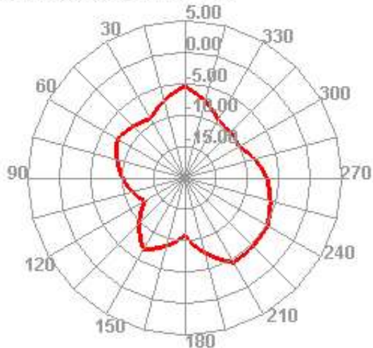
2450.000MHz E2
