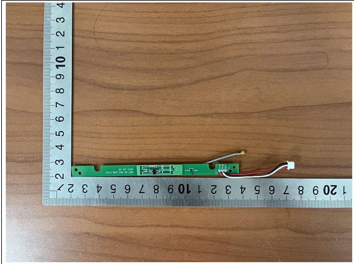
RFID Antenna (M/N: XM7-40 Ant_Sub-v100)
