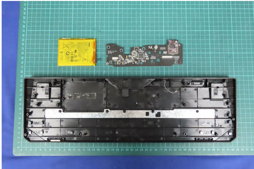
(14) EUT Photo
