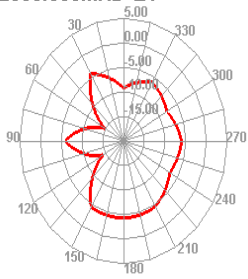
2500.000MHz E1
