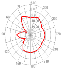
2500.000MHz
