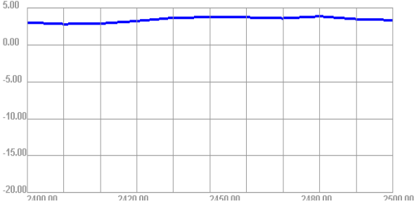
2400.00MHz - 2500.00MHz Efficiency
