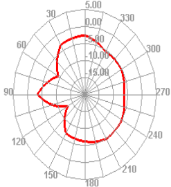
2400.000MHz E1
