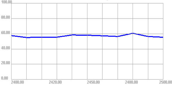
2400.00MHz - 2500.00MHz Efficiency
