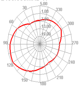
2450.000MHz H
