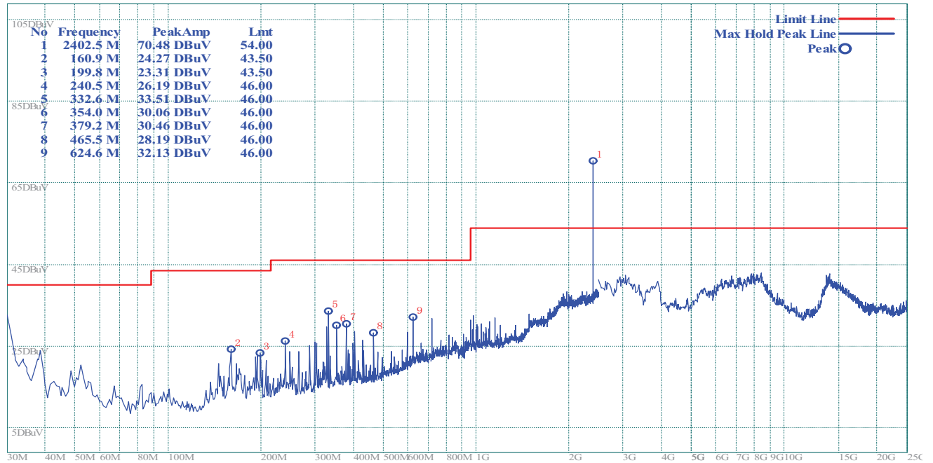
(Plot A.1: Antenna Horizontal)
