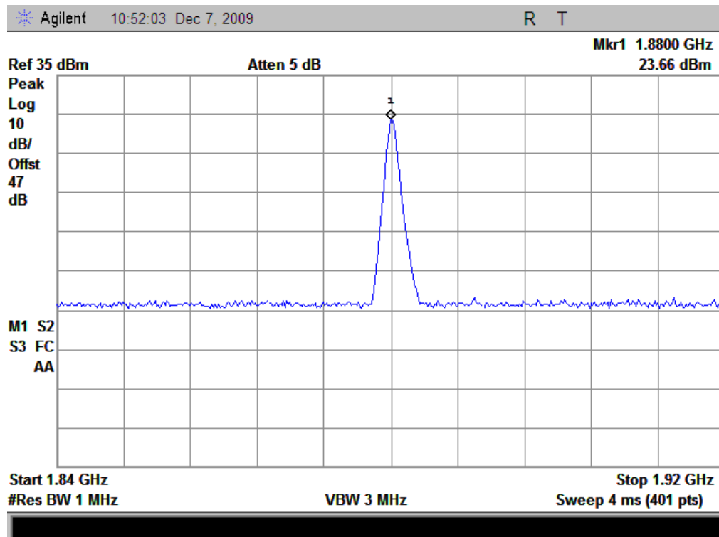
(Plot D: GSM 1900MHz Channel = 661)
