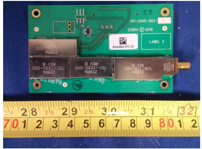
EUT – PCBA3 Top Side
