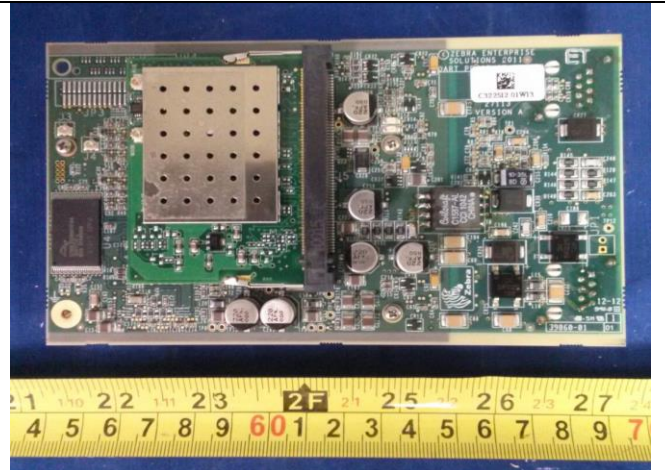
EUT - PCBA1 Top Side
