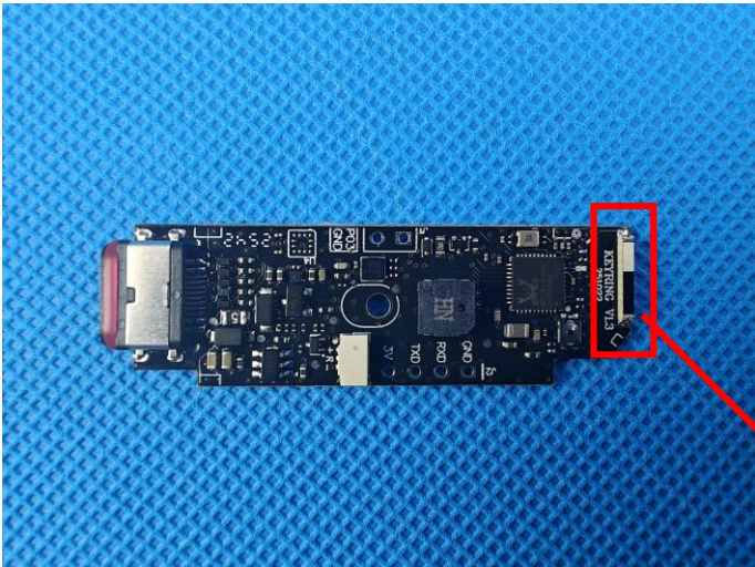
BLE ANT
