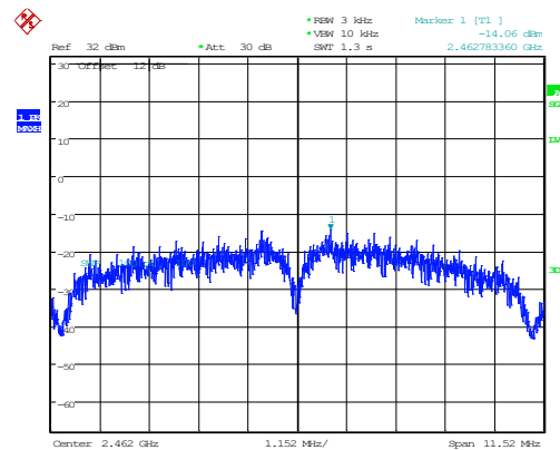
802.11b_2462MHz_Chain 1 -14.06dBm/3kHz
