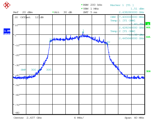
802.11n20_2437MHz_Chain 0 17.400MHz
