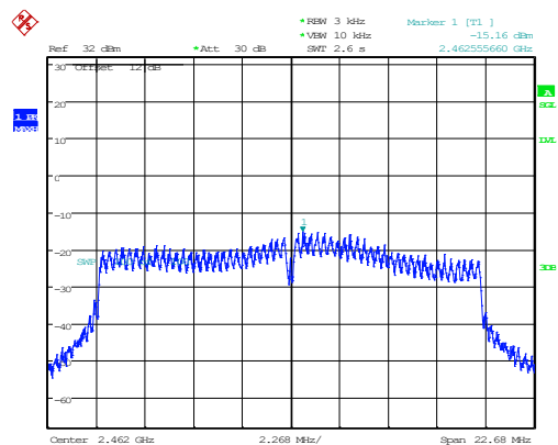
802.11n20_2462MHz_Chain 0 -15.16dBm/3kHz
