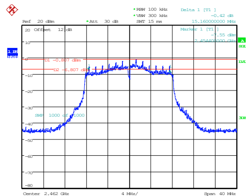
802.11g_2462MHz_Chain 1 15.160MHz
