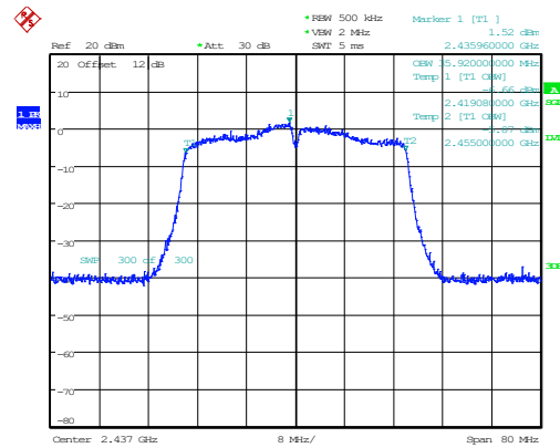
802.11n40_2437MHz_Chain 1 35.920MHz
