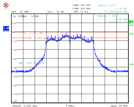
802.11g_2462MHz_Chain 0 15.160MHz
