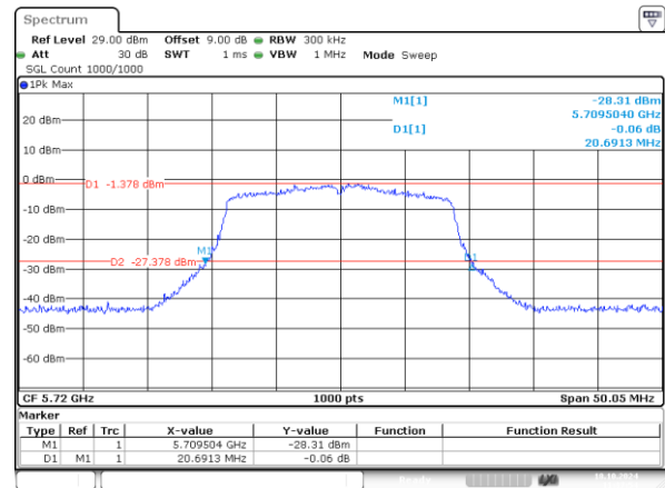
802.11n20_5720MHz_Chain 1 20.691MHz
