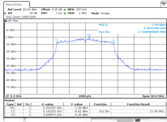
802.11n20_5200MHz_Chain 1 17.450MHz
