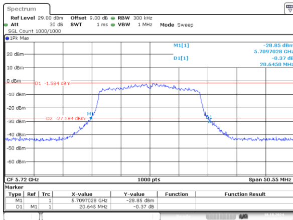
802.11n20_5720MHz_Chain 0 20.645MHz
