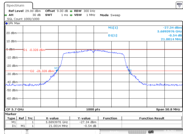
802.11n20_5700MHz_Chain 1 21.001MHz
