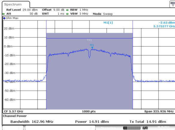
802.11ac160_5570MHz_Chain 0
