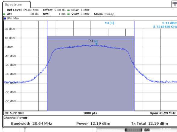
802.11n20_5720MHz_Chain 0
