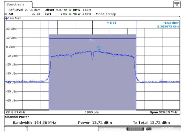
802.11ac160_5570MHz_Chain 1
