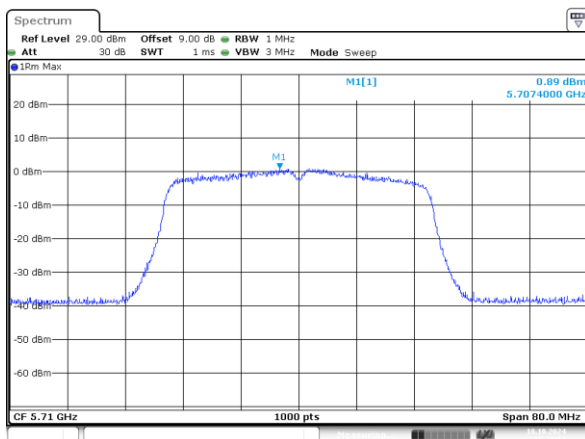
802.11n40_5710MHz_Chain 0
