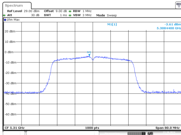
802.11n40_5310MHz_Chain 0
