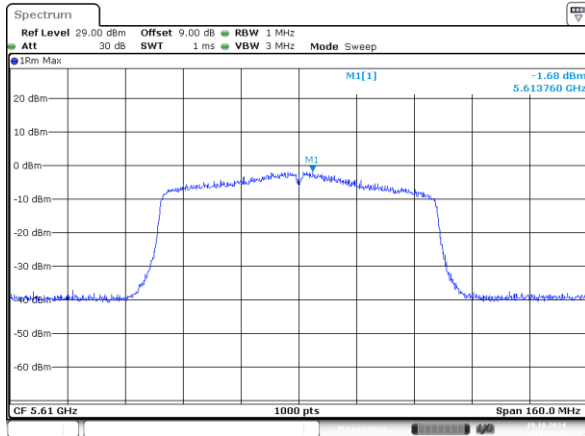
802.11ac80_5610MHz_Chain 0
