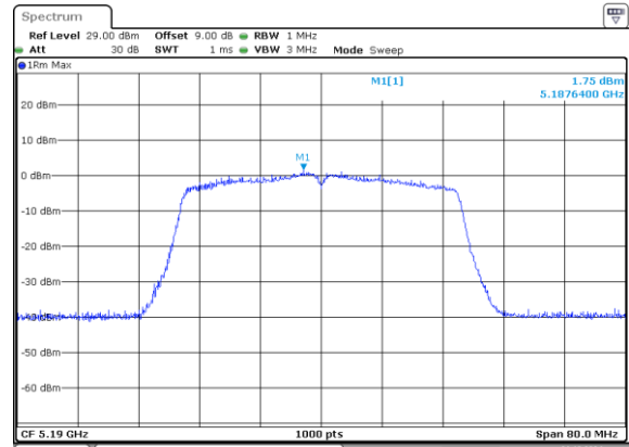
802.11n40_5190MHz_Chain 1
