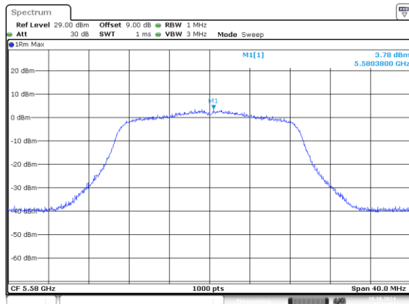
802.11n20_5580MHz_Chain 0
