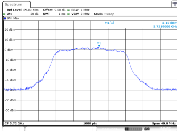
802.11a_5720MHz_Chain 0
