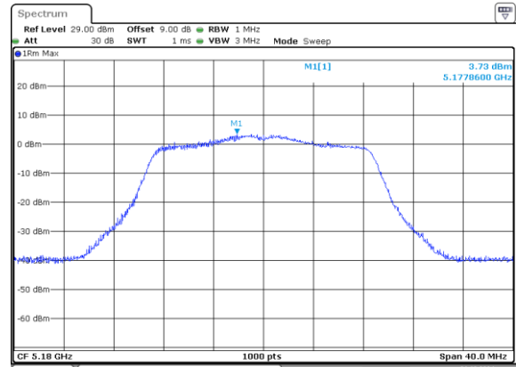
802.11n20_5180MHz_Chain 1
