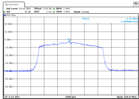
802.11ac80_5210MHz_Chain 1
