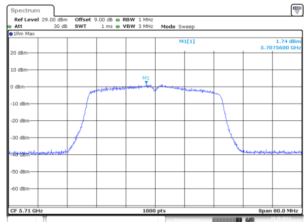
802.11n40_5710MHz_Chain 1
