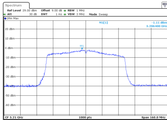
802.11ac80_5210MHz_Chain 0
