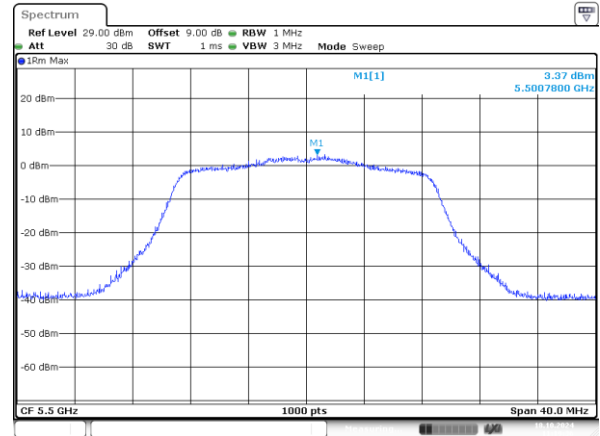
802.11n20_5500MHz_Chain 1
