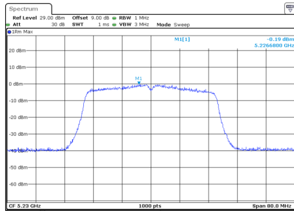
802.11n40_5230MHz_Chain 0
