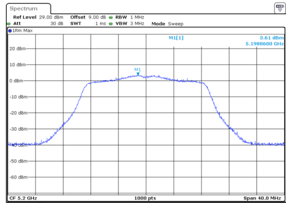
802.11n20_5200MHz_Chain 1
