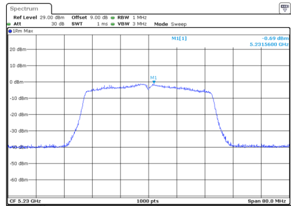
802.11n40_5230MHz_Chain 1
