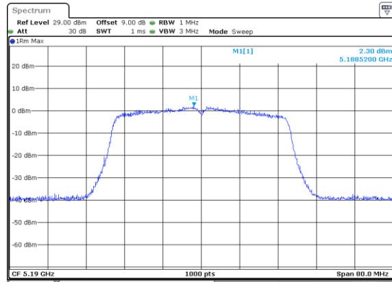
802.11n40_5190MHz_Chain 0
