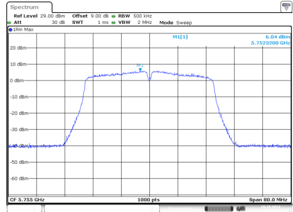
802.11n40_5755MHz_Chain 1
