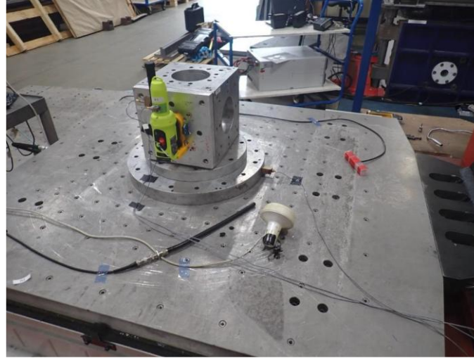
Y Axis Test Setup
