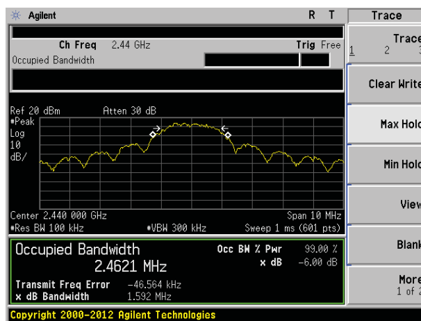
2440MHz
