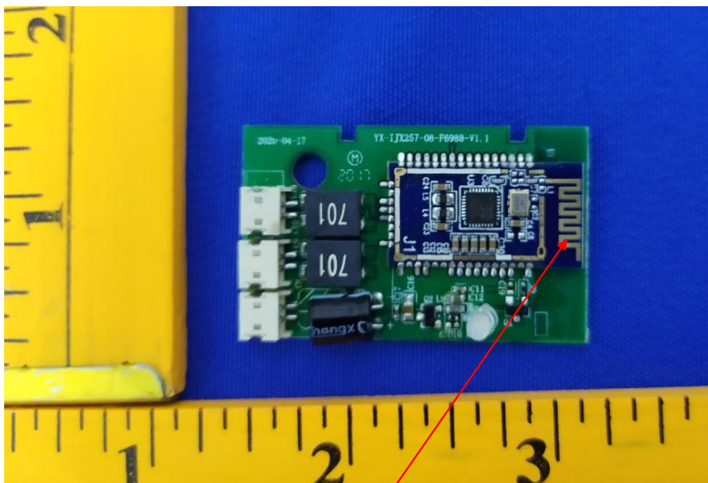
Antenna
