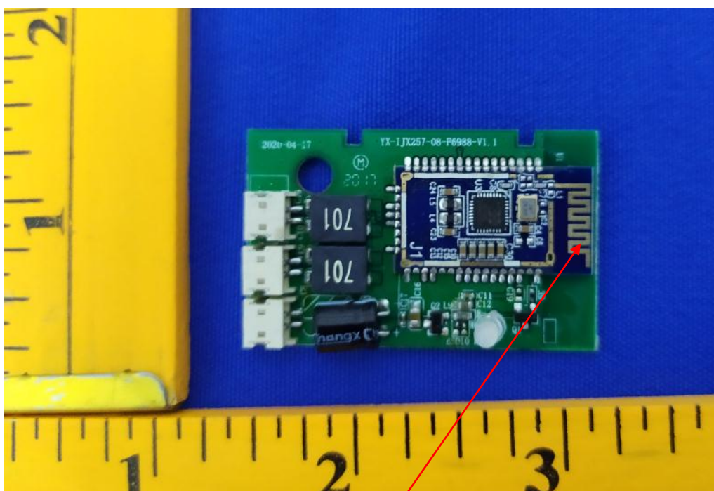
Antenna
