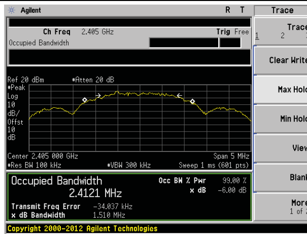
2405MHz
