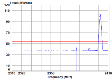
BLE_TX_CH_00_Horizontal-AVG
