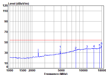
BLE_TX_CH_19_Horizontal-Avg
