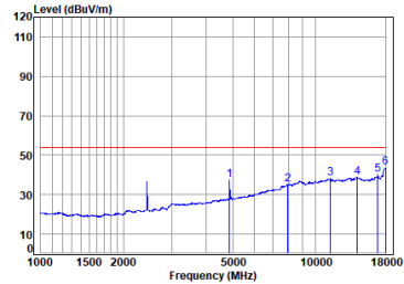
BLE_TX_CH_19_Horizontal-Avg
