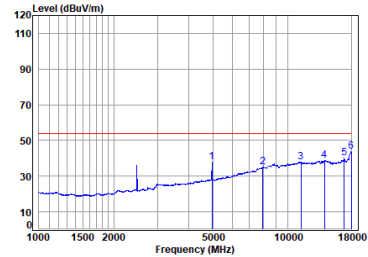
BLE_TX_CH_39_Horizontal-Avg
