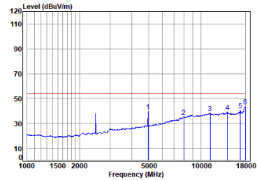
BLE_TX_CH_39_Vertical-Avg
