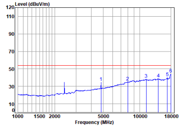
BLE_TX_CH_00_Horizontal-Avg
