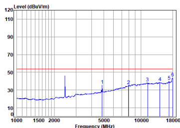
BLE_TX_CH_19_Vertical-Avg
