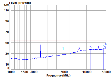
BLE_TX_CH_19_Vertical-Avg
