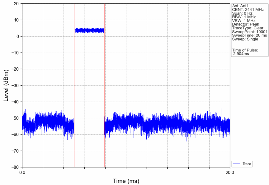
8DPSK_3DH5_HOPP_Ant1_NTNV
