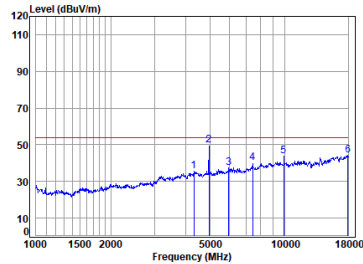
01 BLE_1M_TX_CH_39_Horizontal-Avg
