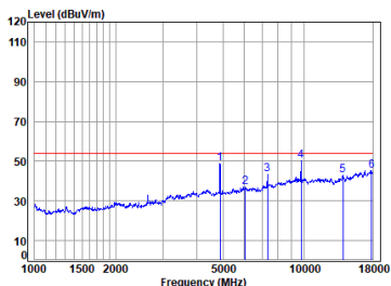
01 BLE_1M_TX_CH_19_Horizontal-Avg
