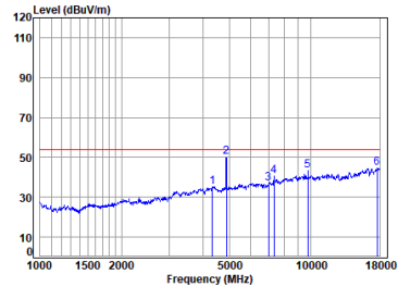
01 BLE_1M_TX_CH_19_Horizontal-Avg
