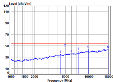
01 BLE_1M_TX_CH_39_Vertical-Avg
