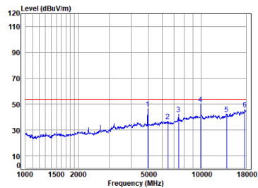
01 BLE_1M_TX_CH_39_Vertical-Avg
