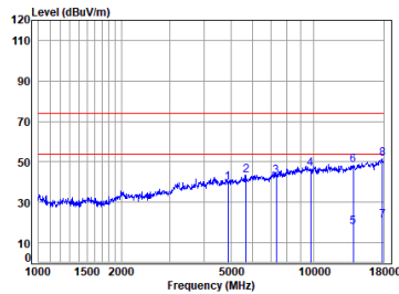
BT_DH5_TX_CH_39_Horizontal
