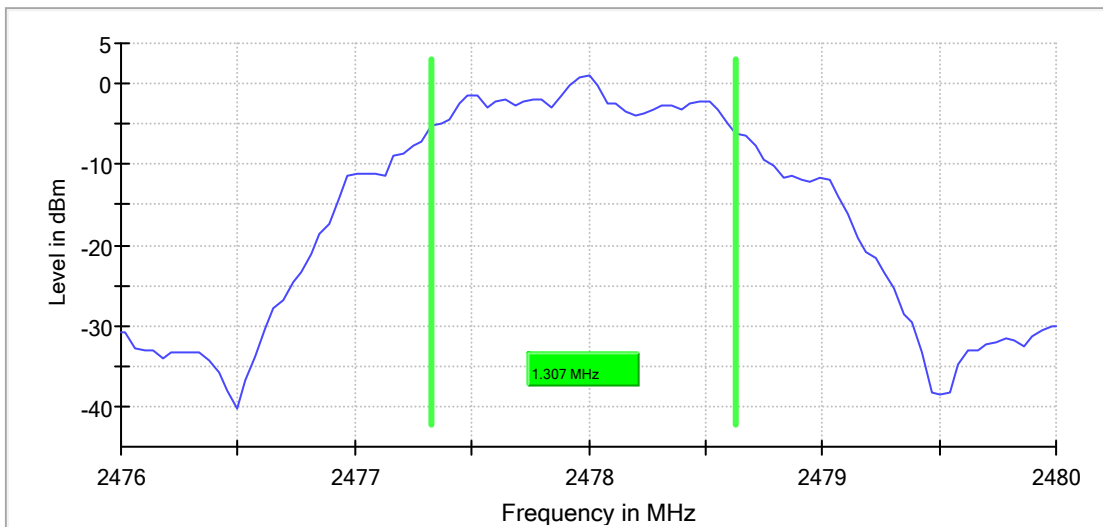
BLE_2M_Ant1_2478
