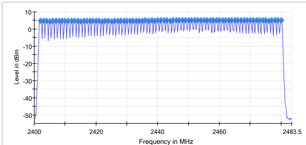
3DH5_Ant1_Hop
