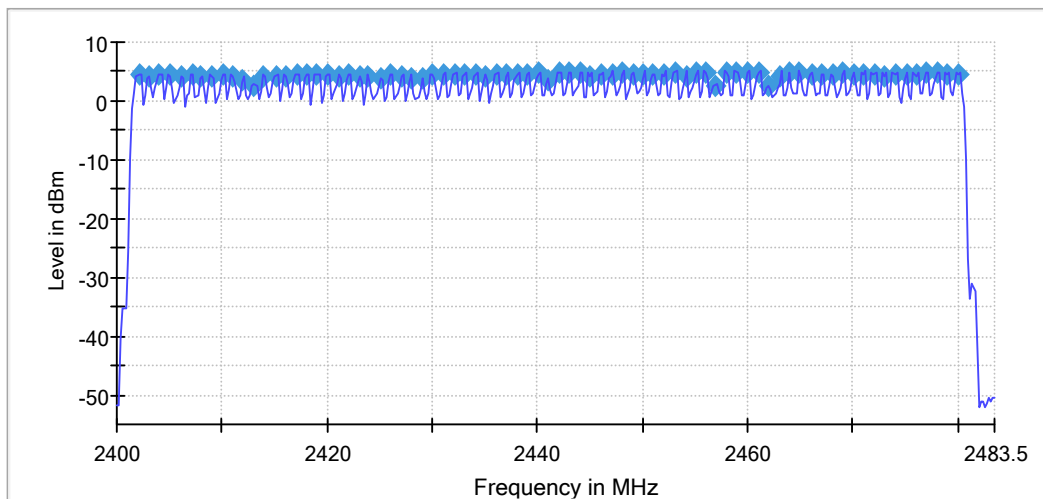
3DH5_Ant1_Hop
